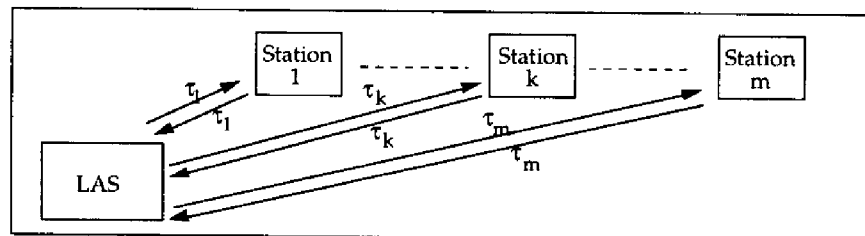
Figure 5.1: Le mécanisme du jeton EA
