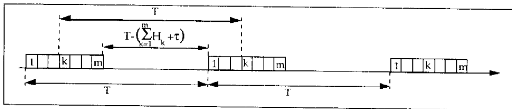
Figure 5.2: Cas 1 de la séquence de génération de jetons EA
