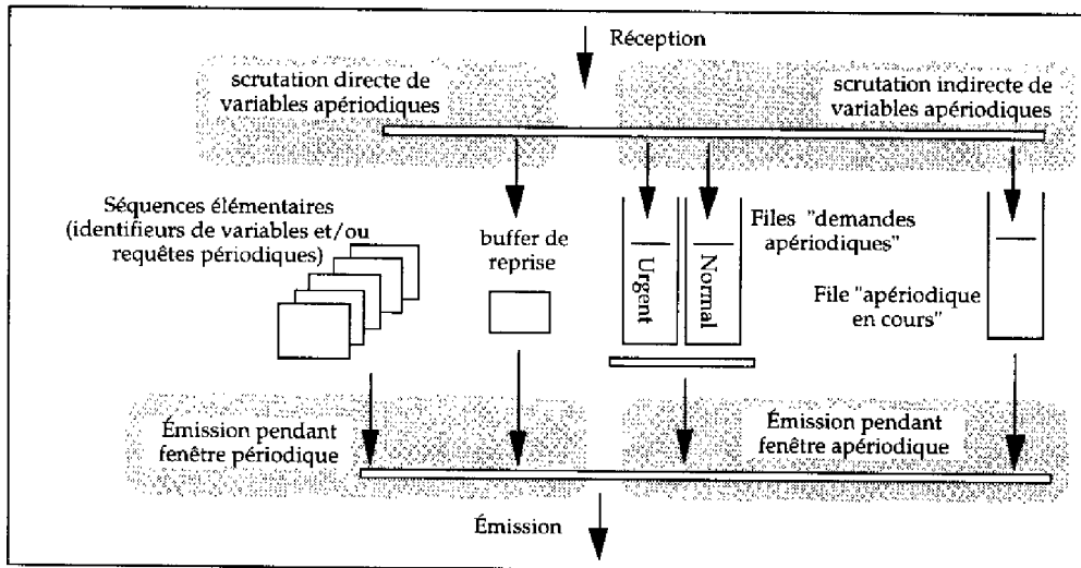
Figure 3.6: Les mécanismes de l'arbitrage d'accès dans FIP
