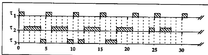
Figure 2.2: Exemple d'ordonnancement ED
