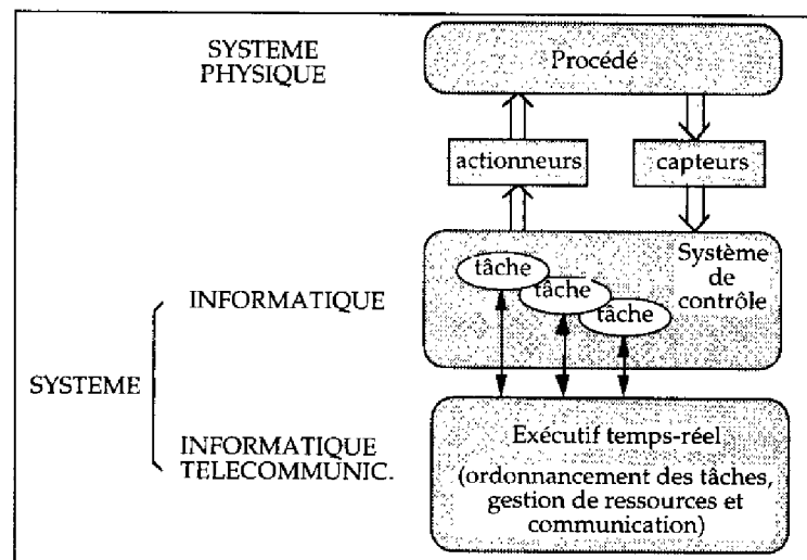
Figure 1.1: Système temps-réel
