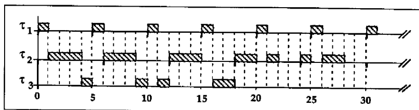
Figure 2.1: Exemple d'ordonnancement RM
