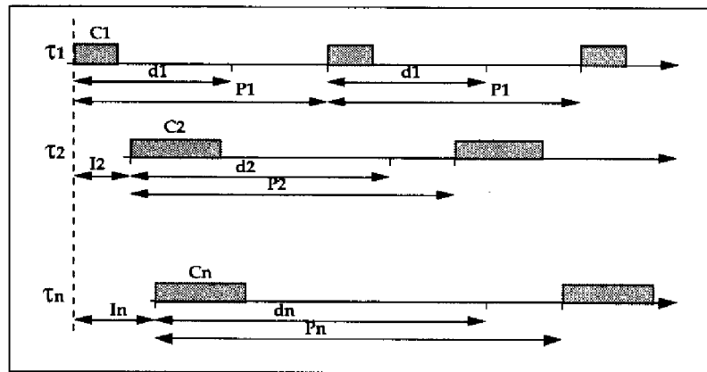
Figure 1.2: Modèle des tâches
