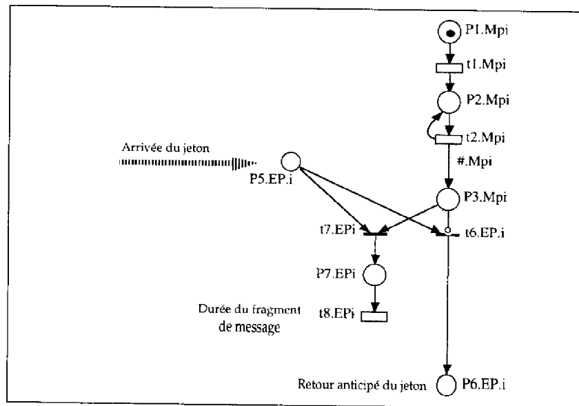
Figure 5.6: Service de flux de messages périodique Mp_i
