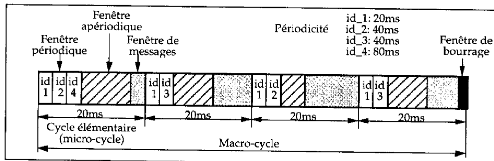
Figure 3.5: Table de scrutation dans FIP
