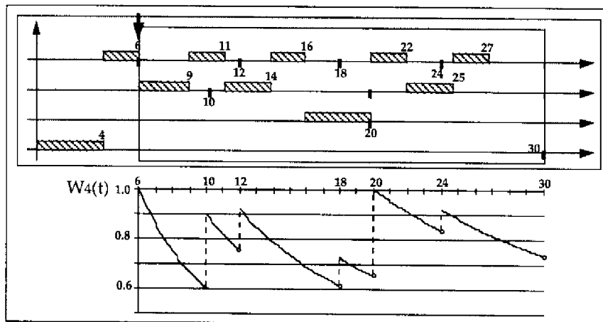
Figure 2.6: Séquence temporelle et demande normalisée W_4(t)
