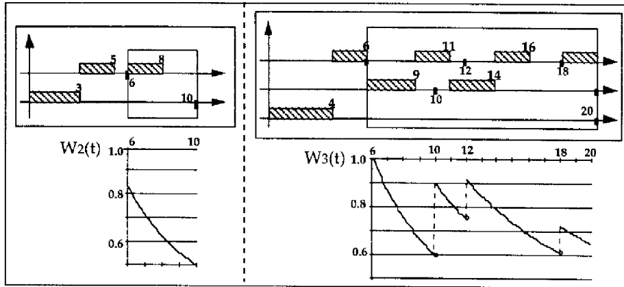
Figure 2.5: Séquences temporelles et demande normalisée W_2(t) et W_3(t)
