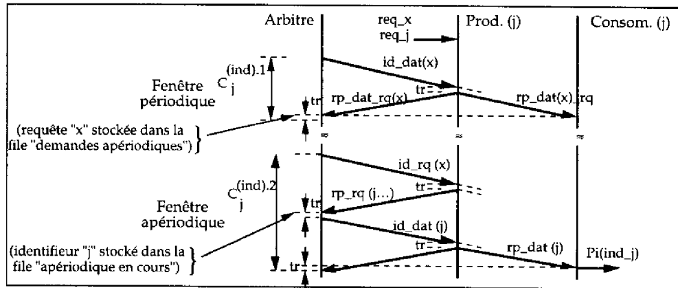
Figure 3.9: Scrutation indirecte de variables aperiodiques
