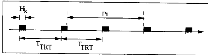
Figure 4.5: Évaluation de v_i dans la station k
