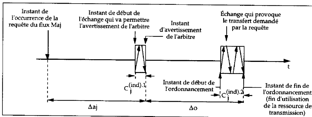
Figure 4.4: Retards d'ordonnement et d'avertissement dans la scrutation indirecte d'une variable apériodique
