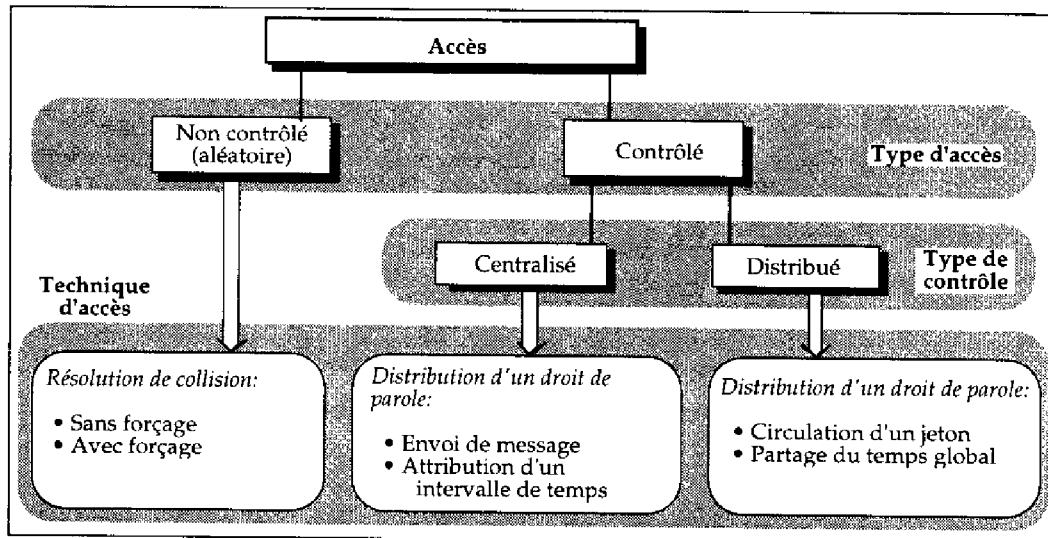
Figure 3.2: Les techniques d'accès
