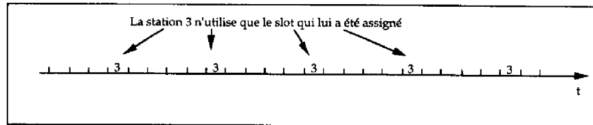
Figure 3.13: Protocole TTP
