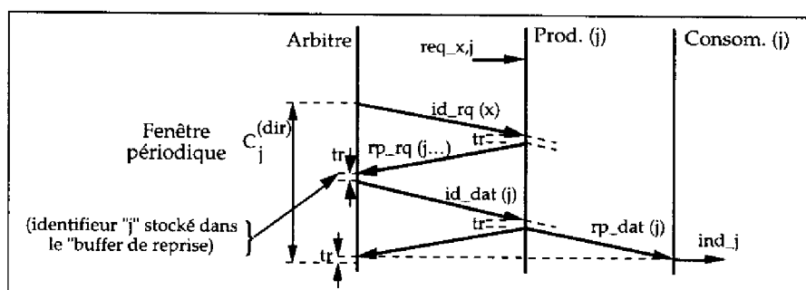
Figure 3.8: Scrutation directe de variables apériodiques
