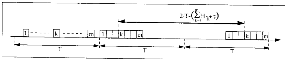
Figure 5.3: Cas 2 de la séquence de génération de jetons EA
