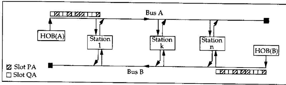
Figure 3.10: Le réseau DQDB
