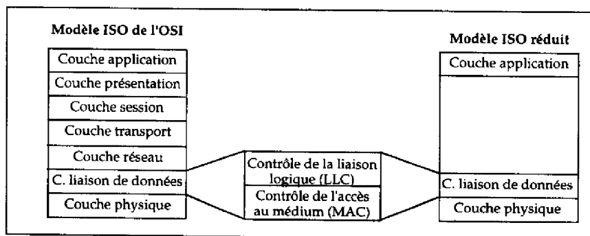
Figure 1.3: Le modèle de référence ISO de l'OSI
