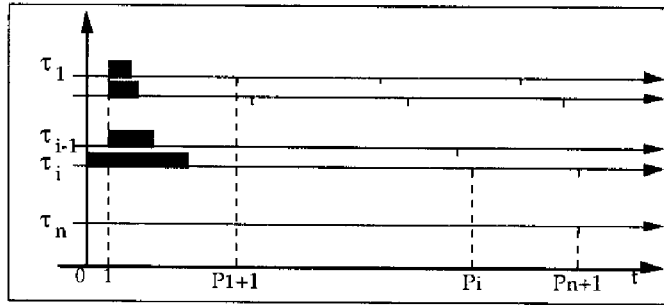
Figure 2.3: Pire cas de déphasage (tâche \tau_i )
