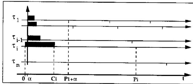
Figure 2.4: Pire cas de déphasage
