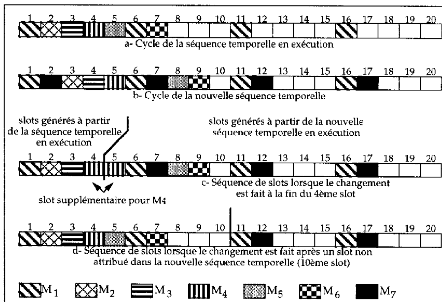
Figure 4.2: Le changement de la séquence temporelle lorsqu'un flux de messages est ajouté
