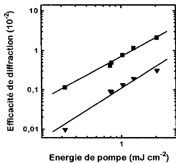
fig. 3 : Efficacité de diffraction fonction de l'énergie de pompe sur CZT. Configuration non-dégénérée \lambda_s = 865 \text{ nm} (carrés) ou 885 \text{ nm} (triangles), \lambda_p = 811 \text{ nm} . Le pas du réseau est \Lambda = 20 \mu\text{m} . Les droites représentent la fonction énergie à la puissance 1,64 et 1,77.
