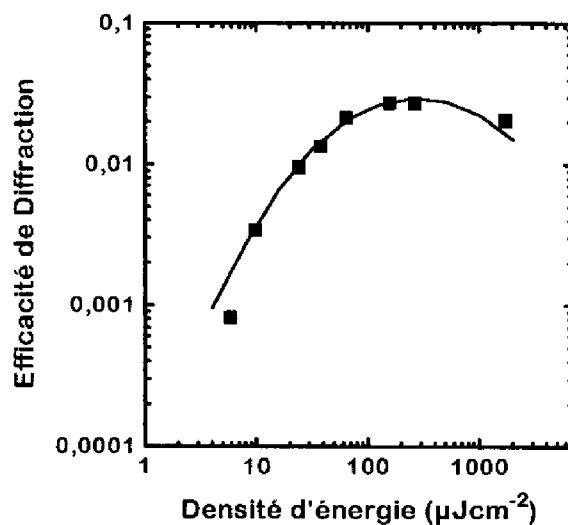
fig. 4 : Efficacité de diffraction en fonction de l'énergie des pompes à énergie de sonde constante. Configuration de Raman-Nath, dégénérée avec \lambda=1,42\mu\text{m} . Carrés : Points expérimentaux ; En trait plein, courbe issue de la modélisation ci-dessous.
