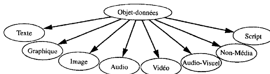
Figure 4.2 Classes Données 1
