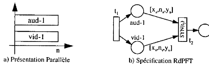
Figure 2.26 Dérive temporelle
