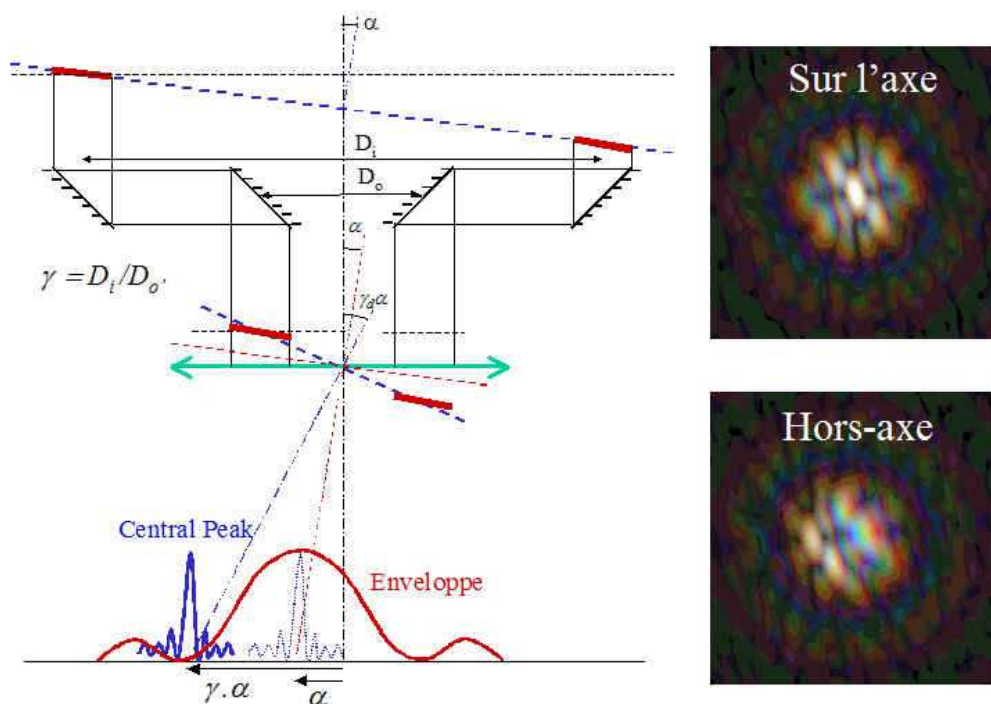
Fig. 2.3 – Propriétés d'imagerie dans le cas d'une étoile ponctuelle hors-axe.
