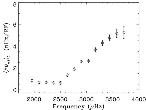
Fig. 6.5 – Sensibilité des modes à l'activité magnétique en fonction de leur fréquence : cette figure illustre pour chaque mode sa variation observée en fréquence normalisée par le flux radio (d'après García et al., 2004b ).
