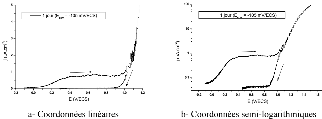
Figure 51 : courbe de polarisation anodique acquise selon le protocole « quasi in situ » sur un échantillon d'acier 304L immergé depuis 1 jour dans la Seine sur le site de Choisy-le-Roi (vitesse de balayage : 0,15 mV/s, échelles linéaire et semi-logarithmique)
