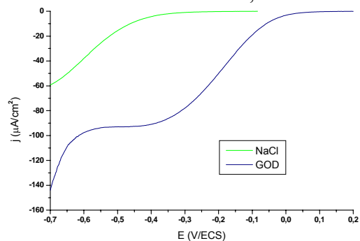
d- Acier 316L : zoom entre -0,7 et 0 V/ECS
