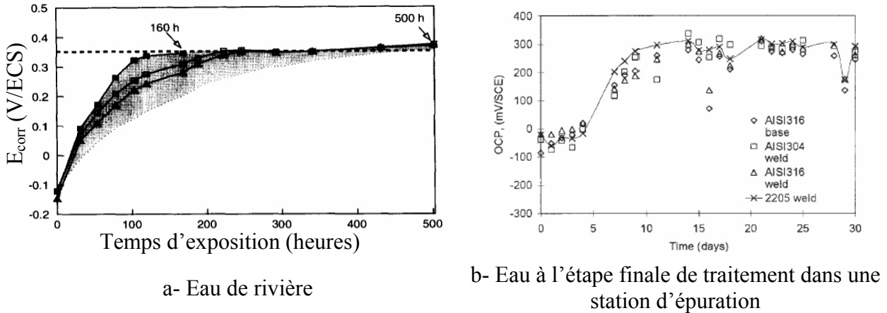
Figure 2 : Evolution du potentiel de corrosion libre a- d'échantillons d'acier 316L immergés en eau de rivière [25] b- d'échantillons d'aciers 304 et 316 immergés dans une eau usée contenant 0,515 g/L de Cl - [34]
