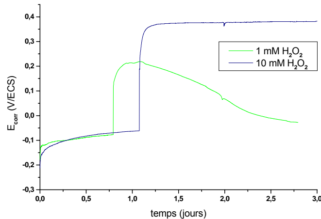
Figure 112 : évolution du potentiel de corrosion libre de 2 échantillons d'acier 254SMO immergés en eau de rivière artificielle, avec introduction de différentes concentrations de H 2 O 2 à t = 24h environ
