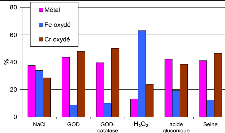
Figure 100 : pourcentage en métal, fer oxydé et chrome oxydé des échantillons d'acier 304L en fonction de la solution d'immersion
