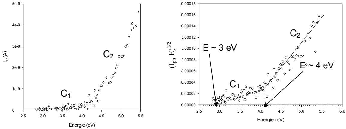
b- Transformée linéaire (I_{ph} \cdot E)^{1/2} = f(E)
