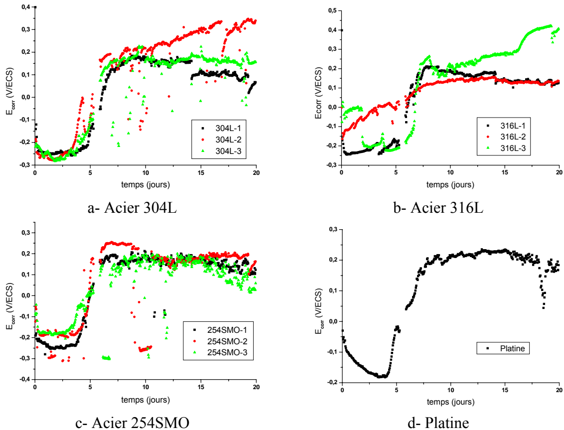
Figure 46 : suivi du potentiel de corrosion libre d'échantillons métalliques immergés le 20 Septembre dans la Seine sur le site de Flins (T=14°C)
