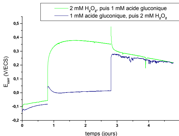
Figure 116 : évolution du potentiel de corrosion libre de 2 échantillons d'acier 316L immergés en eau de rivière artificielle, avec introduction successive de 2 mM de H 2 O 2 et de 1 mM d'acide gluconique, dans les deux ordres possibles
