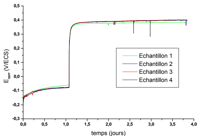
Figure 110 : évolution du potentiel de corrosion libre de 4 échantillons d'acier 254SMO immergés en eau de rivière artificielle, avec introduction de 10 mmol/L de H 2 O 2 à t = 24h environ
