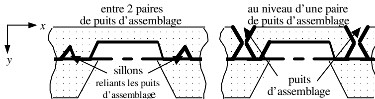
Figure VI.4 : Vue de coupe au niveau d'une paire de puits d'assemblage
