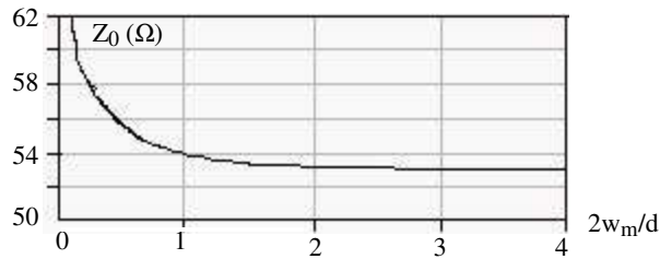
Figure IV.8 : Impédance en fonction de la largeur de demi-plan de masse w_m sur silicium massif pour une largeur de ruban w = 70 \mu\text{m} et une largeur de fente s = 50 \mu\text{m}
