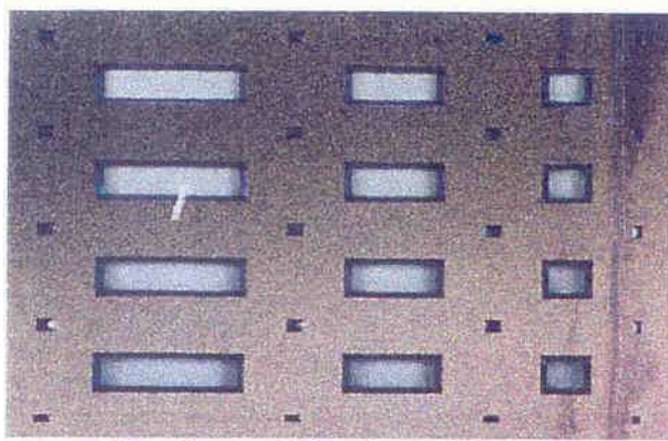
Figure II.22 : Membranes 2x2, 2x4, 2x6 mm 2 sur un substrat de silicium
