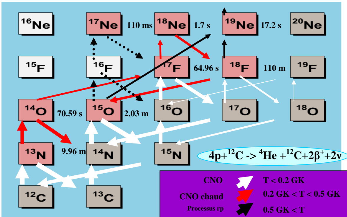
Figure III-29 Le cycle CNO et CNO-chaud. Avec les flèches pointillées sont présentées les nouvelles réactions proposées par ce travail comme réactions dans le cadre de cycle CNO-chaud. Les deux réactions sont ^{15}\text{O}(p,\gamma)(\beta^+)^{16}\text{O} et ^{15}\text{O}(p,\gamma)(p,\gamma)^{17}\text{Ne} . Les deux réactions sont en compétition et si les valeurs des facteurs spectroscopiques pour les niveaux de ^{17}\text{Ne} considérés sont correctes, la réaction (p,\gamma)(p,\gamma) est la réaction dominante. Un nouveau noyau peut être produit dans le cadre de ces réactions – le ^{17}\text{Ne} .
