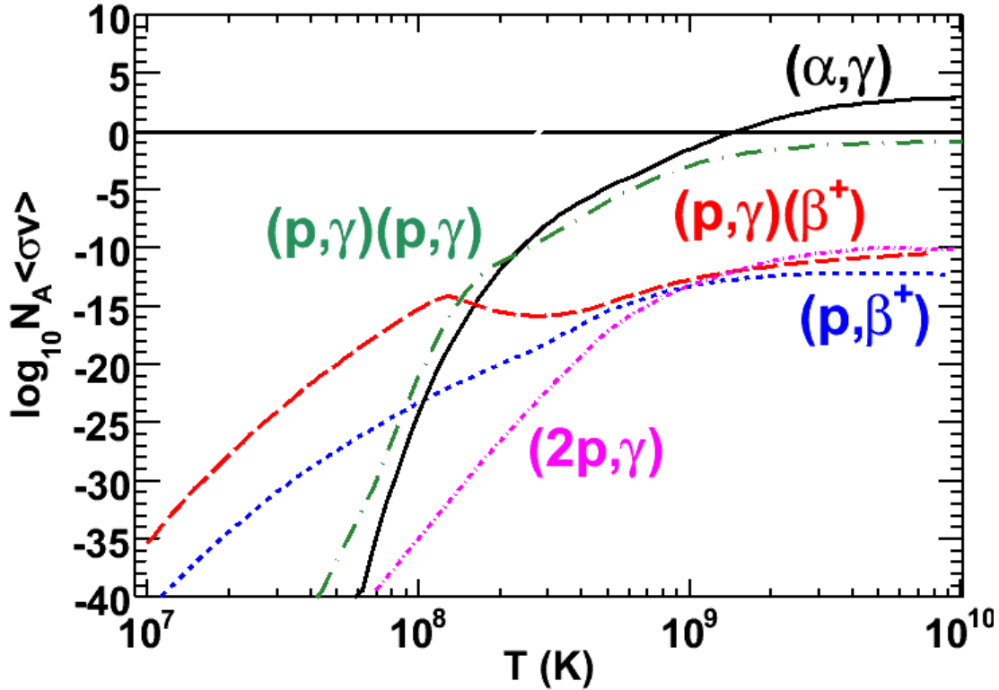
Figure III-27 Le calcul de taux ( fait avec le code numérique PN1oNR) pour la réaction ^{15}\text{O}(p,\gamma)(p,\gamma)^{17}\text{Ne} et la comparaison avec les autres processus possibles à partir d' ^{15}\text{O} - ^{15}\text{O}(2p,\gamma)^{17}\text{Ne} , ^{15}\text{O}(\alpha,\gamma)^{19}\text{Ne} , ^{15}\text{O}(p,\beta^+)^{16}\text{O} et ^{15}\text{O}(p,\gamma)(\beta^+)^{16}\text{O} . Les deux taux de réactions, (p,\gamma)(\beta^+) et (p,\gamma)(p,\gamma) , sont limités par la probabilité de capture radiative ^{15}\text{O}(p,\gamma)^{16}\text{F}^{\text{gs}} . Pour la réaction (p,\gamma)(p,\gamma) , la densité du milieu astrophysique utilisé pour le calcul est de 10^6 \text{ g/cm}^3 .
