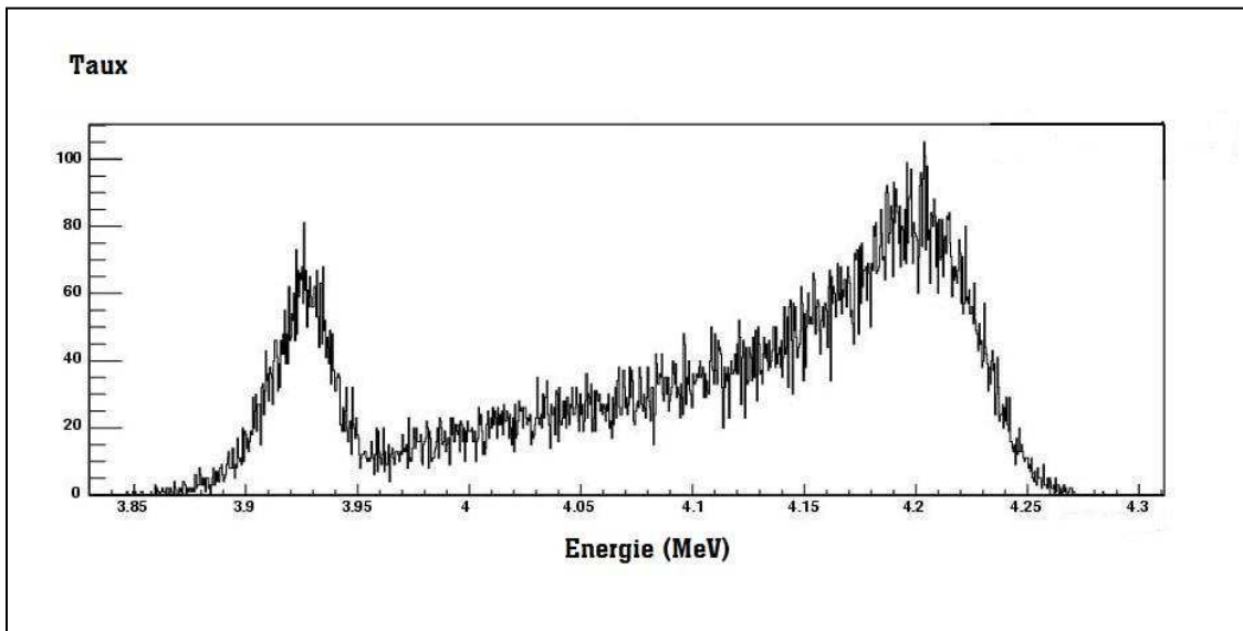
Figure II-19 Fonction d'excitation attendue pour la réaction {}^4\text{He}({}^{15}\text{N},\alpha){}^{15}\text{N} . Le calcul a été fait avec la théorie de la matrice R à partir des états connus du noyau composé pour cette réaction, le {}^{19}\text{F} .
