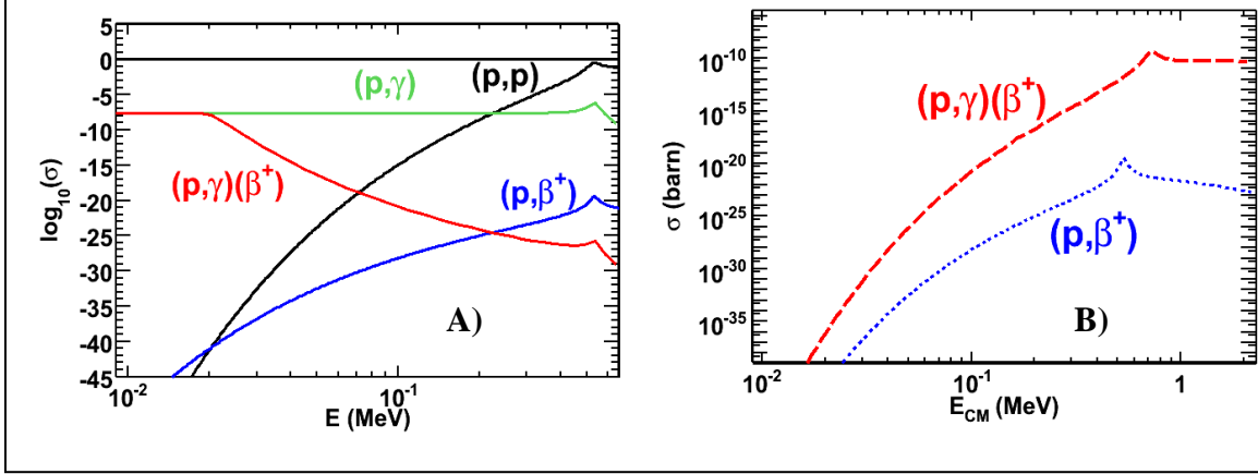
Figure III-22 Section efficace de la réaction ^{15}\text{O}(p,\gamma)(\beta^+)^{16}\text{O} , et comparaison avec la section efficace de la réaction ^{15}\text{O}(p,\beta^+) . Dans la figure A), nous avons représenté différents termes de l'équation III-20, et la comparaison avec les réactions ^{15}\text{O}(p,p)^{15}\text{O} et ^{15}\text{O}(p,\beta^+) . La courbe (p, \gamma ) représente la section efficace de la réaction ^{15}\text{O}(p,\gamma)^{16}\text{F}^{\text{gs}} de peupler l'état fondamental de ^{16}\text{F} à une énergie relative E entre le proton et ^{15}\text{O} (calculé pour une énergie dans le système de centre de masse égale à 0.729 MeV). La courbe (p, \gamma )( \beta^+ ) représente la section efficace de la réaction ^{15}\text{O}(p,\gamma)(\beta^+)^{16}\text{O} peuplant l'état fondamental de ^{16}\text{F} (peuplé par la transition gamma) à une énergie finale relative E entre le proton et l' ^{15}\text{O} (la courbe est calculée pour une énergie incidente proton égale à 0.729 MeV). Dans la figure B, nous avons représenté la dépendance avec l'énergie dans le système de centre de masse de la section efficace de réaction (p, \gamma )( \beta^+ ) et la comparaison avec la section efficace de réaction (p, \beta^+ ) calculé auparavant.
