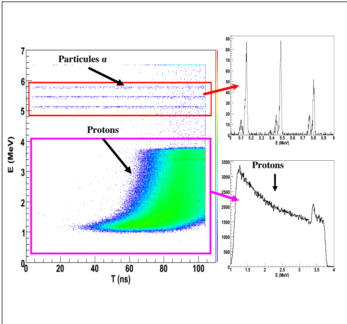
Figure III-5 A gauche : spectre de l'énergie des particules en fonction du temps de vol obtenu avec le détecteur silicium pour la mesure de la réaction {}^1\text{H}({}^{15}\text{N},\text{p}){}^{15}\text{N} . On observe deux composantes, des protons en provenance de la réaction (p,p) et des particules \alpha en provenance de la source trois pics alpha placée à côté du détecteur. Partie supérieure droite : spectre en énergie des particules \alpha . Partie inférieure droite : spectre énergie pour les protons en provenance de la réaction {}^1\text{H}({}^{15}\text{N},\text{p}){}^{15}\text{N} . Le pic dans ce dernier spectre est une résonance qui correspond à la formation du noyau composé {}^{16}\text{O} . La largeur à demi-hauteur pour le pic alpha de 5.48 MeV était de 14.78 keV.
