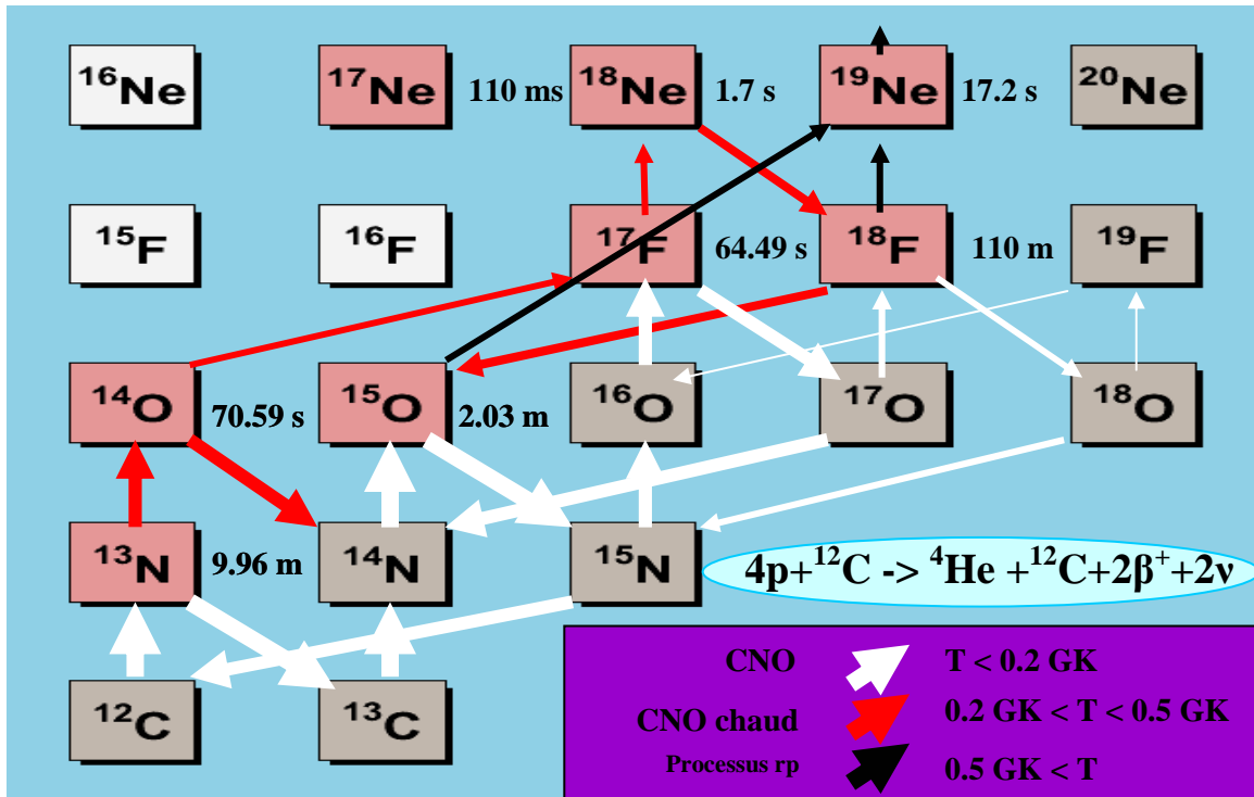
Figure I-1 Le cycle CNO et CNO-chaud. Le cycle CNO est responsable de la combustion de l'hydrogène dans les étoiles de métallicité (abondance en éléments plus lourds que {}^4\text{He} ) élevée. Le cycle CNO chaud met en scène des réactions impliquant des noyaux radioactifs de plus courte durée de vie. Les réactions qui permettent l'échappement (« break-out ») du cycle CNO sont particulièrement intéressantes pour la nucléosynthèse explosive extrême (sursauts X de type I). L'épaisseur de la flèche représente l'intensité de la réaction.
