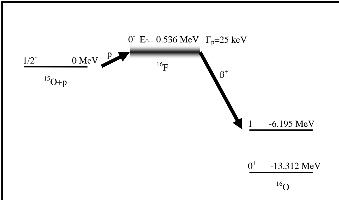
Figure III-13 Représentation schématique de la réaction ^{15}\text{O}(p, \beta^+)^{16}\text{O} . Comme l'état fondamental de ^{16}\text{F} avec spin/parité 0^- et celui d' ^{16}\text{O} est de 0^+ , la transition bêta de ^{16}\text{F} favorise certainement plutôt le premier état 1^- d' ^{16}\text{O} .
