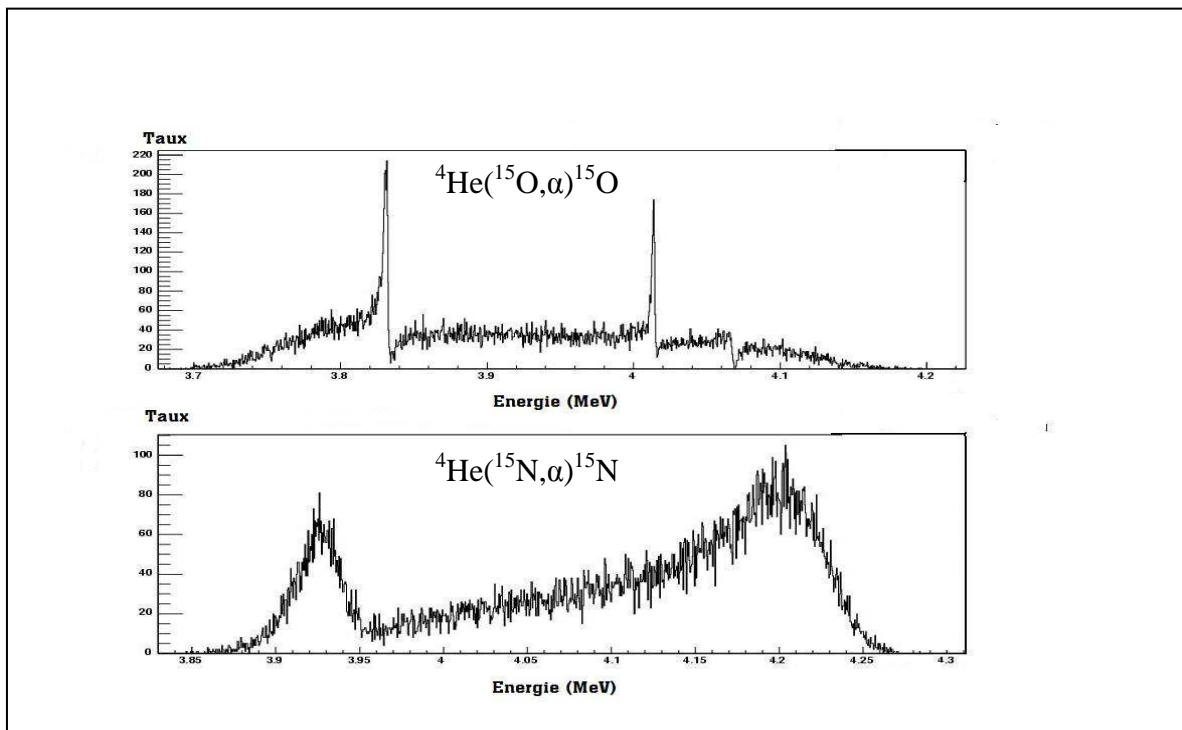
Figure II-22 Spectres simulés attendus pour les deux réactions de diffusion élastique résonante, {}^4\text{He}({}^{15}\text{N}, \alpha){}^{15}\text{N} et {}^4\text{He}({}^{15}\text{O}, \alpha){}^{15}\text{O} . Malheureusement, à cause des conditions expérimentales (contaminants probablement causé par la diffusion du faisceau sur les fenêtres de la cible), nous n'avons pas réussi à obtenir de bonnes mesures.
