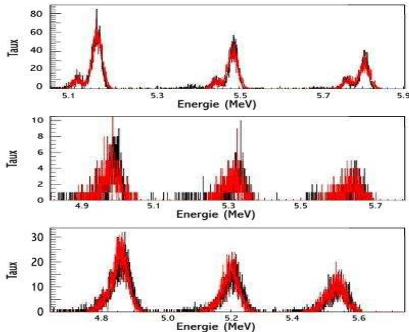
Figure II-16 Mesures et simulations de perte d'énergie et de stragglings dans la cible gazeuse. Nous avons effectué des tests avec une source radioactive pendant lesquels nous avons mesuré le stragglings en énergie produit par les feuilles de mylar et par la cible gazeuse. En noir sont présentées les mesures expérimentales, et en rouge les résultats des simulations. Dans l'image supérieure nous voyons, en noir, le spectre d'énergie de la source trois pics \alpha seule (sans cible gazeuse ni feuille de mylar), et en rouge le spectre utilisé dans la simulation. Au centre, la perte d'énergie et le stragglings produits par deux feuilles de mylar de 0.9 \mu\text{m} épaisseur sont présentés. Dans la partie inférieure, le stragglings et la perte d'énergie, mesurés après deux feuilles de mylar de 0.9 \mu\text{m} épaisseur et 310 mbar de pression d'hélium à l'intérieur de la chambre gazeuse.
