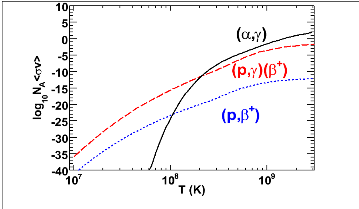
Figure III-23 Dépendance en température pour divers taux de réaction. Le taux pour le processus ^{15}\text{O}(p,\gamma)(\beta^+)^{16}\text{O} est comparé avec celui pour la réaction ^{15}\text{O}(p,\beta^+)^{16}\text{O} et avec celui de la réaction ^{15}\text{O}(\alpha,\gamma)^{19}\text{Ne} .
