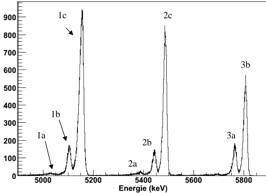
Figure II-13 Le spectre en énergie de la source trois pics alpha que nous avons utilisée. Les trois pics les plus intenses ont des énergies égales à 5156.6, 5485.6 et 5804.8 keV. La résolution du détecteur utilisé est donnée par la largeur à demi hauteur pour le pic à 5485.6 keV, cette largeur est égale à 14.5 keV
