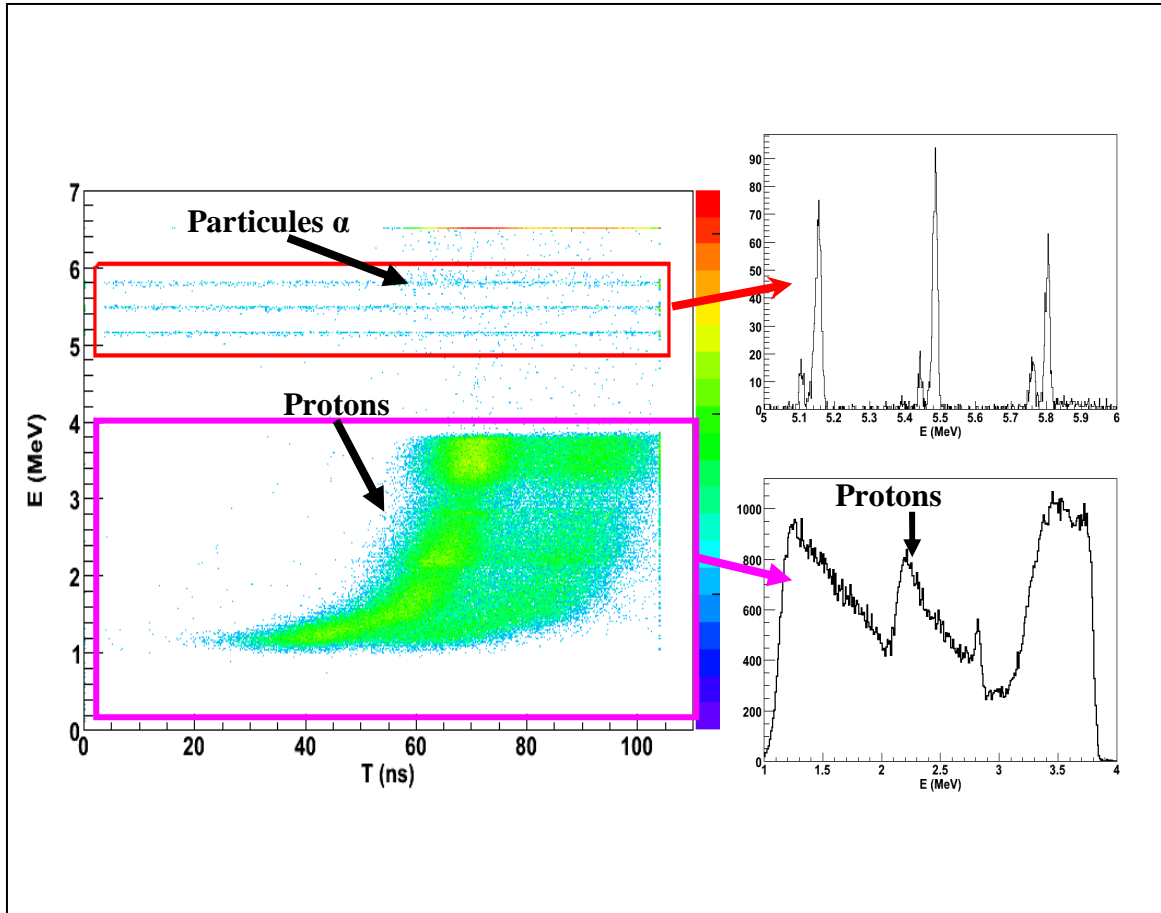
Figure III-4 A gauche : spectre de l'énergie des particules en fonction du temps de vol obtenu avec le détecteur de silicium pour la mesure de la réaction {}^1\text{H}({}^{14}\text{N},\text{p}){}^{14}\text{N} . On observe deux composantes, en bas les protons en provenance des réactions (p,p) et en haut les particules \alpha en provenance de la source trois pics alpha mise à côté du détecteur. Dans la partie supérieure droite, nous montrons le spectre en énergie des particules \alpha . Dans la partie inférieure droite, nous montrons le spectre en énergie pour les protons en provenance de la réaction {}^1\text{H}({}^{14}\text{N},\text{p}){}^{14}\text{N} . La largeur à demi-hauteur pour le pic alpha de 5.48 MeV était de 15.5 keV.
