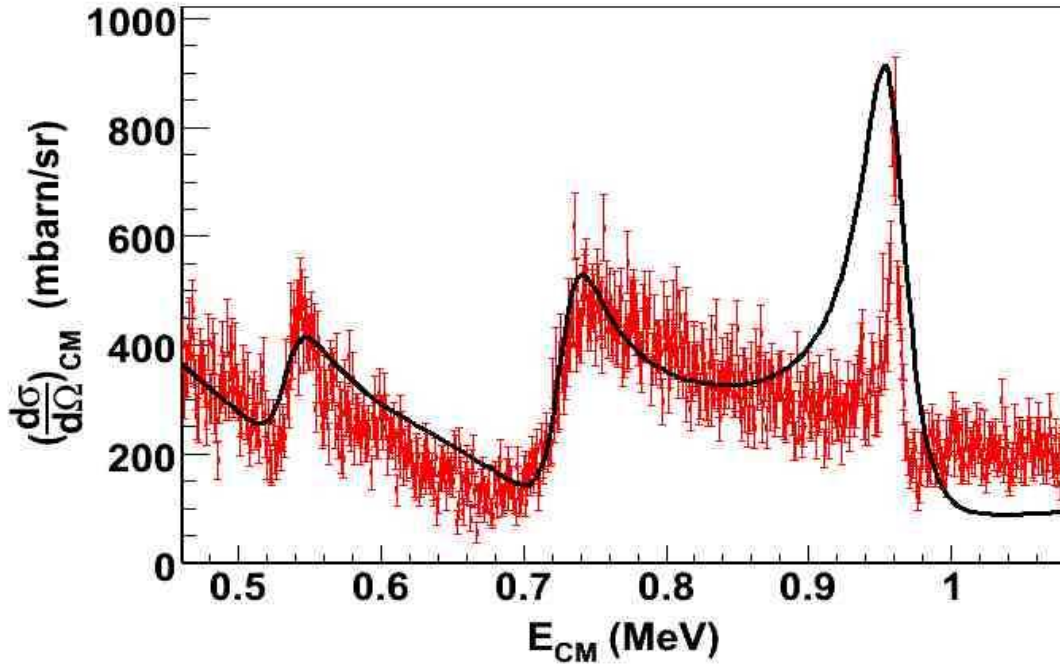
Figure III-11 Comparaison entre la fonction d'excitation mesurée (en rouge) et celle calculée (en noir) pour la réaction {}^1\text{H}({}^{15}\text{O},\text{p}){}^{15}\text{O} à partir de propriétés connues avant de notre mesure. Il est clair que nous pouvons améliorer l'accord en changeant certaines des propriétés de ces niveaux. La fonction d'excitation dans le système de centre de masse est obtenue à partir de la fonction d'excitation présentée dans la Figure III-7
