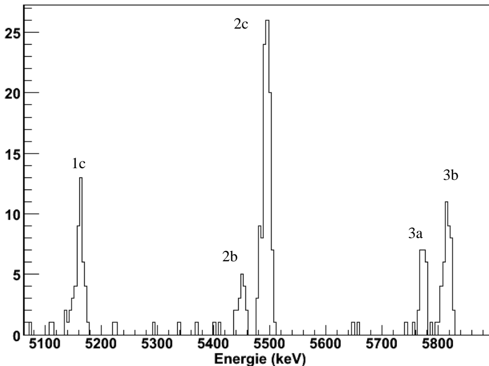
Figure II-14 Le spectre alpha mesuré au point objet du spectromètre, pour une valeur de la rigidité magnétique de 0.337 Tm. La différence en énergie entre les deux pics extrême (1c et 3b) est de 651.6 keV
