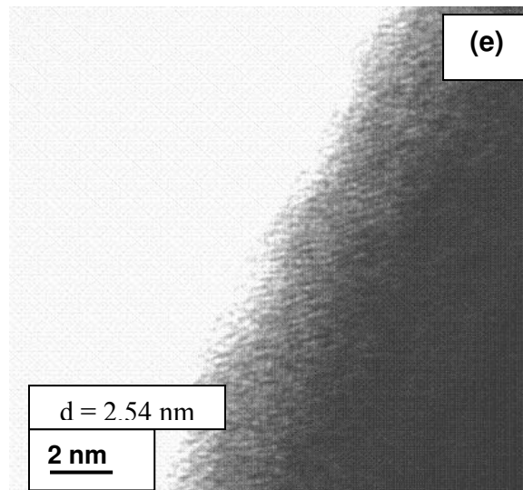
Figure 3-23 : (a) cristal noir, (b), (d), (e) frange de réseau et (c) transformée de Fourier de (b)
