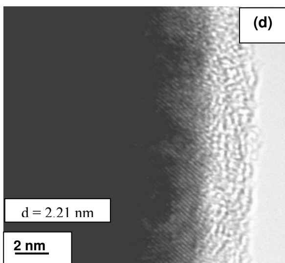
Figure 3-23 : (a) cristal noir, (b), (d), (e) frange de réseau et (c) transformée de Fourier de (b)
