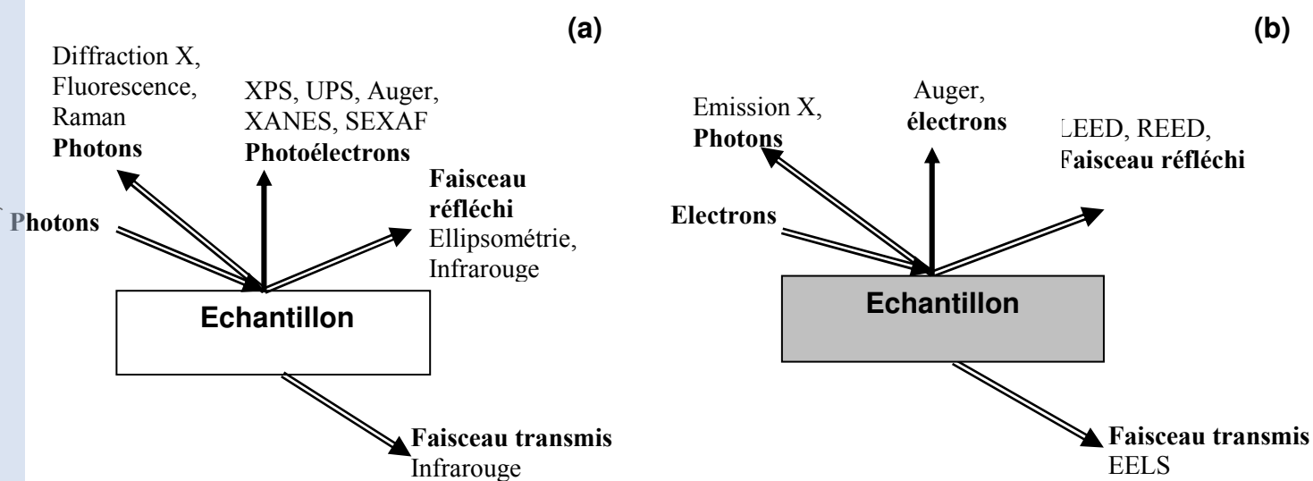
Figure 2-7 : Principaux processus d'interaction rayonnement-matière et les techniques d'analyse de surface associées:
