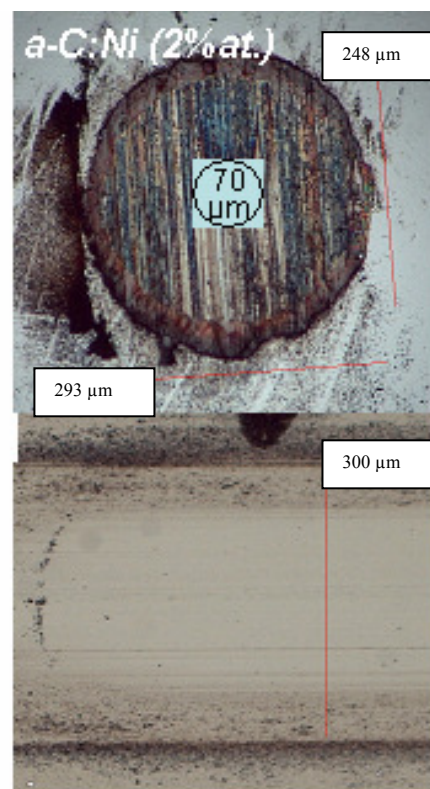
Figure 4-6 : Test tribologique « longue durée » (30000 cycles) relatif à a-C :Ni (2%at.). Images optiques de la bille en acier et du plan revêtu au terme des 30000 cycles.
