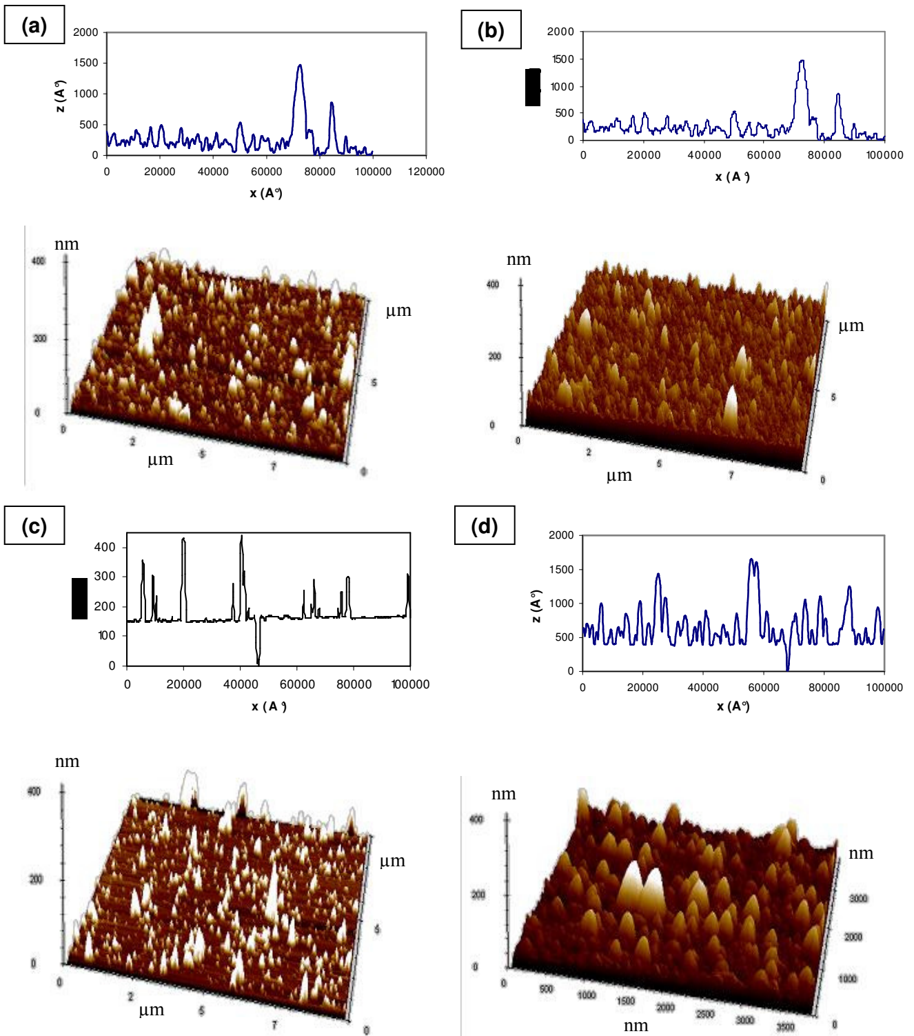
Figure 3-8 : Profils de rugosité et images 3D obtenues, par microscopie à force atomique (AFM) en « tapping mode », de films (a) a-C:Ni 2% at., (b) a-C:Ni 15% at., (c) a-C:Ta 2% at. et (d) a-C:Ta 15% at.
