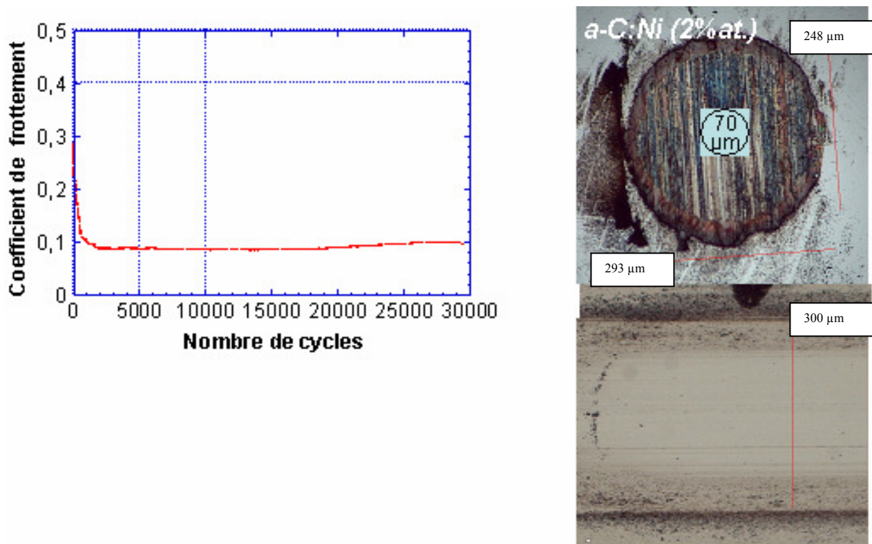
Figure 4-6 : Test tribologique « longue durée » (30000 cycles) relatif à a-C :Ni (2%at.). Images optiques de la bille en acier et du plan revêtu au terme des 30000 cycles.
