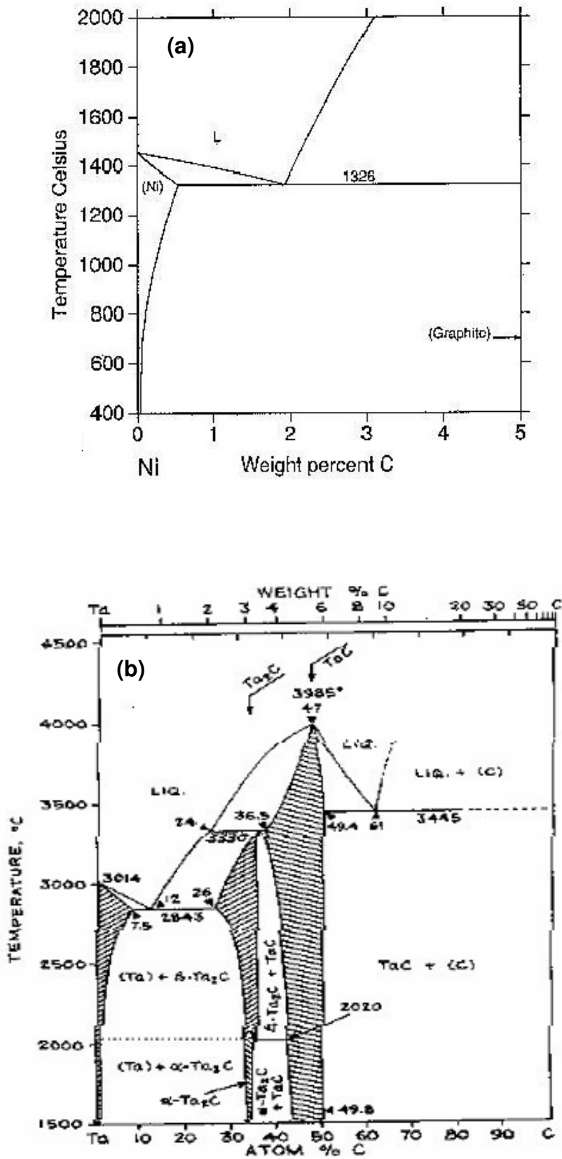
Figure 2-6 : (a) Diagramme de phase du système binaire nickel – carbone [108] (b) : Diagramme de phase du système binaire tantalé – carbone [109]
