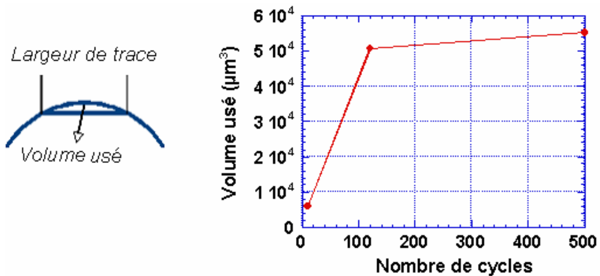
Figure 4-4 : Volume usé de la bille en acier 100C6, au terme des 3 phases du test de frottement à amplitude variable.
