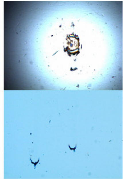
Figure 4-1 : Test de frottement d'une couche de ta-C non dopée, obtenue par PLD en mode femtoseconde. Images optiques de la trace d'usure sur la bille et sur le plan au terme de l'essai. La largeur de la trace est de l'ordre de 70 micromètres.
