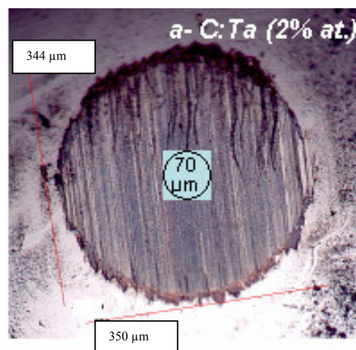
Figure 4-2 : Evolution globale du coefficient de frottement des ta-C dopés ou alliés par Ni ou Ta, en fonction du nombre de cycles : toutes les courbes sont inscrites dans l'enveloppe cernée par les deux courbes extrêmes. La courbe inscrite dans cette zone correspond à a-C:Ta (2 %at.). L'image optique montre la cicatrice d'usure correspondante, sur la bille.
