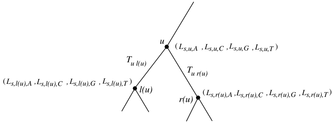
FIG. 3.2 – Association d'un vecteur de vraisemblance à un noeud interne ainsi qu'à ses deux noeuds fils
