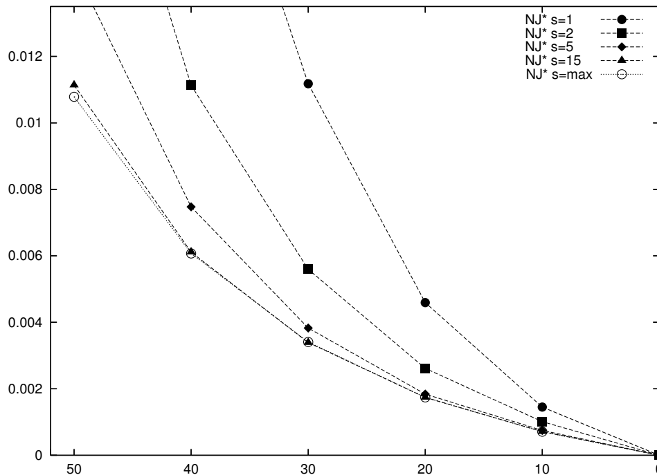
FIG. 6.3 – Performances de la combinaison de plusieurs critères d'agglomération
