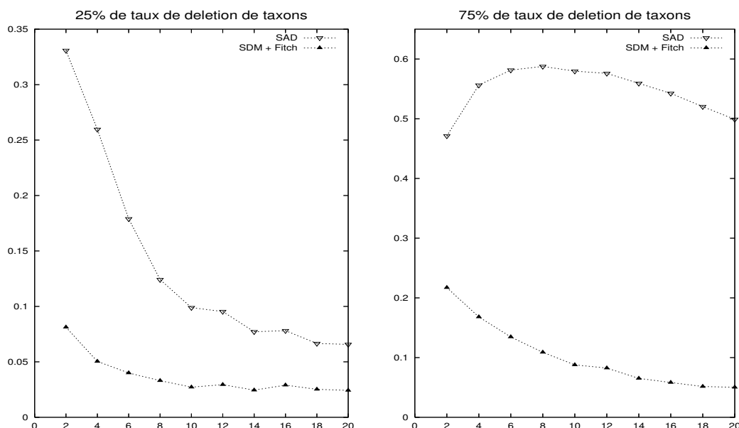
FIG. 7.1 – Performances des méthodes de distance par combinaison basse et moyenne
