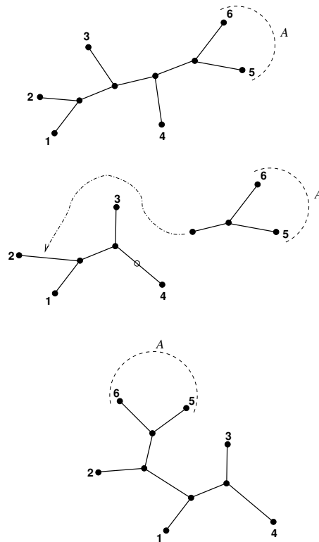
FIG. 2.7 – Réarrangement de type SPR
