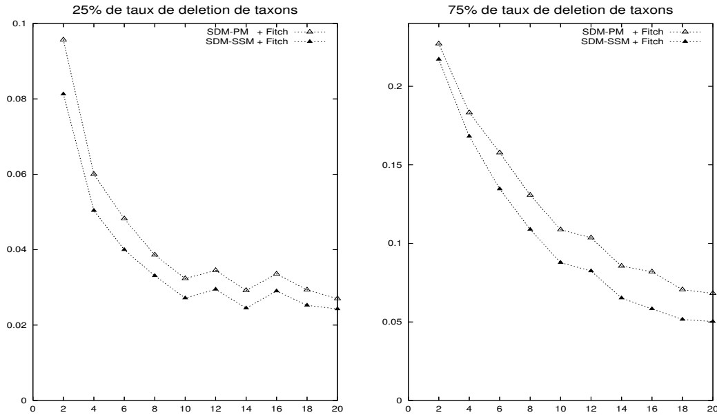
FIG. 5.3 – Observation du recouvrement topologique des scénarios de combinaison moyenne utilisant SDM
