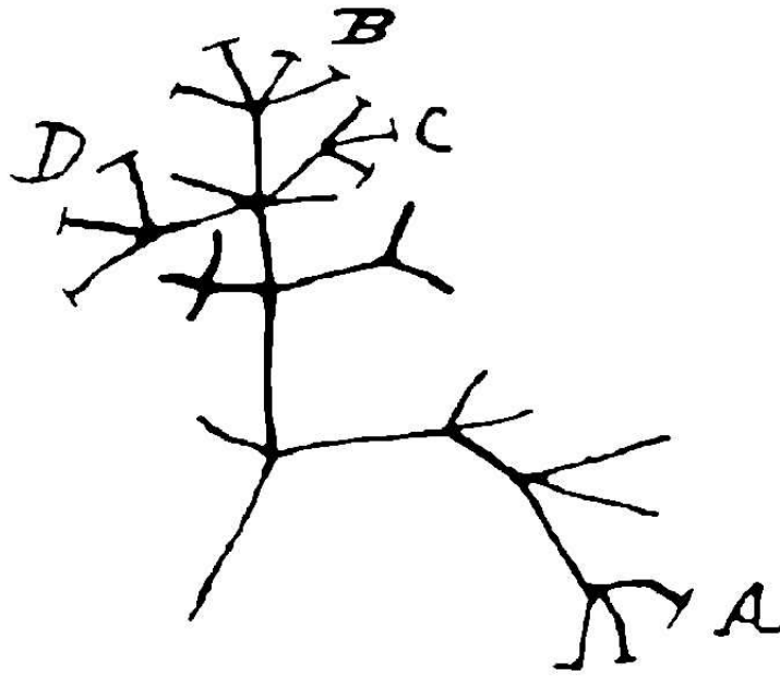
FIG. 1.2 – Modélisation de l'évolution par Darwin (1837)
