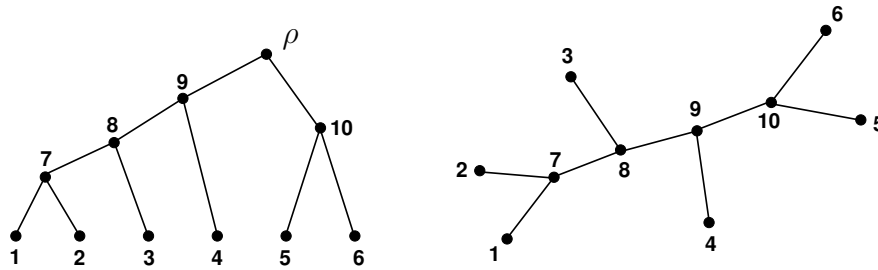
FIG. 2.1 – Exemple d'arbres phylogénétiques
