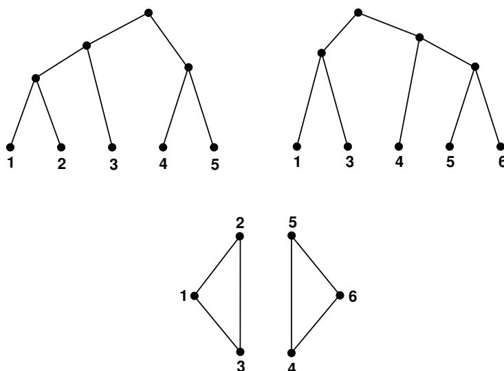
FIG. 4.2 – Construction du graphe représentant l'information topologique d'une collection de deux arbres
