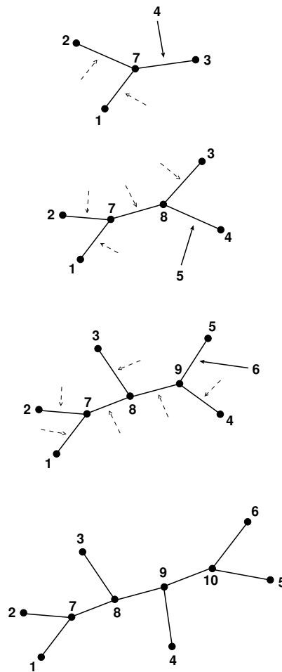
FIG. 2.4 – La procédure d'insertion pour construire un arbre phylogénétique non enraciné
