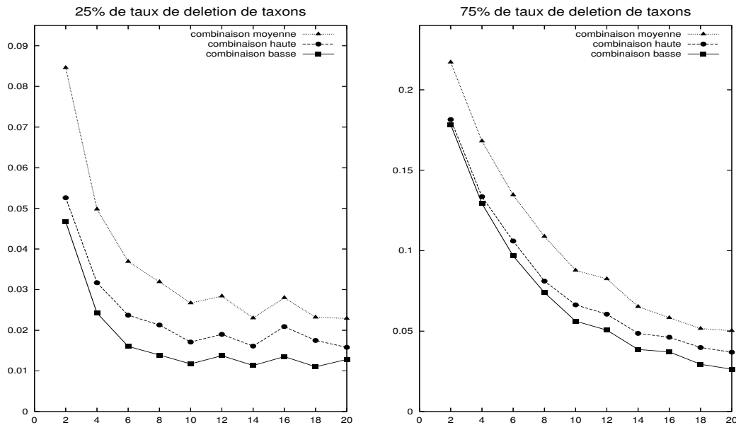
FIG. 7.4 – Performances des meilleurs scénarios de combinaison moyenne, haute et basse
