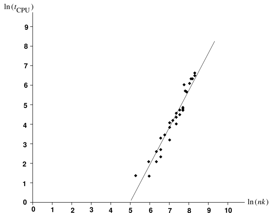
FIG. 5.1 – Estimation de la complexité en pratique de la résolution du système linéaire de la méthode SDM
