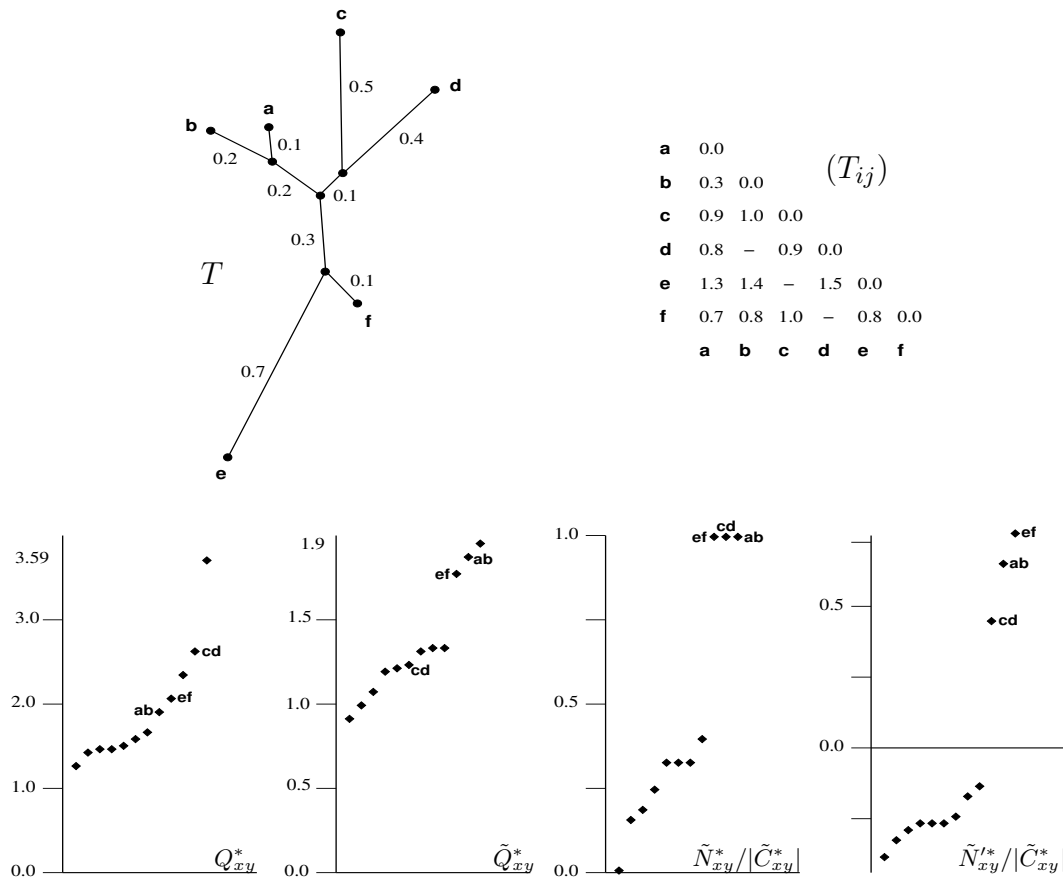
FIG. 6.2 – Distribution des valeurs des quatre critères d'agglomération Q_{xy}^* , \tilde{Q}_{xy}^* , \tilde{N}_{xy}^*/|\tilde{C}_{xy}^*| et \tilde{N}'_{xy}^*/|\tilde{C}'_{xy}^*|
