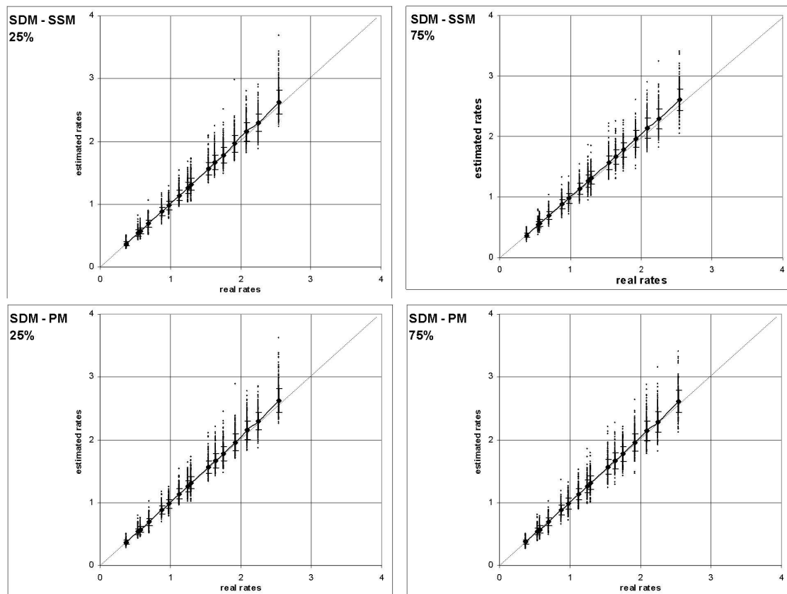
FIG. 5.2 – Observation de la stabilité des estimations des vitesses d'évolution relatives par SDM
