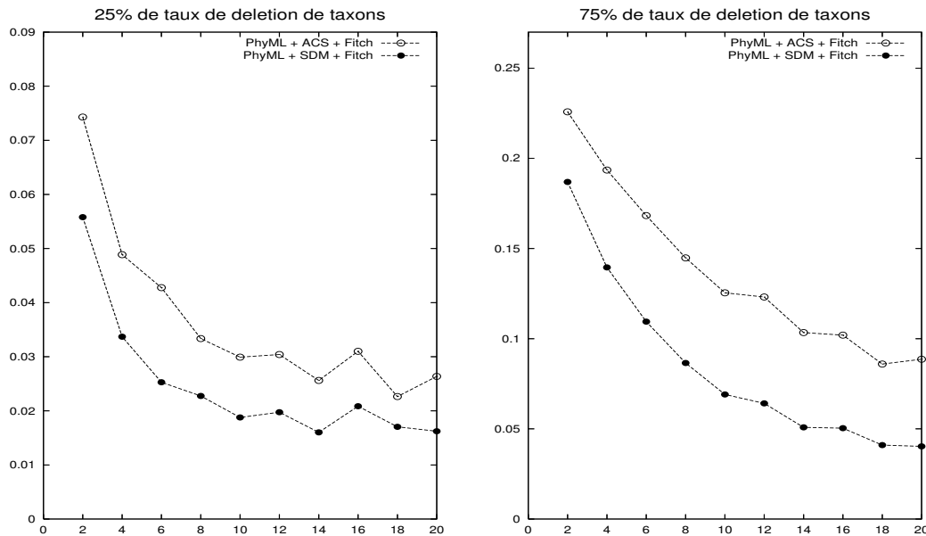
FIG. 7.3 – Performances des scénarios PHYML+ACS+FITCH et PHYML+SDM+FITCH
