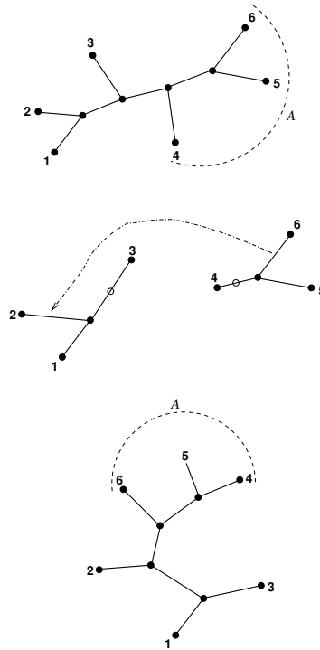
FIG. 2.8 – Réarrangement de type TBR
