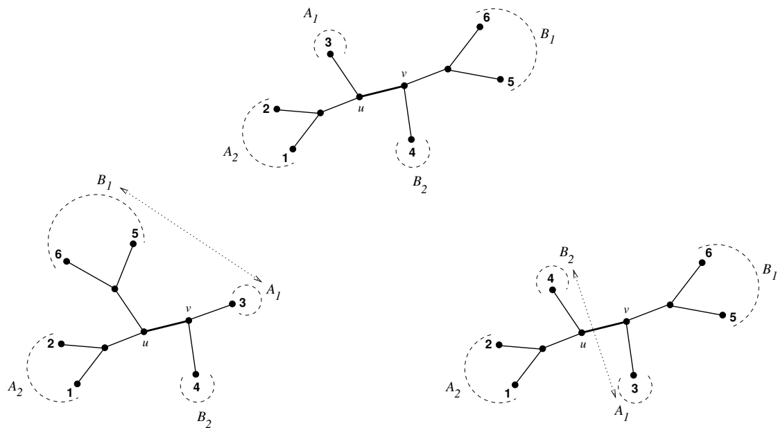
FIG. 2.6 – Réarrangement de type NNI
