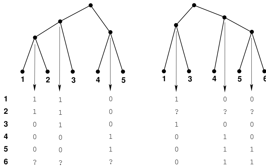
FIG. 4.3 – Construction de la représentation matricielle binaire de l'information topologique d'une collection de deux arbres
