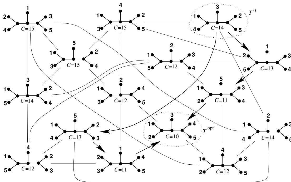
FIG. 2.5 – Exemple d'une recherche locale
