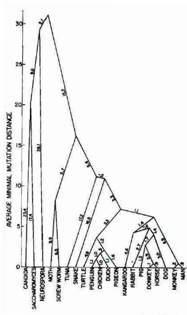
FIG. 1.3 – Arbre phylogénétique inféré par Fitch et Margoliash (1967)
