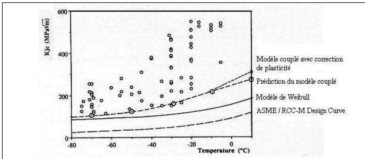
Figure I-20 : Evolution de la borne inférieure de probabilité en fonction de la température calculée par un couplage des modèles de Rousselier et de Beremin [Eripret - 96]
