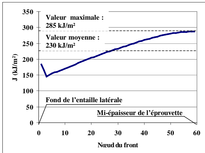
Figure III-15 : Evolution de J le long du front de fissure pour une valeur moyenne de 230 \text{kJ/m}^2 .
