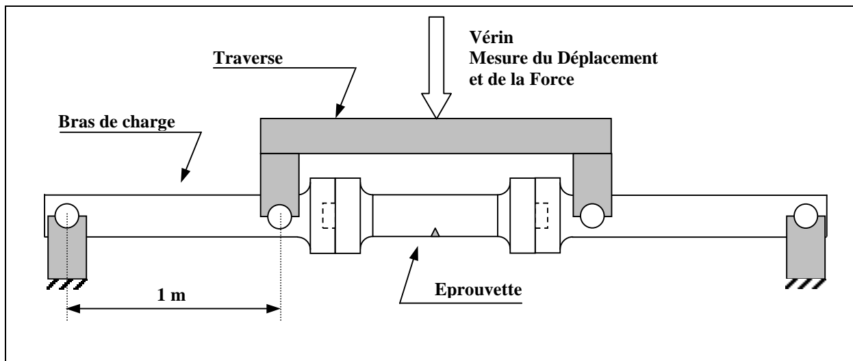
Figure VI-14 : Schéma du banc de flexion-4-points.
