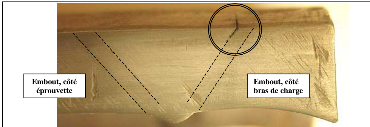
Figure VI-29 : Décollement dans la soudure de l'embout SUD.
