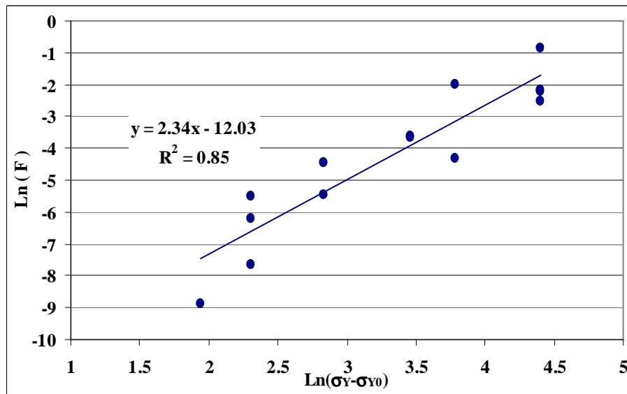
Figure II-23 : Corrélation entre F et la limite d'élasticité
