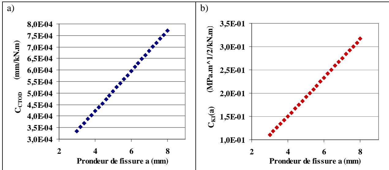
Figure VI-13 : Evolutions de la complaisance C_{CTOD} (a) et du rapport C_{KI} = \Delta KI/\Delta M^\circ (b) en fonction de la profondeur de fissure a.
