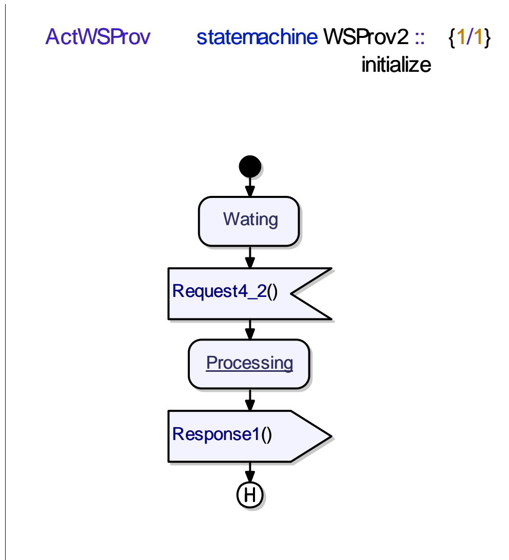
FIG. B.14 – Diagramme de machine à état du second service Web fournisseur.
