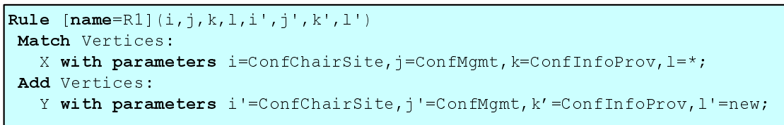
FIG. 5.12 – Règle R1 appliquée à l'action de duplication de services Web.
