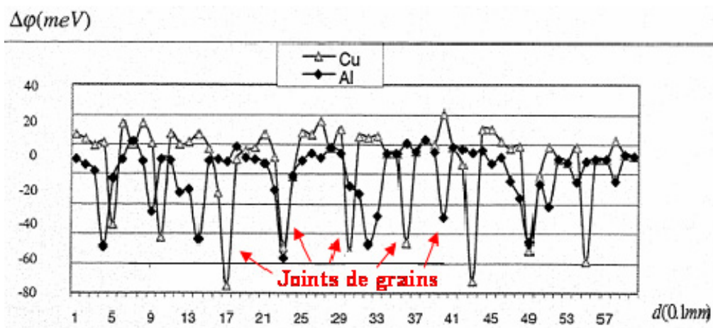
Figure IV.11. Potentiel de contact mesuré à l'aide d'une sonde Kelvin standard sur des couches polycristallines d'aluminium et de cuivre [Li2004].
