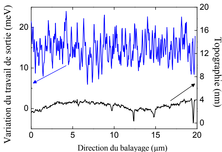
Figure IV.27. Profils topographique et électrique extraits le long des lignes pointillées des cartographies de la Figure IV.26.
