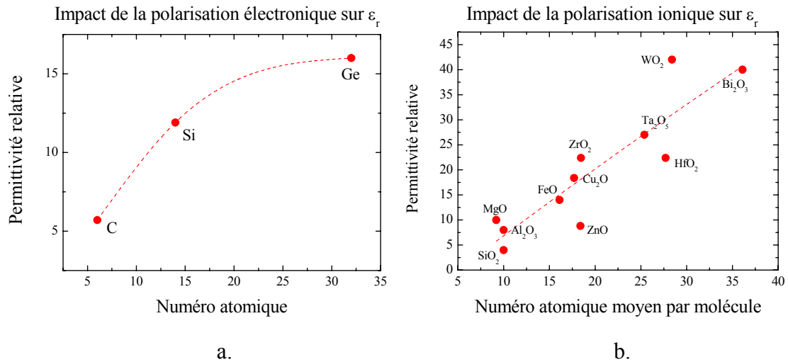
Figure I.15. (a) Permittivité relative du C, Si et Ge en fonction de leur numéro atomique et (b) permittivité relative en fonction du numéro atomique moyen de différents oxydes.
