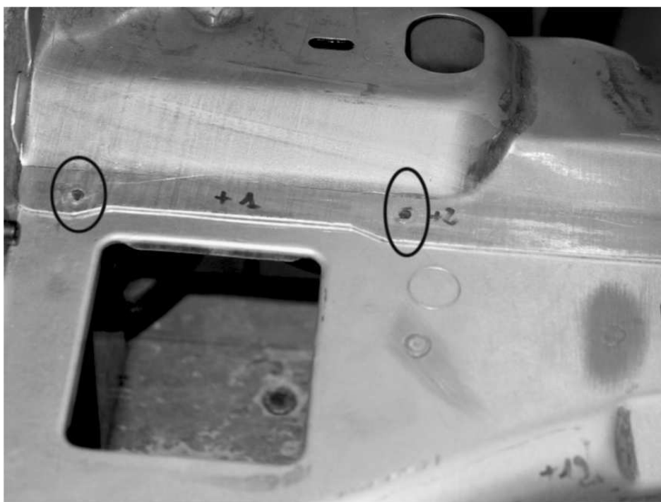
FIG. 8.12 – Vue du tablier, points de soudure 15 et 16 en place
