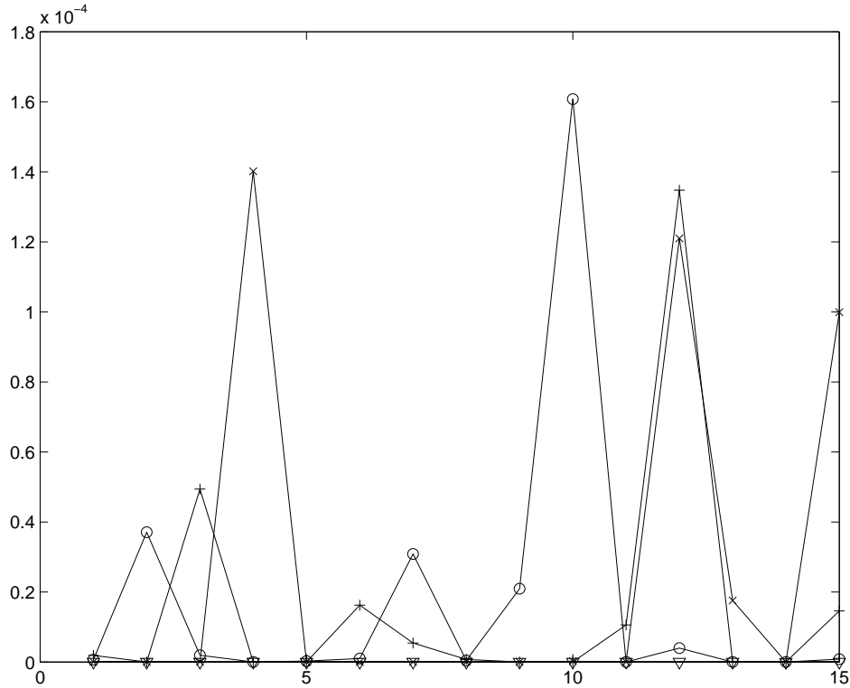
FIG. 6.12 – Carré de la sensibilité des valeurs propres vis-à-vis des angles de couplage, en fonction de l'ordre du mode considéré. 50 calculs. -o- : Angle 4 ; +- : Angle 5 ; -x- : Angle 7 ; -v- : Autres angles.
