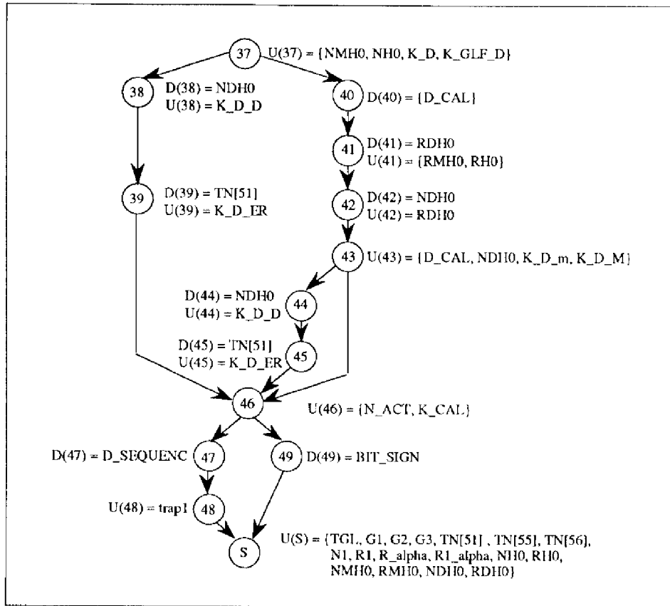
Partie 3 du graphe définition-utilisation de calcul-d-tsgv
