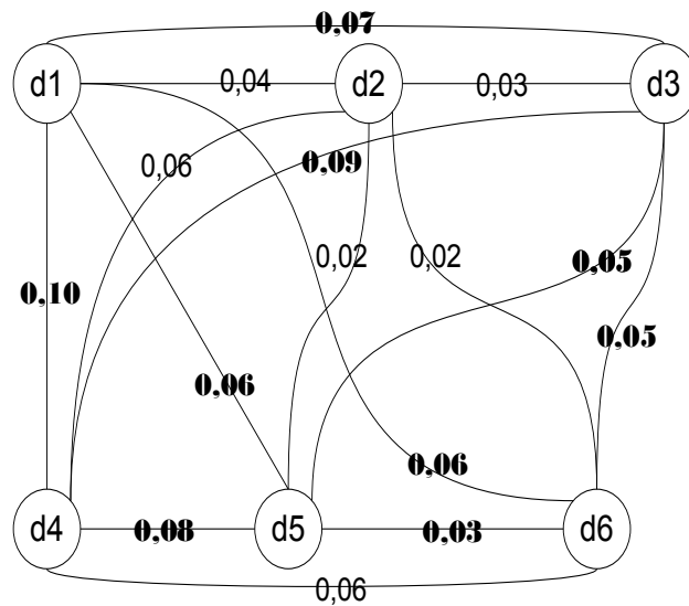
FIG. 4.5 – graphe de distance après application de l’algorithme de dijkstra
