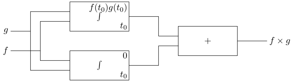
FIG. 2.3: Simulation d'un multiplicateur par des intégrateurs
