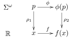
FIG. 2.1: \phi est une (\rho_1, \rho_2) -représentation de f
