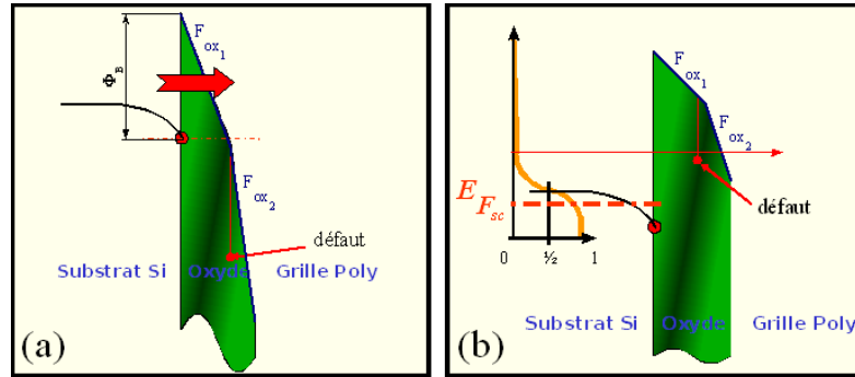
Figure 6.16: Diagrammes de bandes montrant l'origine des zones de limitation de la conduction des pièges présentées Figure 6.15
