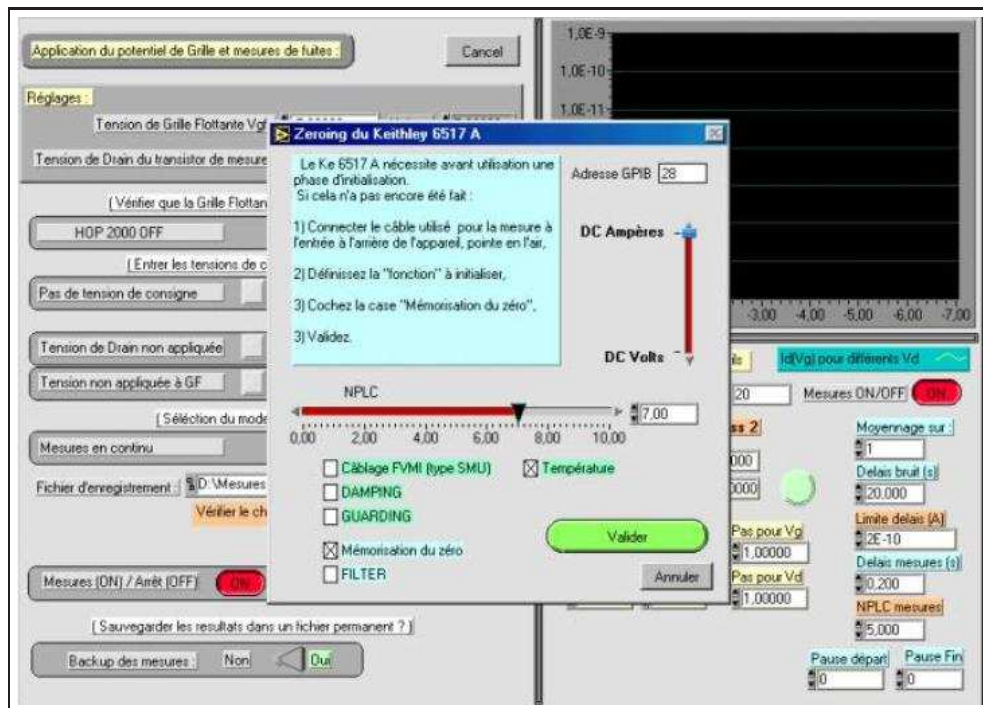
Figure B.5: Capture d'écran du logiciel d'acquisition; Initialisation de l'appareil KEITHLEY 617 A.
