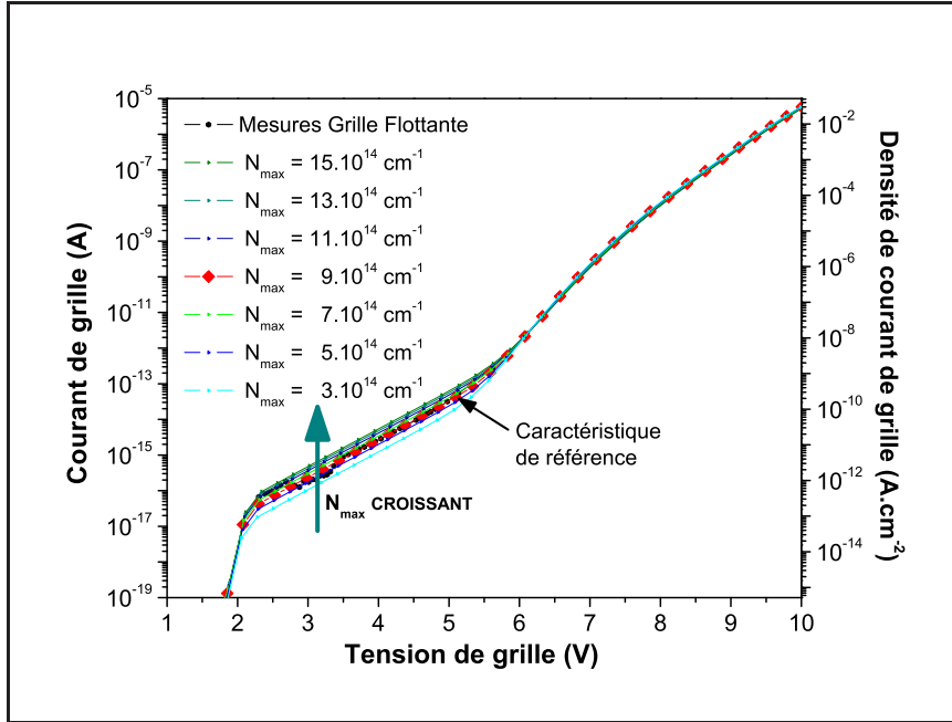
Figure 5.7: Évolution du courant SILC simulé en fonction du paramètre N_{\max} , dans la représentation semi-logarithmique.
