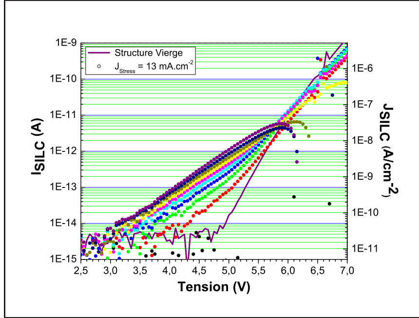
Figure 2.8: Exemple de visualisation d'un chargement global négatif de l'oxyde à travers l'apparition du kink.
