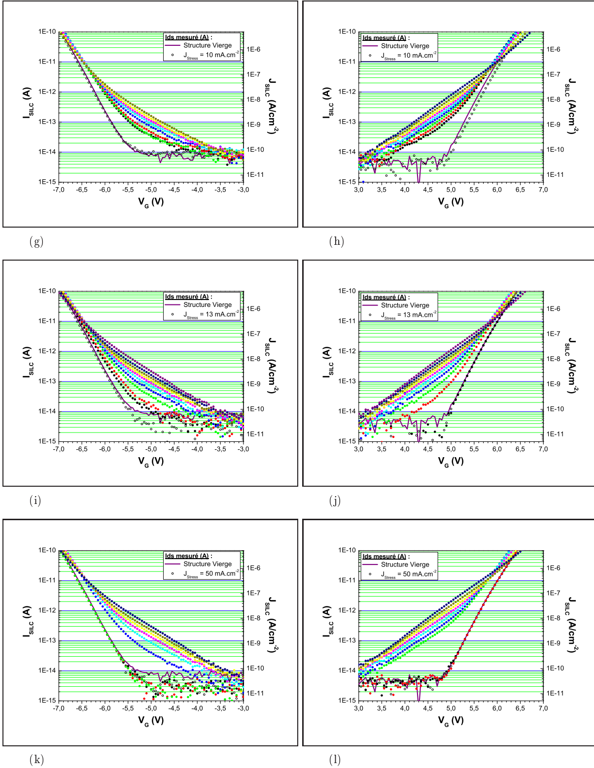
Figure 6.1: Réseaux de caractéristiques I-V pour des stress positifs et négatifs. Chaque réseau correspond à une densité de courant de stress constante. Les différentes courbes de chaque réseau correspondent à des quantités de charges injectées cumulées croissantes.
