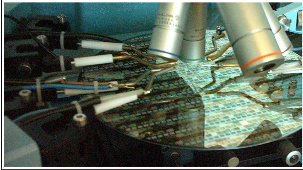
Figure 3.6: Photographie des bras portes-pointes et des connexions des câbles.
