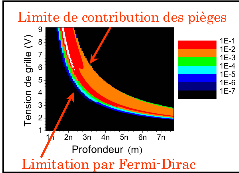
Figure 6.15: Distribution de probabilité de conduction d'un piège en fonction de sa position dans l'oxyde et du potentiel de grille appliqué à la capacité et définition des domaines de limitation de la conduction.
