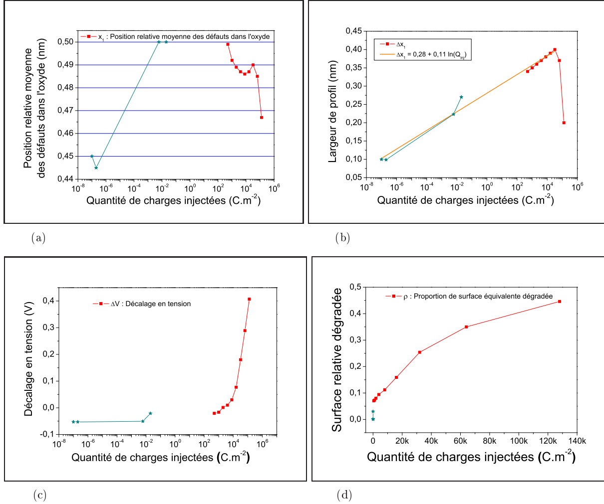
Figure 6.5: Évolution des paramètres des défauts pour le réseau de caractéristiques obtenu en mesures directes à J_{Stress} = +10 mA.cm^{-2} , en fonction de la quantité de charges injectées (■) et pour les mesures grille flottante présentées Figure 6.4(a) (*).
