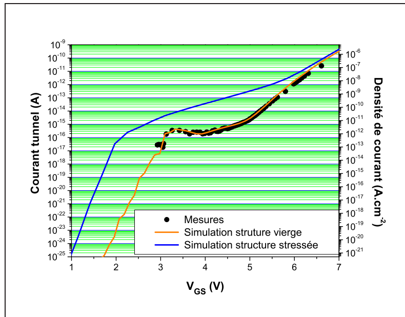
Figure 6.24: Caractéristiques I-V d'une structure GF 1 quasi-vierge et stressée à Q_{inj} = 16\,000\,C.m^{-2} .
