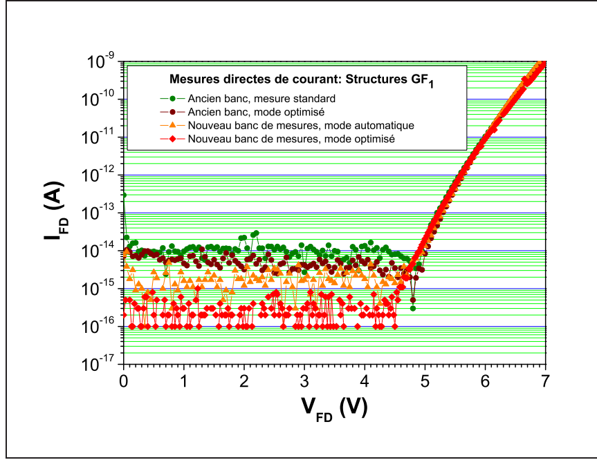
Figure 3.11: Courbes expérimentales I_{FD}(V_{FD}) comparant la résolution des mesures de courant tunnel obtenues sur le banc initial (●) et sur le nouveau banc : en mode automatisé (▲), et en mode optimisé (◆). S = 19\,360\,\mu\text{m}^2
