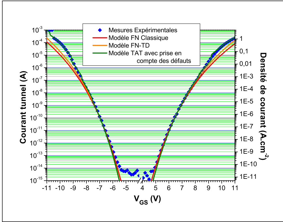
(a) Structure \text{GF}_1 : Comparaison entre le modèle classique ( Fig.4.8 ), le modèle tenant compte de la transparence (Modèle FN-TD) ( Fig.4.14 ) et le modèle tenant compte de la transparence et des défauts (Modèle TAT).
