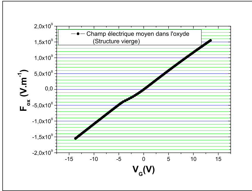
Figure 4.5: Structure GF 1 : Champ électrique moyen en fonction de la polarisation de grille, calculé à l'aide de l'équation (4.13).
