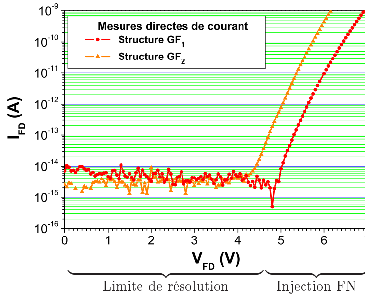
Figure 3.4 : Caractéristiques I-V de l'oxyde tunnel, réalisées avec le banc de mesures initial, sur une structure GF 2 (▲) et sur une structure GF 1 (●). Une résolution de 7 \cdot 10^{-15} A est atteinte. Le décalage en courant, observé entre les deux courbes en régime d'injection Fowler-Nordheim, est dû à la différence des épaisseurs et surfaces tunnel des deux types de structures.
