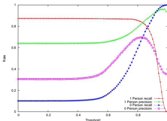
FIG. 3.13 – Résultat de classification personne et non-personne. L'axe horizontal représente la variation de seuil_{person} , l'axe verticale représente le taux de reconnaissance.
