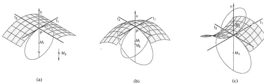
FIG. 2.2 – Classification de la surface via la relation de deux courbures principales. (a) \lambda_1 \lambda_2 = 0 Parabolique. (b) \lambda_1 \lambda_2 > 0 Elliptique. (c) \lambda_1 \lambda_2 < 0 Hyperbolique. Les deux directions principales sont t_1, t_2 . Les deux courbures principales sont inverses du rayon des cercles osculateurs.
