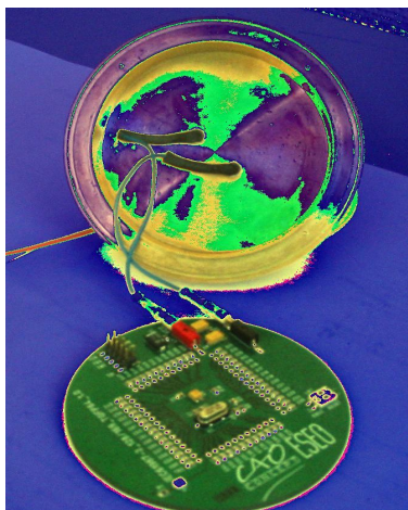
Figure V-40.a. Cloche avec la carte de test
