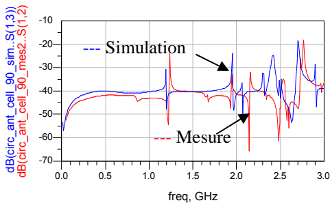
Figure III-10. Paramètre de couplage S12 entre la cellule et l'antenne : Orientation 90°
