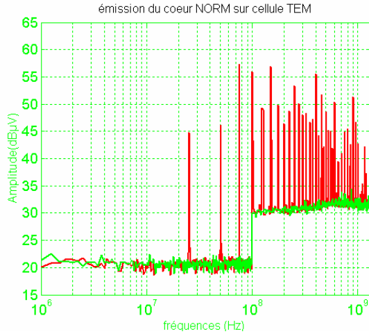
Figure III-61. Niveau d'émission + bruit du cœur Norm
