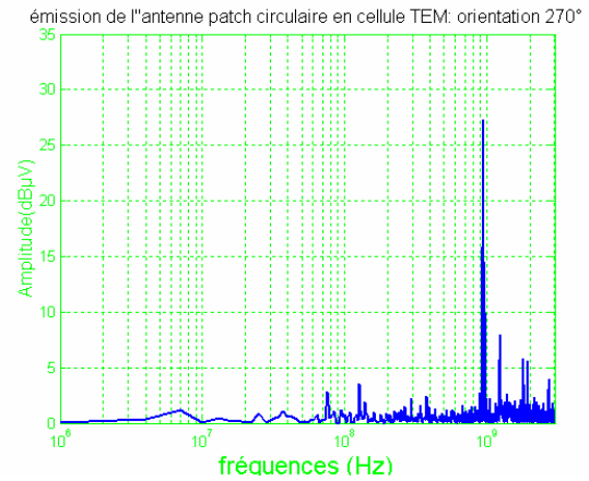
Figure III-22. Analyse spectrale de l'émission
