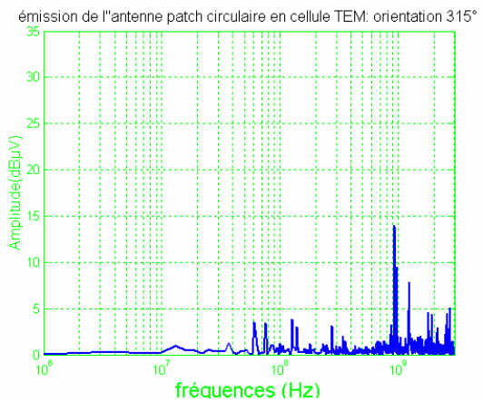
Figure III-24 . Analyse spectrale de l'émission de l'antenne : Orientation 315°
