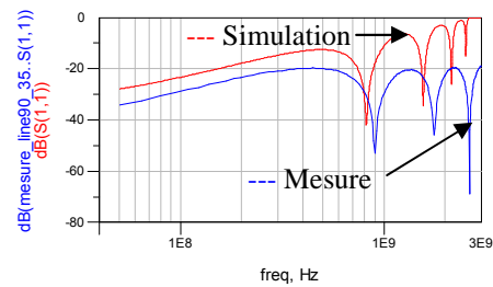
Figure IV-17. Paramètre S11 de la cellule (mesure & simulation)
