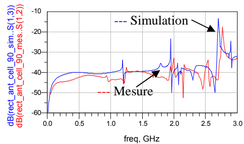
Figure III-34. Mesures d'antenne dans la direction Ouest
