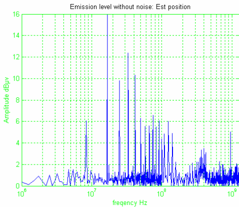
Figure III-50. Niveau d'émission en cellule TEM : position EST
