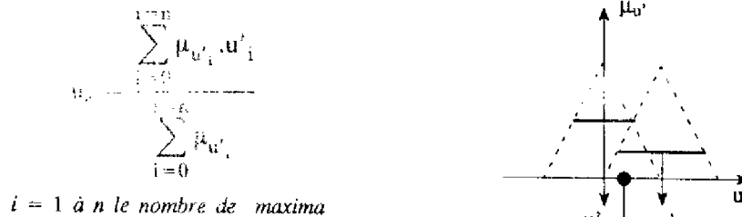
Figure 9 : Défuzzification par le centre des maxima
