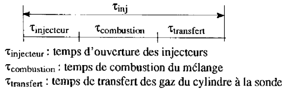
Figure 41 : Décomposition du retard \tau_{inj}
