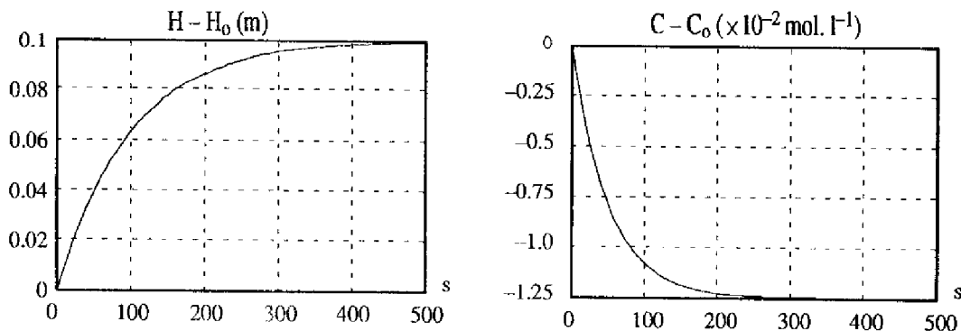
Figure 66 : Evolution des sorties avec q 1 =1 l s -1 et q 2 =0 l s -1
