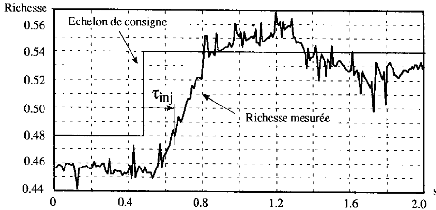
Figure 40 : Richesse en boucle ouverte avec un échelon de temps d'injection
