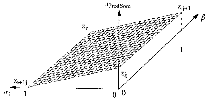
Figure 17 : Surface de commande avec un raisonnement produit-somme
