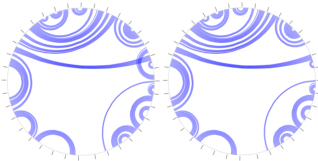
Fig. 8.6: Version originale et aplanie de la structure d'un intron du groupe 1 chez B. atropupurea
