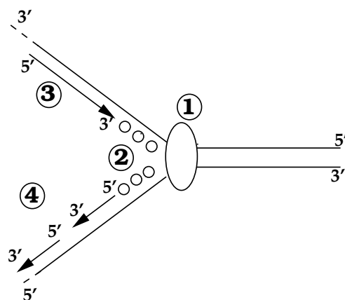
Fig. 6.8: Réplication de l'ADN
