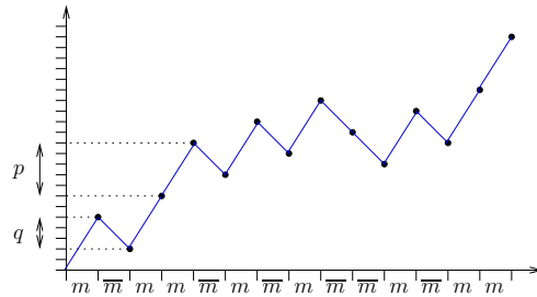
Fig. 9.1: Encodage d'un chemin par un mot sur \{m, \overline{m}\}^*
