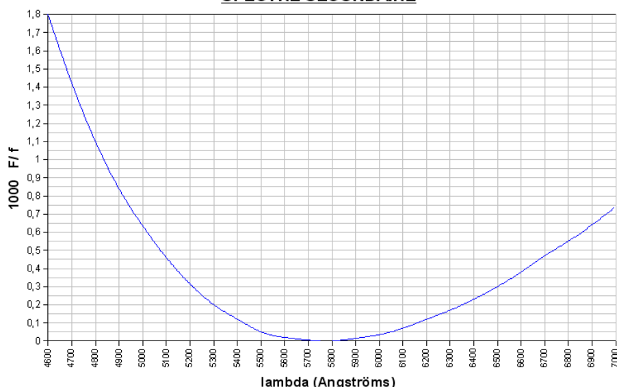
Illustration 2.2.2: Spectre secondaire (aberration chromatique) de l'objectif de la LJR (doc. F. Chauveau).
