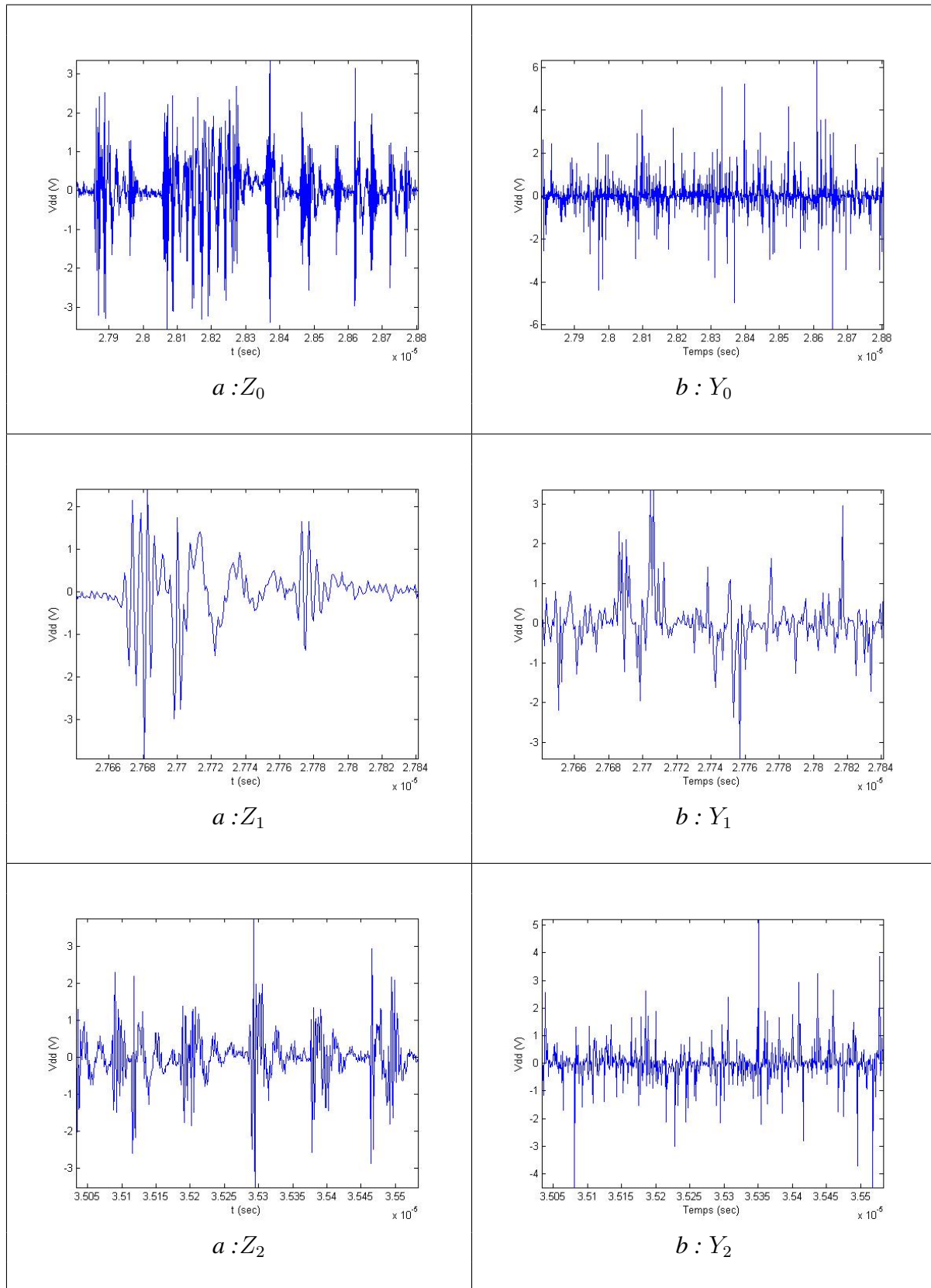
FIG. 9 – Z_i (a) accompagnés de leurs Y_i respectifs (b), i = 0 \dots 2
