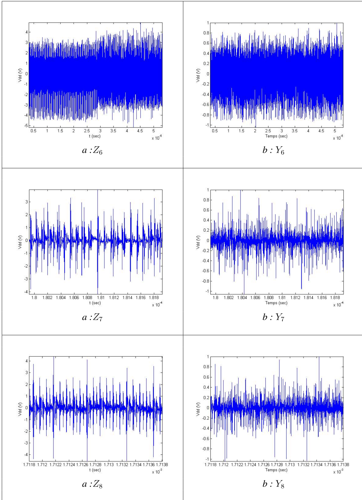
FIG. 3 – Z_i (a) accompagnés de leurs Y_i respectifs (b), i = 6 \dots 8
