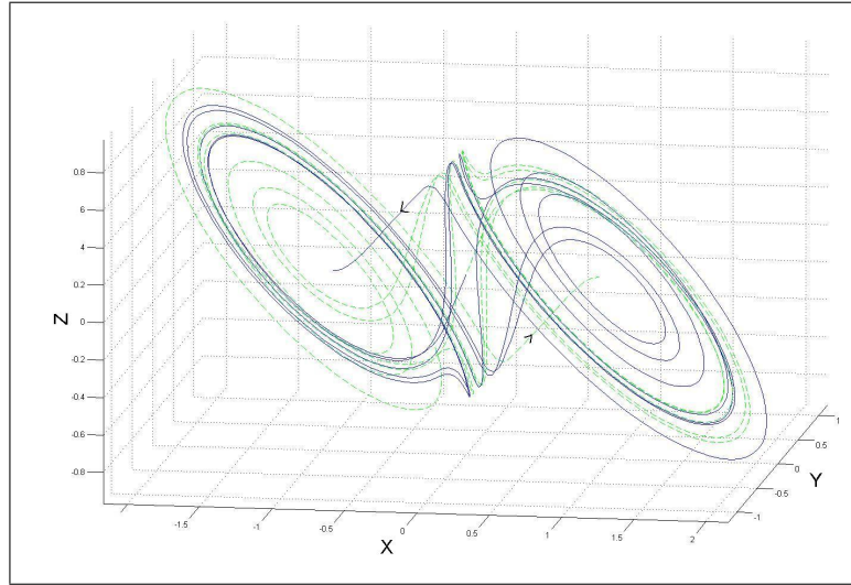
FIG. 12 – Trajectoires hétéroclines obtenues avec a = -0,7 . Les trajectoires sont représentées par 1000 points avec un pas de discrétisation h = 0,1 , issues de conditions initiales proches et symétriques par rapport à P_0 .
