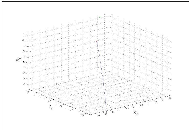
FIG. 9 – Perturbation du système au voisinage de P_0 . Pour a = -0,7 , la solution diverge très rapidement
