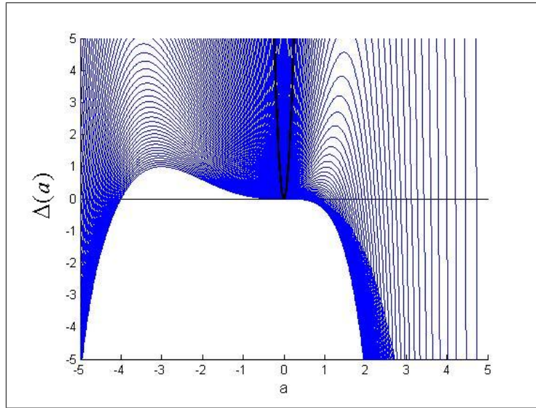
FIG. 2 – Représentation graphique de l'application qui à tout a \in \mathbb{R} associe \Delta(a) pour plusieurs valeurs de \eta \in ]0 ; 1[ . La courbe en gras est celle où \eta = 0, 1 .
