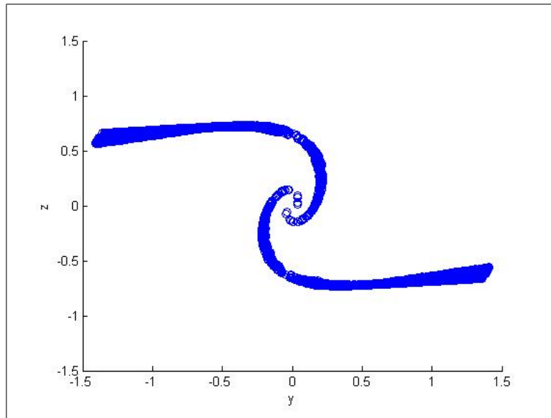
FIG. 23 – Section de Poincaré x = 0 avec a = -0,7 sur N = 1000000 points avec un pas h = 0,1 .
