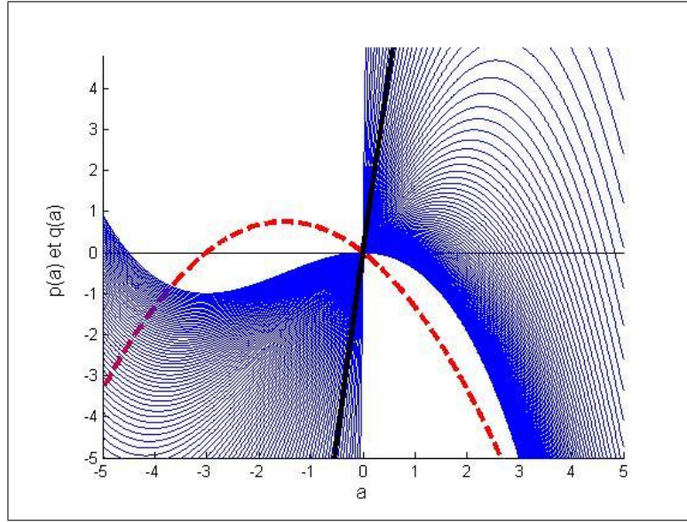
FIG. 1 – Représentation graphique de p (trait pontillés), et de q (traits pleins) en fonction de a pour différentes valeurs de \eta . En gras le cas où \eta = 0, 1 .
