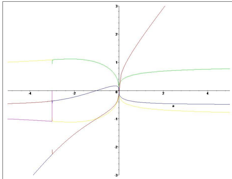
FIG. 2 – Représentation graphique des applications qui à tout a \in \mathbb{R} font correspondre les parties réelles et imaginaires des valeurs propres \{\lambda_i\}_{i=1, \dots, 3} : \lambda_1(a) (en rouge), Re[\lambda_2(a)] (en bleu), Im[\lambda_2(a)] (en vert), Im[\lambda_3(a)] (en jaune) et si a < -3 , Im[\lambda_1(a)] (en magenta)
