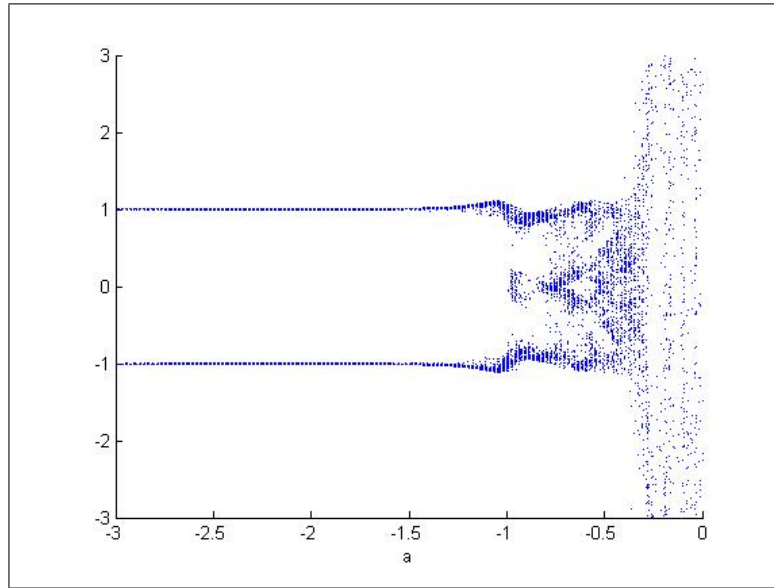
FIG. 14 – Diagramme de bifurcation pour a \in [-3 ; 0] . En ordonnée, pour chaque valeur de a , les N_{tir} = 50 valeurs moyennes de 600 échantillons de la solution de ( P_a ).
