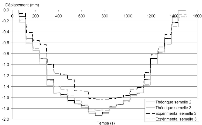
FIG. 4.9 – Déplacement vertical des deux semelles libres lors du test de l'instrumentation
