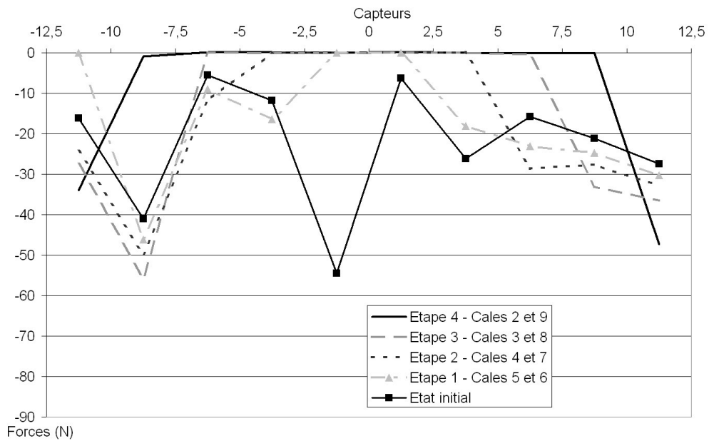
FIG. 3.28 – Evolution des efforts sur les cales mobiles durant l'essai n°4
