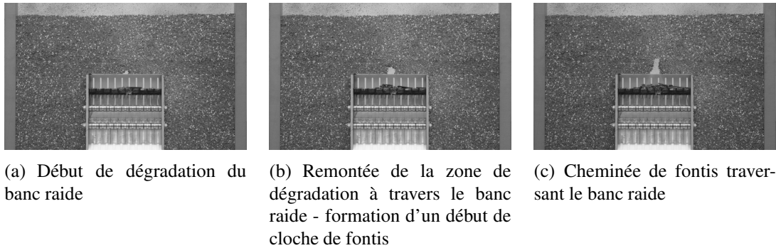
FIG. 3.7 – Photos prises lors de la dégradation du banc raide par injection d'eau
