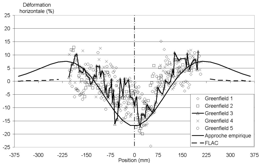
FIG. 7.15 – Evolution de la déformation horizontale en surface pour les cinq simulations
