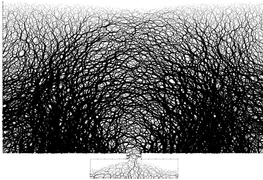
FIG. 8.9 – Réseau des forces de contact inter-particulaires
