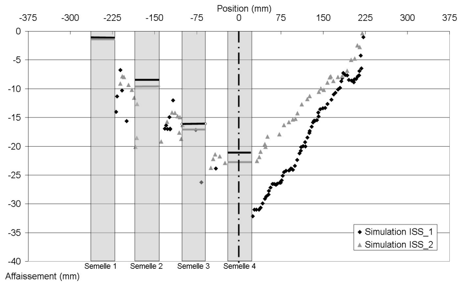
FIG. 7.20 – Déplacements verticaux en surface obtenus en présence de la structure
