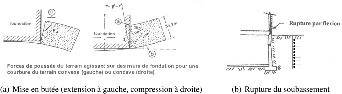
FIG. 1.20 – Mise en butée du sol et rupture d'une fondation par flexion dans Deck (2002)
