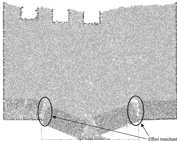
FIG. 7.17 – Etat final du modèle couplé avec la structure (état post-rupture pour la simulation n°2)
