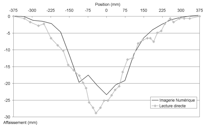
FIG. 3.38 – Comparaison des cuvettes obtenues par corrélation d'images et par lecture directe sur les photos pour l'essai 8
