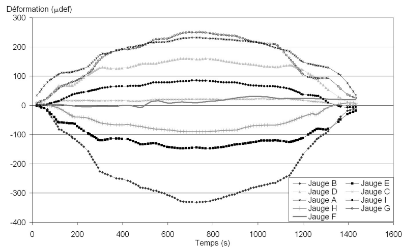
FIG. 4.10 – Déformations dans les jauges lors du test de l'instrumentation
