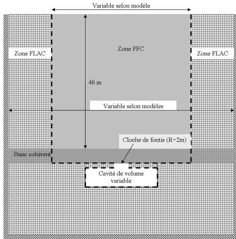
FIG. 8.4 – Géométrie utilisée par le modèle numérique couplé représentant la configuration du massif de L'Hautil
