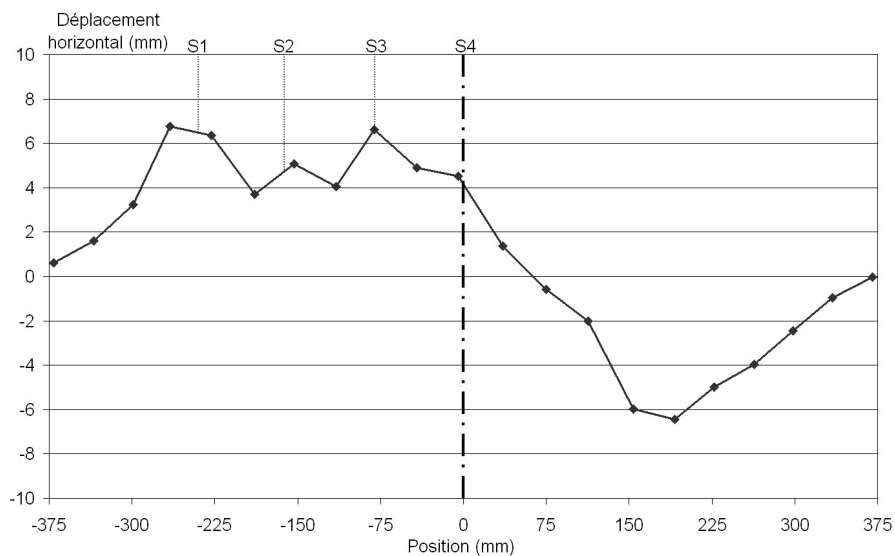
FIG. 4.26 – Déplacements horizontaux pour l'essai 13
