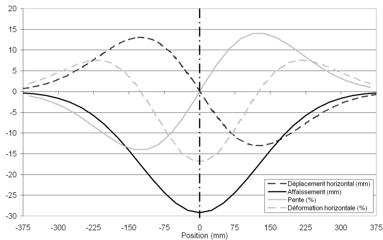
FIG. 1.13 – Allure générale des déplacements et déformations par l'approche de Peck
