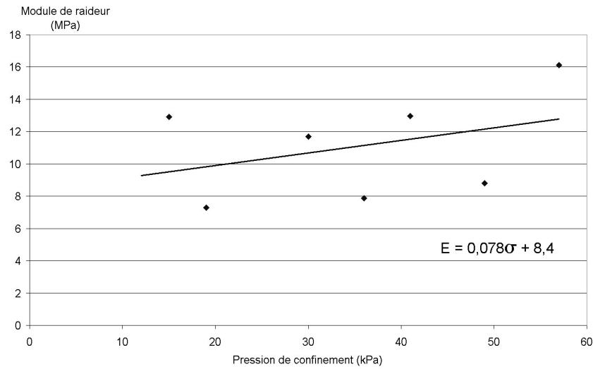
FIG. 2.24 – Evolution du module de raideur initiale en fonction de la pression de confinement - Matériau C/8
