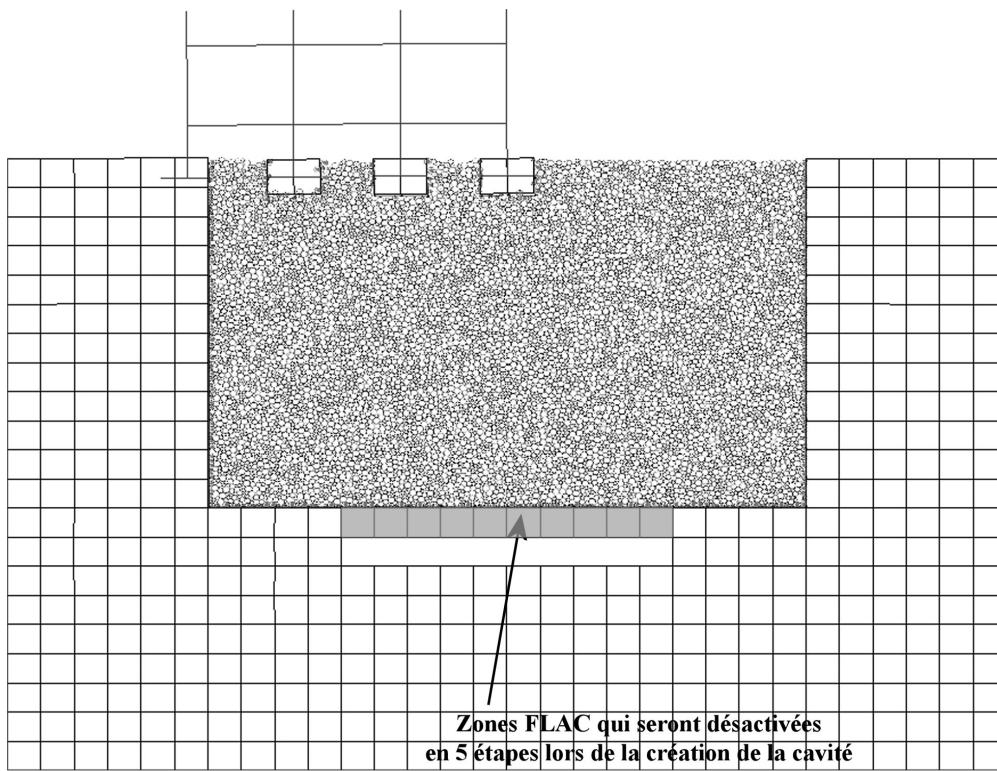
FIG. 7.3 – Assemblage des parties FLAC et PFC de la modélisation couplée en présence de la structure
