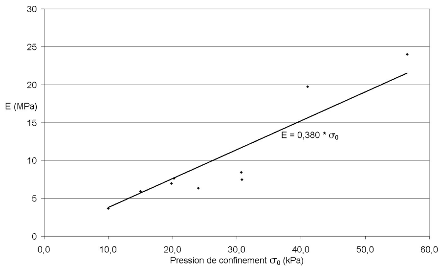
FIG. 2.16 – Modules de raideur initiale en fonction du confinement
