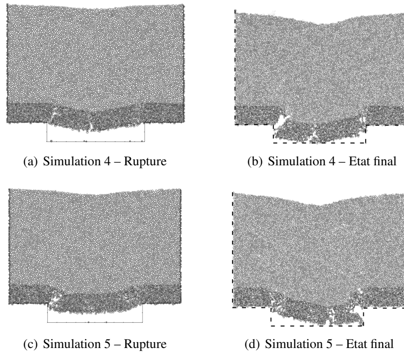
FIG. 7.5 – Rupture et état final pour les simulations n°4 et 5
