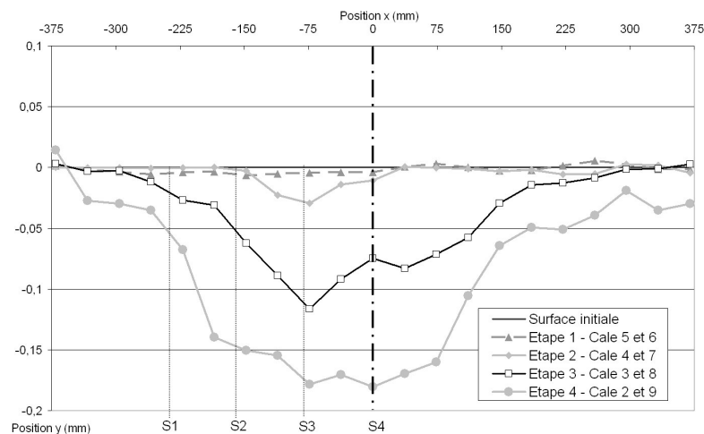
FIG. 4.24 – Affaissements en surface avant la rupture - essai 13
