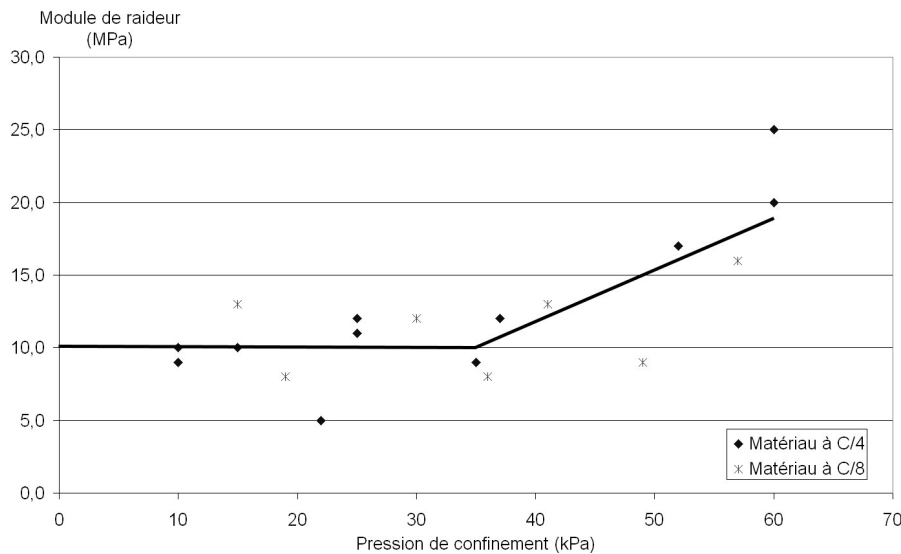
FIG. 2.26 – Module de raideur en fonction du confinement pour les deux concentrations de colle
