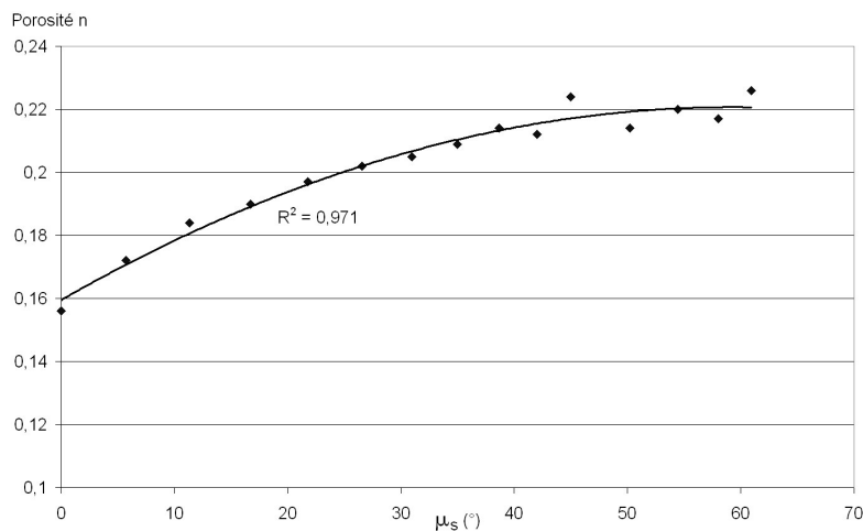
FIG. 6.4 – Variation de la porosité initiale en fonction de l'angle de frottement interne utilisé pour la création de l'éprouvette
