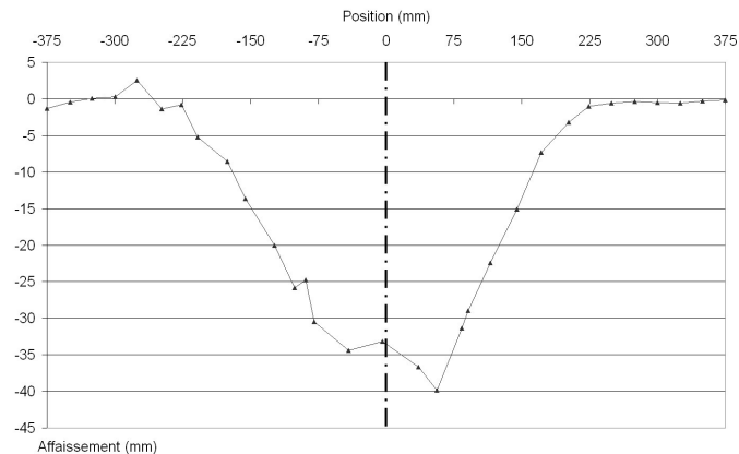
FIG. 3.15 – Cuvette d'affaissement obtenue lors de la rupture de l'essai 2
