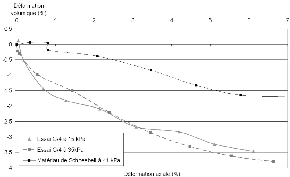
FIG. 2.21 – Déformations volumiques pour deux essais avec des échantillons à C/4
