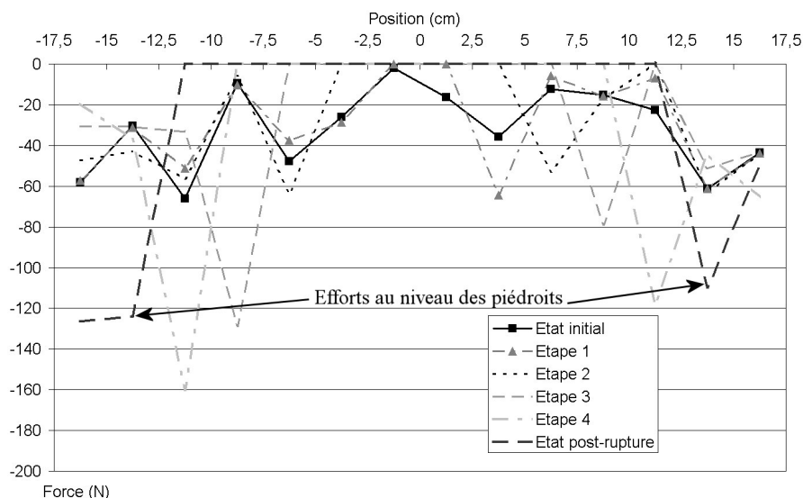
FIG. 7.19 – Evolution des reports de charge au cours de la création de la cavité pour la première simulation
