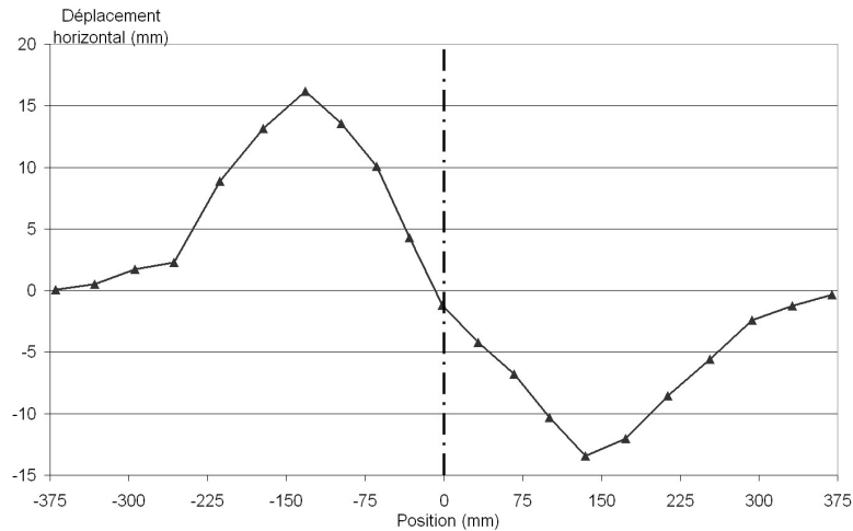
FIG. 3.35 – Déplacements horizontaux pour l'essai 7
