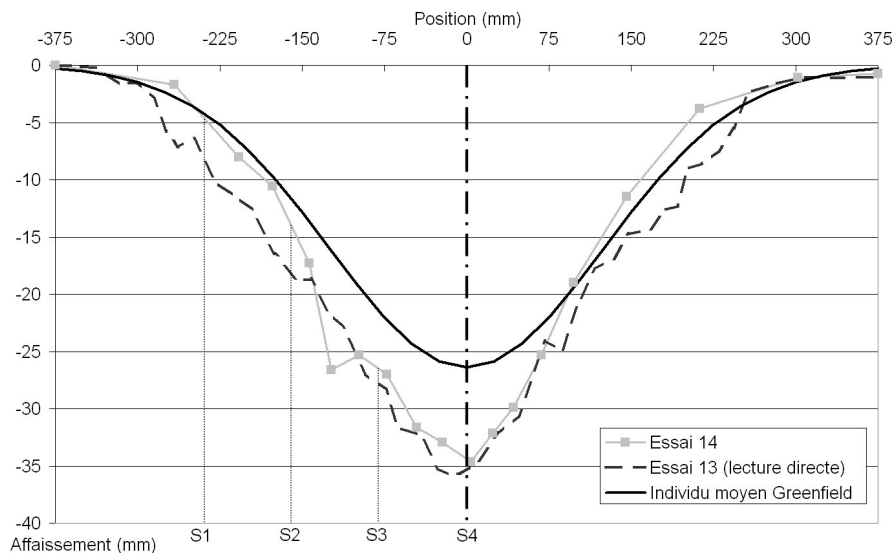
FIG. 4.46 – Comparaison des cuvettes d'affaissement Greenfield et ISS
