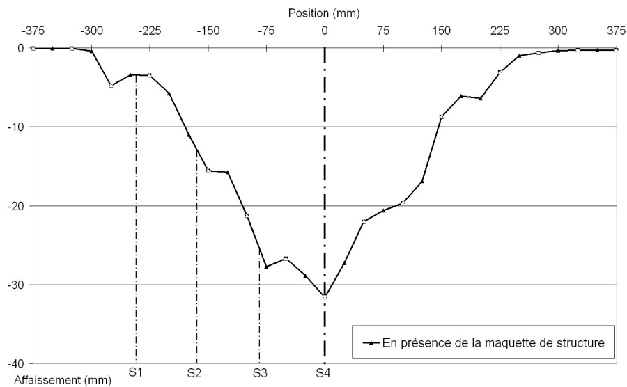
FIG. 4.16 – Cuvette d'affaissement post-rupture - Essai 10
