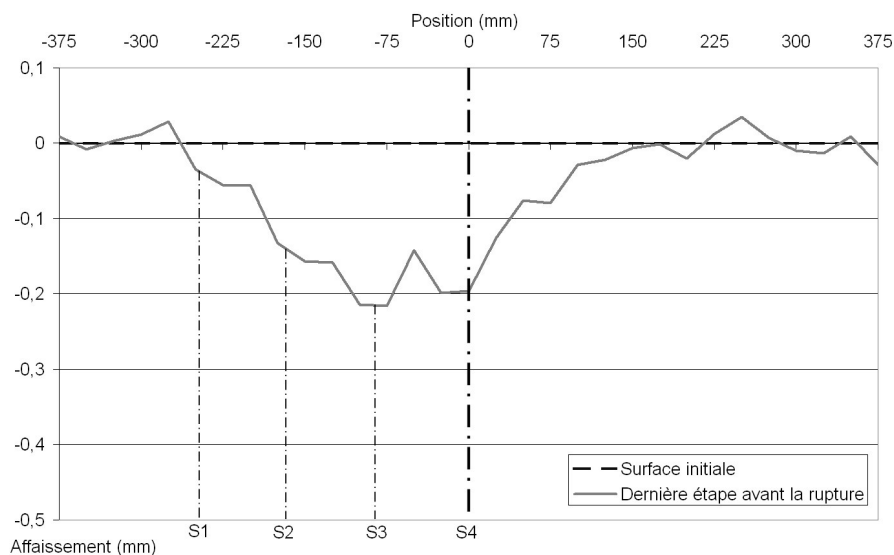
FIG. 4.21 – Affaissement en surface avant la rupture – Essai 10
