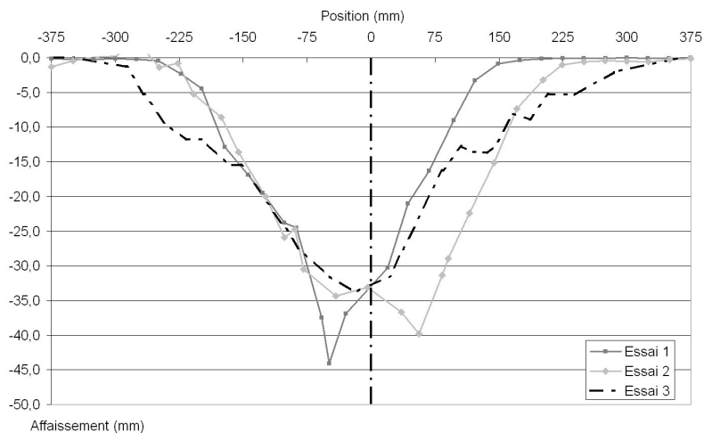
FIG. 3.19 – Cuvettes d'affaissement pour les essais n°1, 2 et 3
