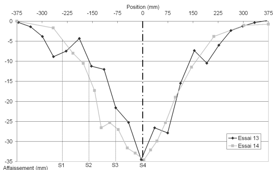
FIG. 4.36 – Cuvettes d'affaissement post-rupture
