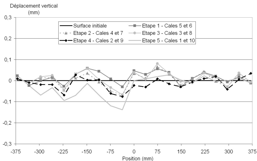
FIG. B.2 – Déplacements en surface après correction - Essai 9 - étapes de création de la cavité
