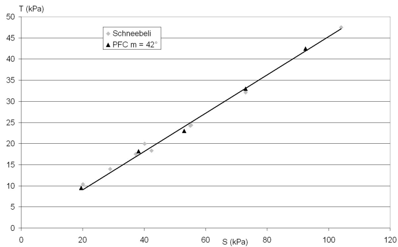
FIG. 6.6 – Résultats pour les essais expérimentaux et le modèle PFC après calage - plan déviatorique S–T avec S = (\sigma_1 + \sigma_2)/2 et T = (\sigma_1 - \sigma_2)/2
