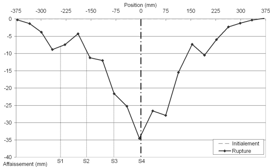
FIG. 4.25 – Cuvette d'affaissement lors de la rupture - essai 13
