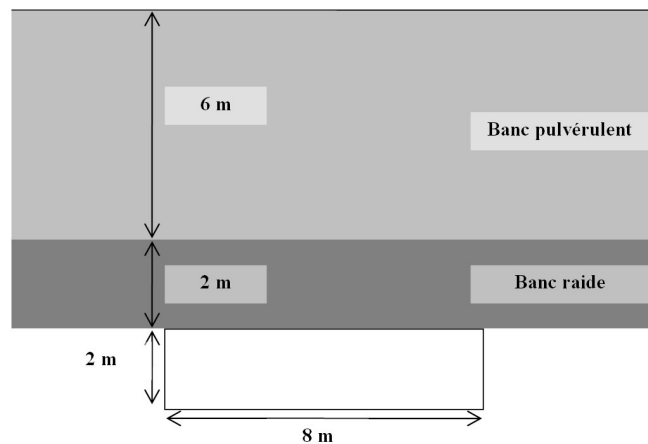
FIG. 2.3 – Coupe schématique de la cavité et de son recouvrement utilisé
