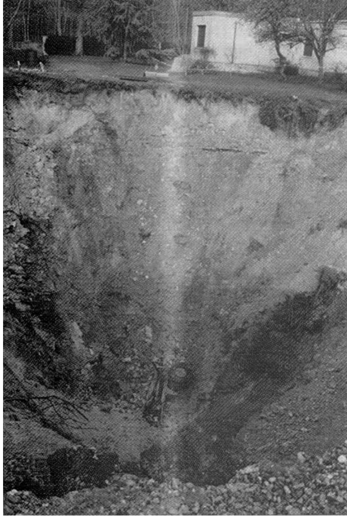
FIG. 8.1 – Photo du fontis survenu le 11 mars 1991 à Chanteloup-Les-Vignes (Photo INERIS)
