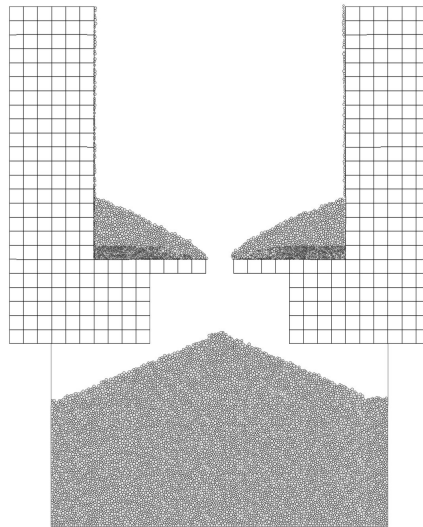
FIG. 8.6 – Etat final de la première simulation
