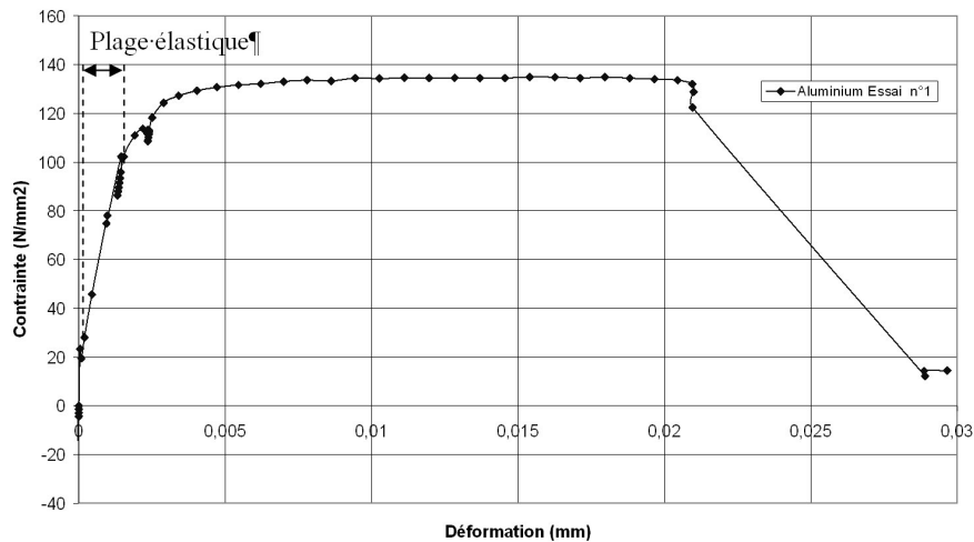
FIG. C.3 – Essai de traction simple sur l'aluminium
