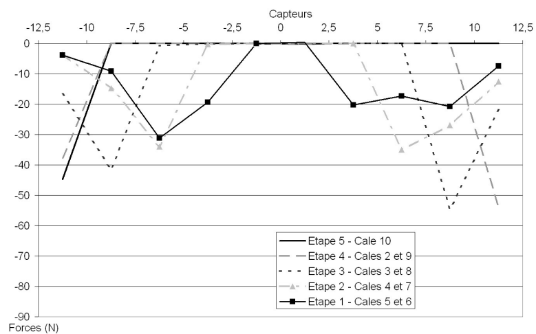
FIG. 3.31 – Evolution des efforts sur les cales mobiles durant l'essai n°5
