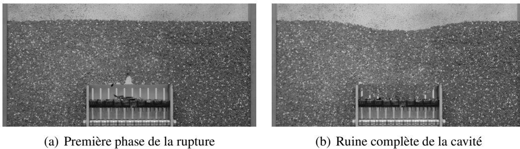
FIG. 3.14 – Deux phases de rupture pour l'essai 2
