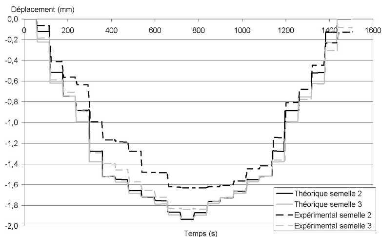
FIG. 4.9 – Déplacement vertical des deux semelles libres lors du test de l'instrumentation
