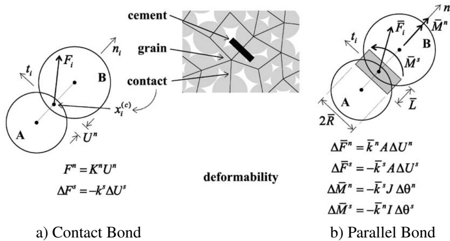
FIG. 5.3 – Schéma des deux types de liaisonnement (Potyondy & Cundall 2004)
