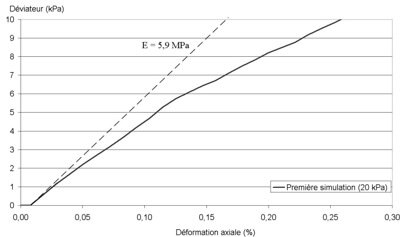
FIG. 6.3 – Courbe contrainte-déformation pour le premier essai biaxial sous PFC
