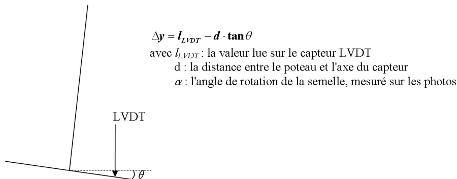
FIG. 4.49 – Schema de principe pour l'incertitude sur la rotation des semelles
