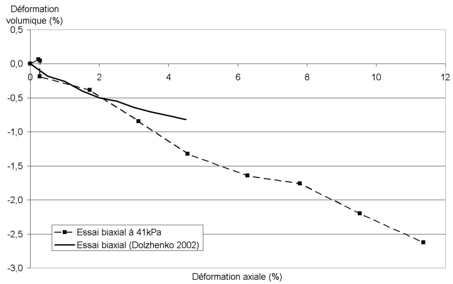
FIG. 2.15 – Déformations volumiques de l'essai à 41 kPa
