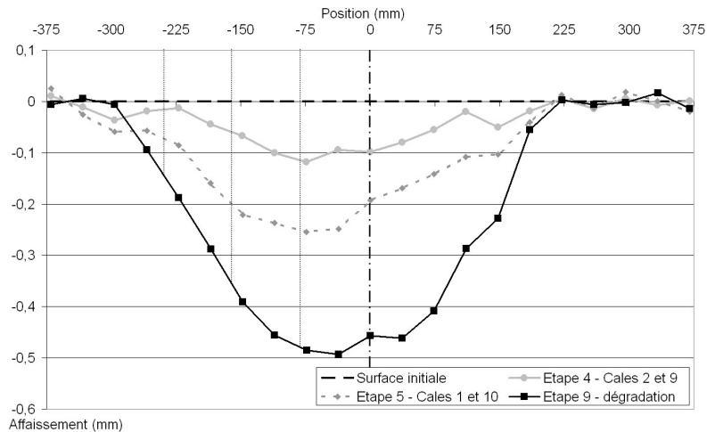
FIG. 4.29 – Déplacements en surface avant la rupture - Essai 14
