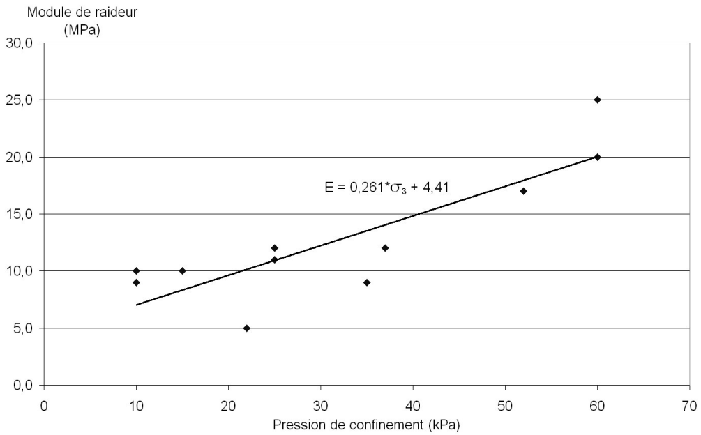
FIG. 2.20 – Evolution du module de raideur avec la pression de confinement
