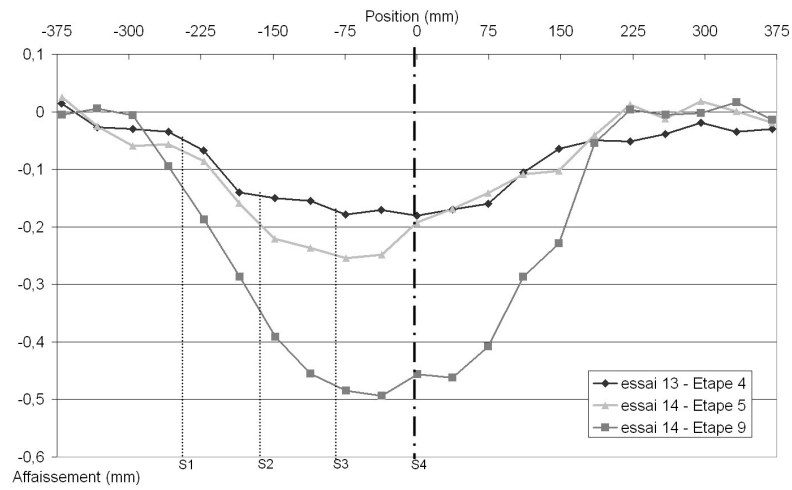
FIG. 4.35 – Déplacements verticaux en surface avant la rupture – Essai 13 et 14
