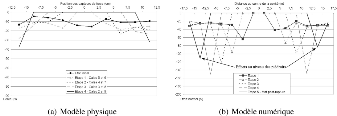
FIG. 7.16 – Deux exemples de report de charge
