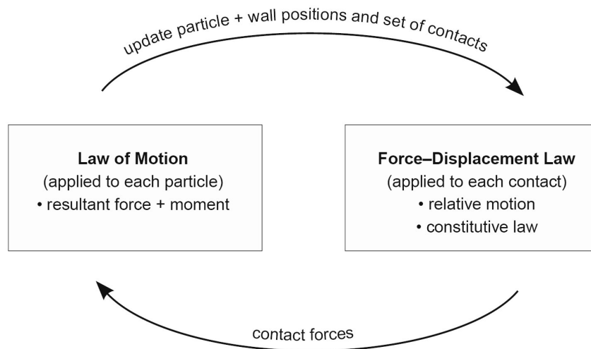
FIG. 5.1 – Cycle de base de l’algorithme utilisé par PFC (extrait de Itasca (2005b))
