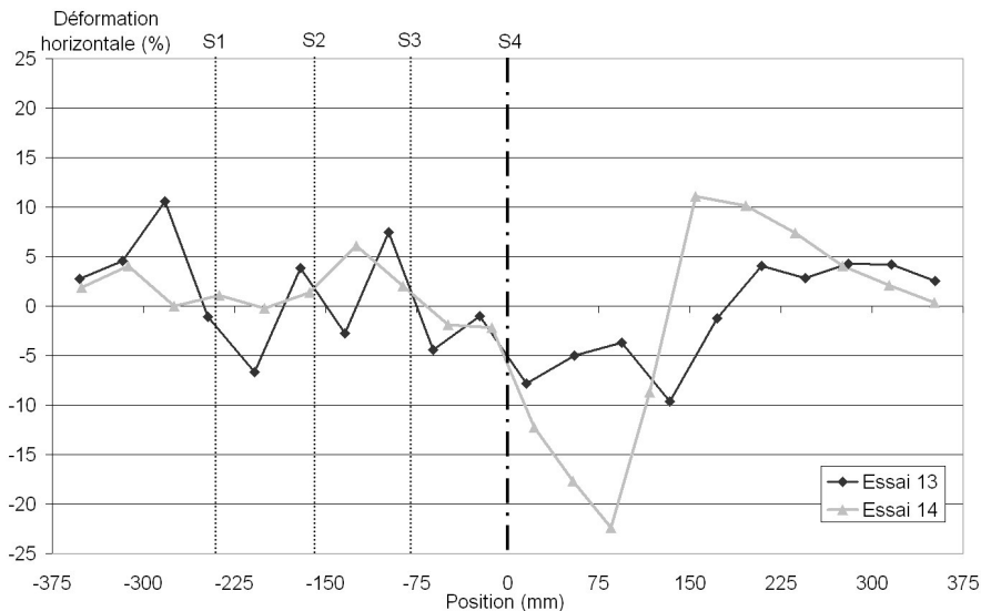
FIG. 4.41 – Déformations horizontales en surface – Essai 13 et 14
