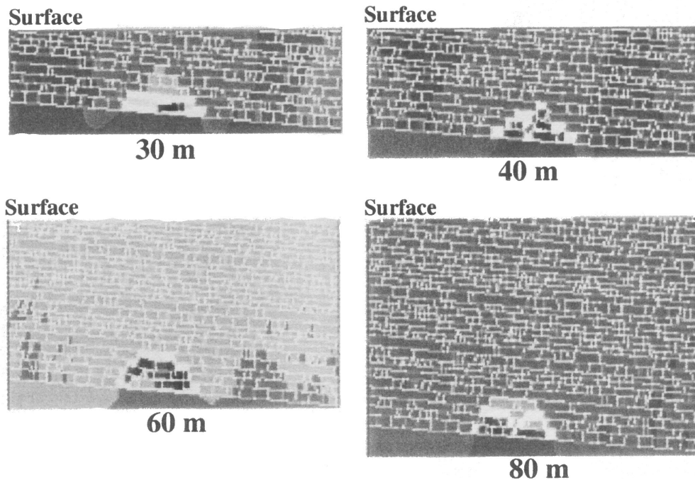
FIG. 1.9 – Formation d'une cloche de fontis obtenue par Didier et al. (2003) pour un recouvrement fracturé, l'épaisseur du recouvrement variant de 30 à 80 m.
