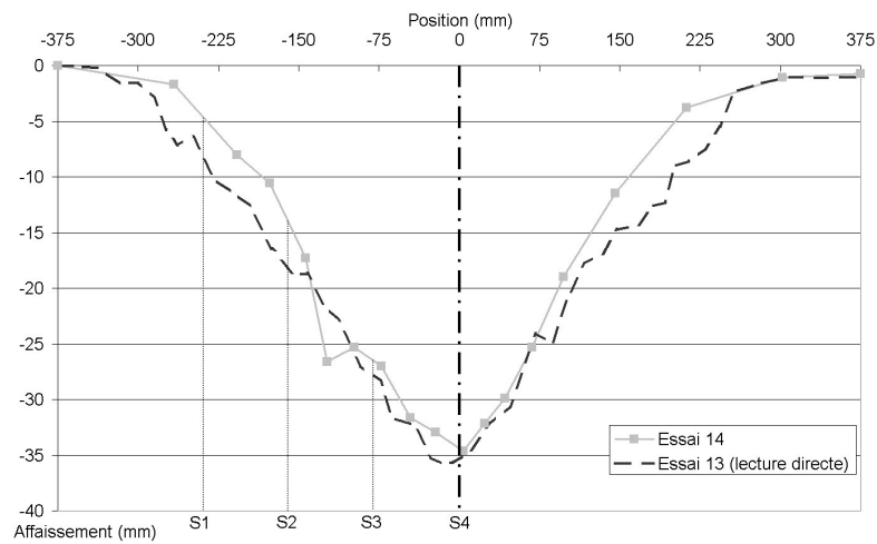
FIG. 4.38 – Comparaison de la cuvette d’affaissement pour les essais n°13 et 14
