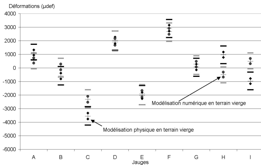
FIG. 7.27 – Déformations dans la structure correspondant aux mouvements du sol en condition de terrain vierge
