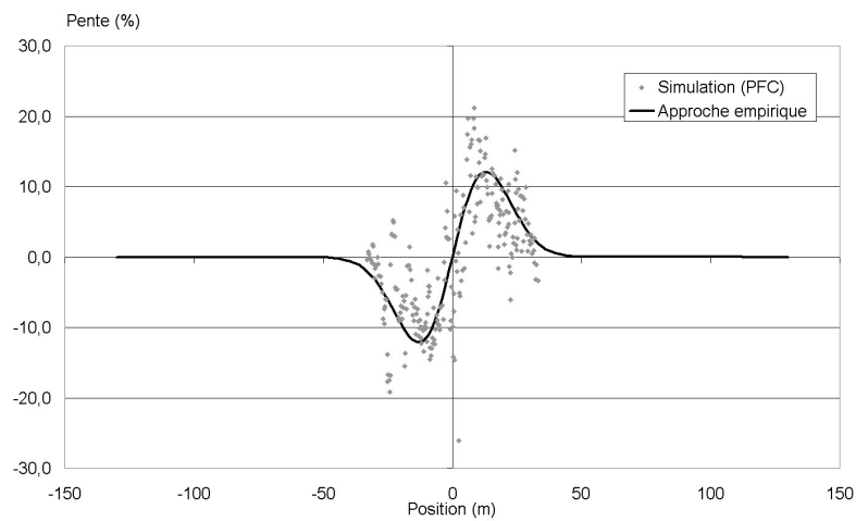
FIG. 8.11 – Tracé de la pente en surface calculée à partir des déplacements des particules
