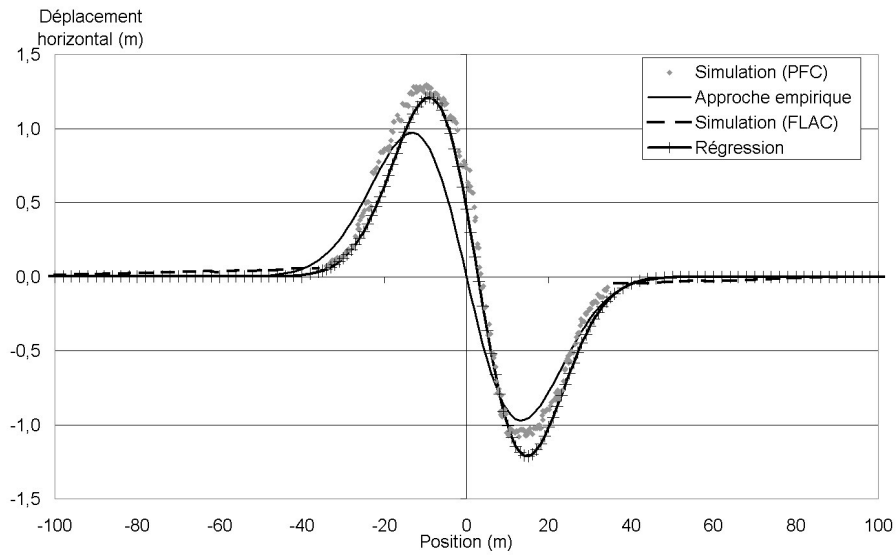
FIG. 8.10 – Déplacements horizontaux en surface pour la seconde simulation
