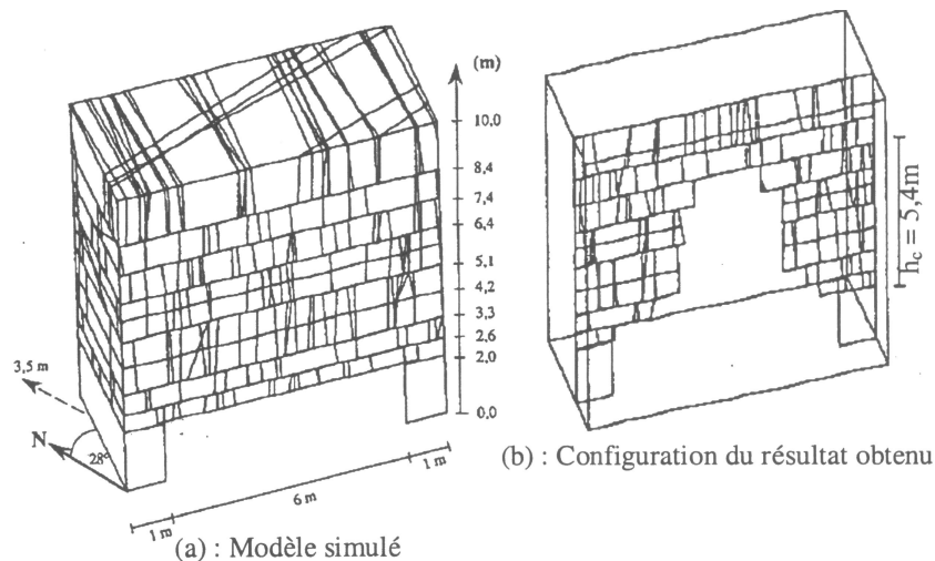
FIG. 1.11 – Massif de marbre modélisé et le réseau de fractures considérées (Asof 1991)
