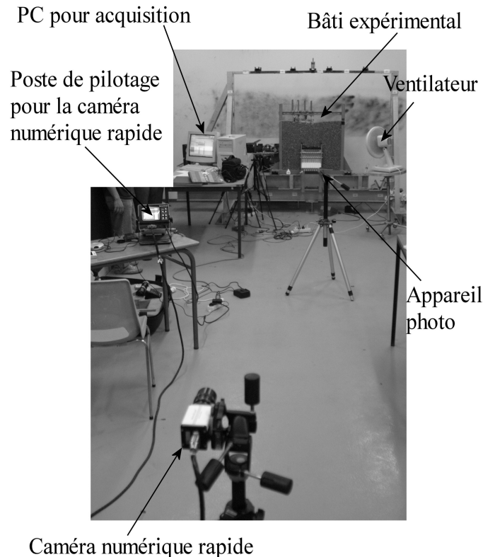
FIG. 3.4 – Vue générale du banc expérimental et de l'appareillage utilisé.
