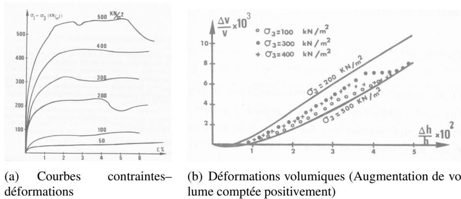
FIG. 2.5 – Essais biaxiaux sur le sol analogique sous différentes valeurs de confinement (Kastner 1982).
