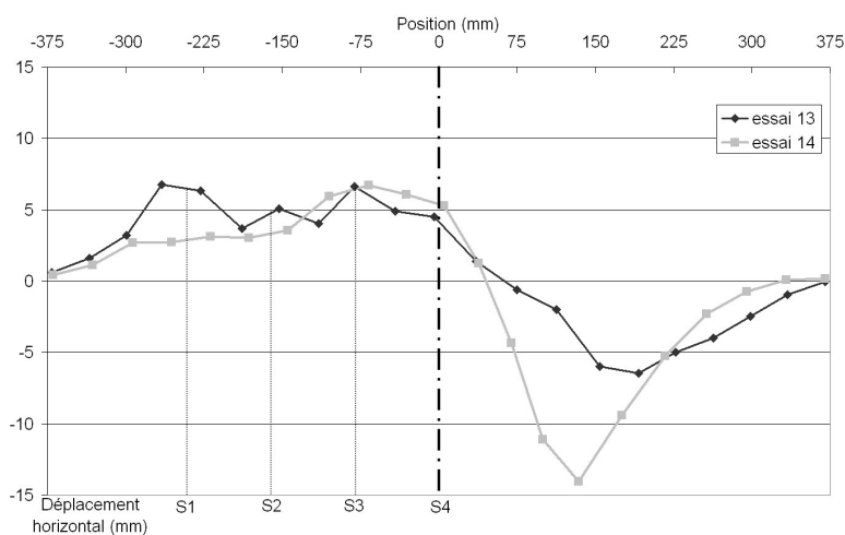
FIG. 4.39 – Déplacements horizontaux en surface – Essai 13 et 14
