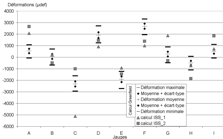
FIG. 7.26 – Déformations au sein de la structure pour les mouvements de terrain des simulations numériques en terrain vierge et en présence de la structure
