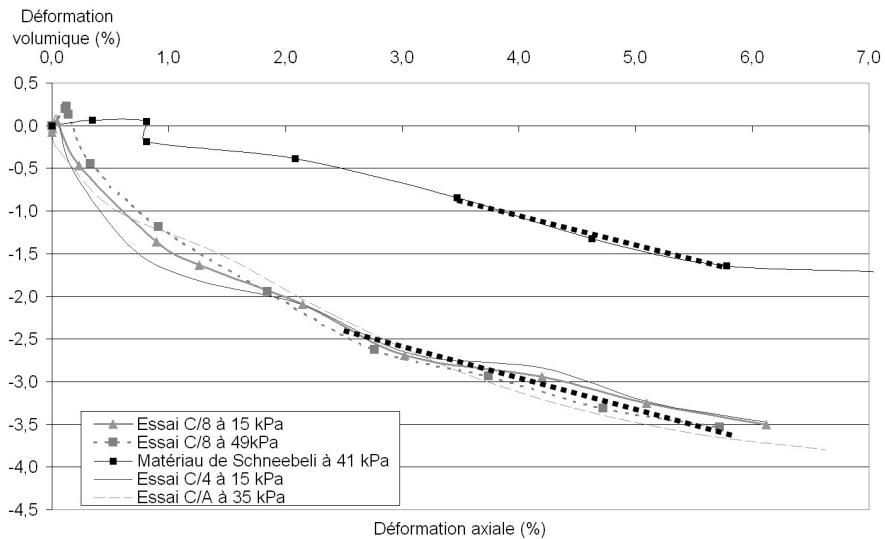
FIG. 2.25 – Déformation volumique pour deux essais avec le matériau à C/8
