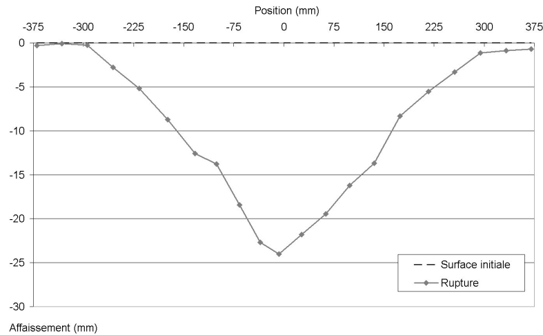
FIG. 3.41 – Cuvette d'affaissement lors de la rupture pour l'essai 9
