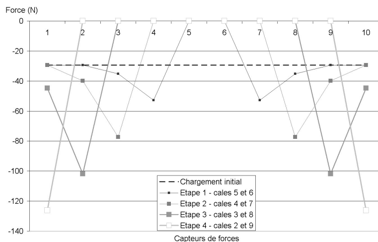
FIG. 3.48 – Evolution théorique des reports de charge sur les cales
