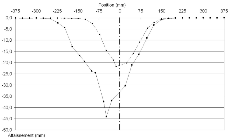
FIG. 3.11 – Cuvettes d'affaissement pour les deux étapes de rupture
