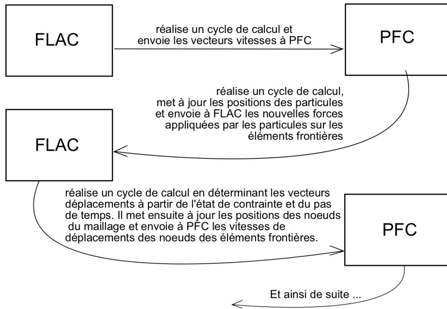
FIG. 5.8 – Présentation schématique de la réalisation d'un cycle de calcul couplé
