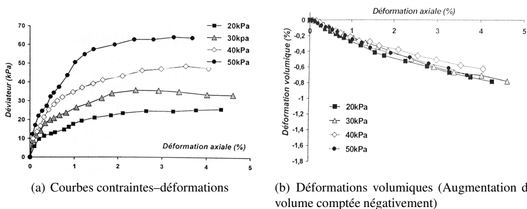
FIG. 2.7 – Résultats des essais biaxiaux de Dolzhenko (2002).
