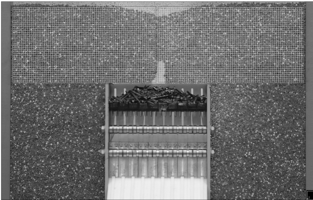
FIG. 3.9 – Illustration du maillage superposé à un cliché de l'essai
