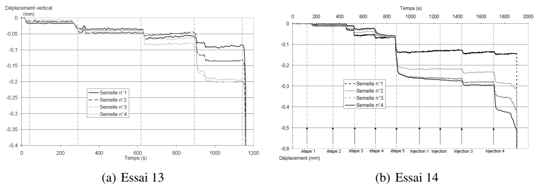
FIG. 4.45 – Déplacements des semelles par les capteurs LVDT avant la rupture
