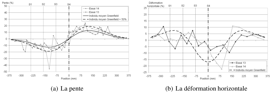
FIG. 4.48 – Evolution de la pente et de la déformation horizontale le long de la surface
