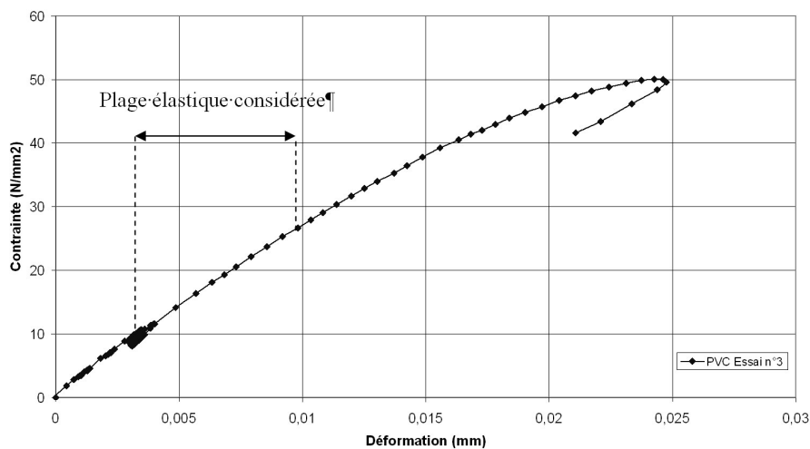
FIG. C.4 – Essai de traction simple sur le PVC
