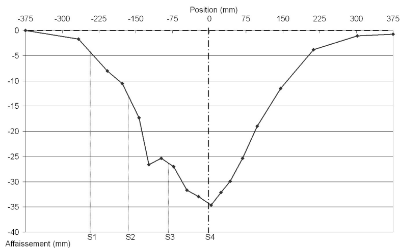
FIG. 4.30 – Cuvette d'affaissement post-rupture - Essai 14
