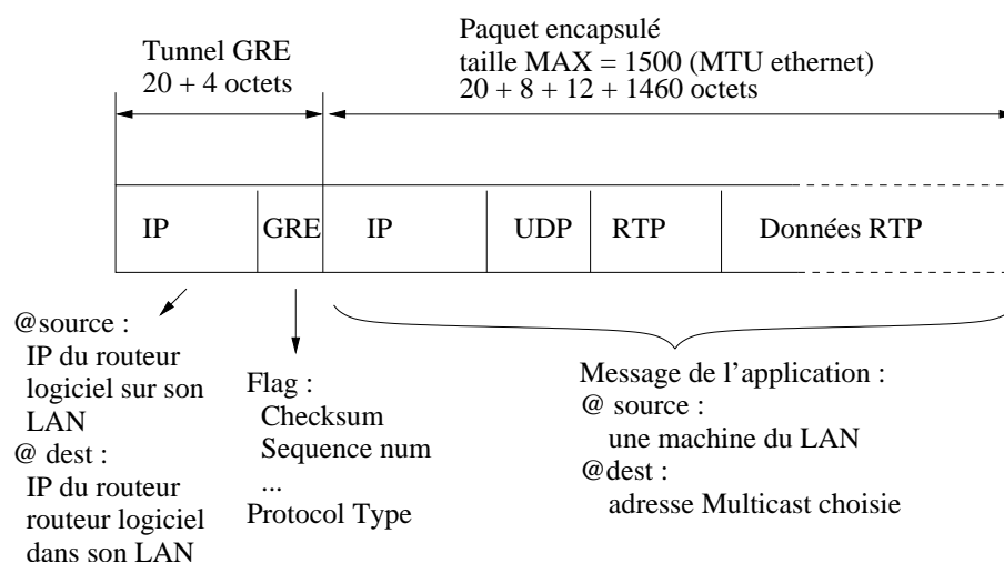
FIG. 9.3 – L'encapsulation de RTP dans un tunnel GRE
