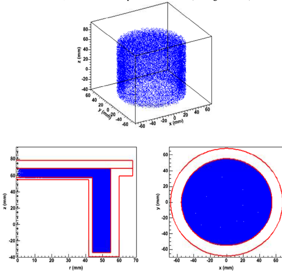
Figure 10-2 : Simulation avec Geant4 d'une source étendue en géométrie bécquer de Marinelli. En rouge sont représentées les parois du bécquer, en bleu les positions de la source générant les photons. La figure en haut est une vue en trois dimensions de la source, la figure en bas à gauche est une projection dans un plan (r, z) où seule la moitié du bécquer est représentée. La figure en bas à droite est la projection dans un plan (x, y)
