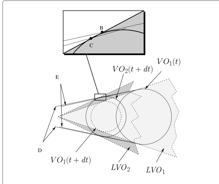
FIG. 4.23 – Erreur d'approximation pour r_B variable Afin de faciliter la compréhension du lecteur, nous nous plaçons dans le cas d'un LVO. Dans le cas nominal (rayon constant), deux VO(t) consécutifs ( VO_1(t) et VO_1(t+dt) ) admettent pour tangentes les droites E passant par les points de tangence. Il s'agit des bords de LVO_1 . Lorsque le rayon de A ou de B augmente au cours du temps, son VO(t) à l'instant t ( VO_2(t+dt) ) est plus grand que dans le cas nominal ( VO_1(t+dt) ). Les bords du VO résultant peuvent être approximés localement par les tangentes D entre VO_1(t) et VO_2(t+dt) . Cette construction implique que les droites E sont situées entre les droites D, et donc que l'approximation du VO à l'aide des points de tangence n'est pas conservative. En revanche, cette approximation englobe LVO_1 .
