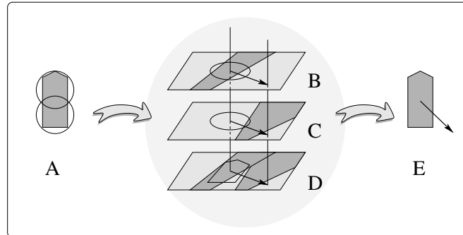
FIG. 4.1 – Méthode de fusion Le robot est ici approximé par deux robots virtuels (A). Leurs NLVO respectifs sont calculés (B et C) puis fusionnés (D) pour former une approximation du NLVO associé au robot réel. Une vitesse sûre peut alors être sélectionnée (E).
