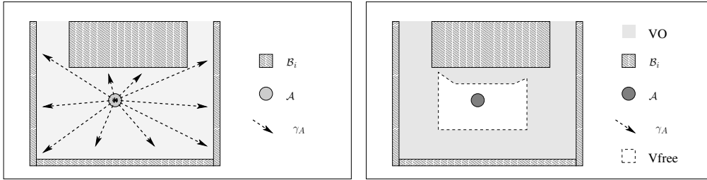
FIG. 2.6 – V_{free\Omega} = \emptyset pour TH \rightarrow \infty Bien que le robot admette des vitesses solutions qui lui permettent de sortir de la pièce modélisée, elles ne sont pas « visibles » à l'aide des VO si TH \rightarrow \infty (à gauche). En revanche, avec un TH borné, alors V_{free\Omega} \neq \emptyset . Le robot peut se déplacer.
