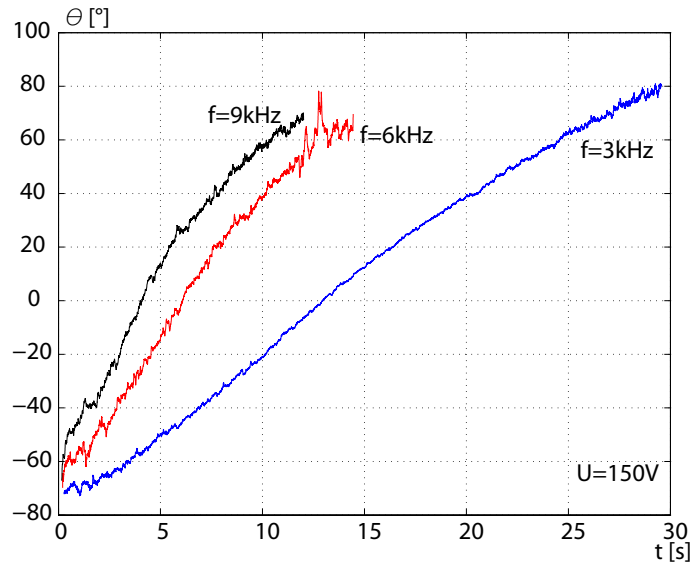
FIG. 3.28 – Mouvement du microsystème autour du tube pour trois fréquence différentes et à U = 150\text{V} .
