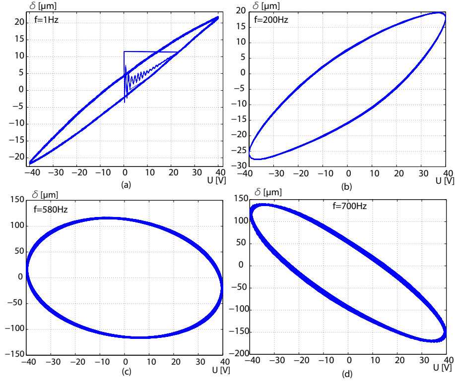
FIG. 5.11 – L’hystérésis de la poutre piézoélectrique est dynamique ( rate-dependant ).
