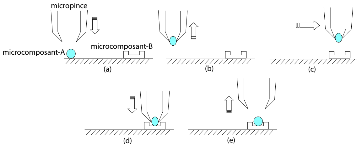
FIG. 2.1 – Microassemblage serial
