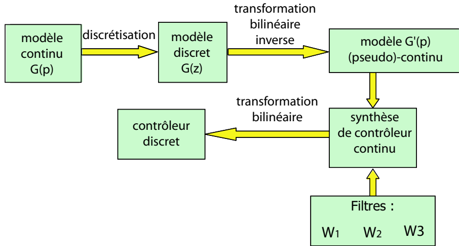
FIG. 5.39 – Les étapes de synthèse d'un correcteur discret en utilisant la transformation bilinéaire.
