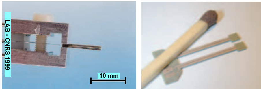
FIG. 2.7 – Une micropince à poutres piézoélectriques unimorphes [Had00] et une micropince à poutres piézoélectriques bimorphes [Agn03b].
