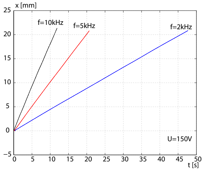
FIG. 3.25 – Mouvement du microsysteme le long du tube pour trois fréquences différentes et à U = 150\text{V} .
