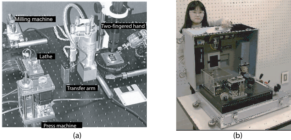
FIG. 2.15 – Premier prototype de micro-usine [Tan01]. a : les différentes stations qui composent le prototype. b : démonstration de sa portabilité.
