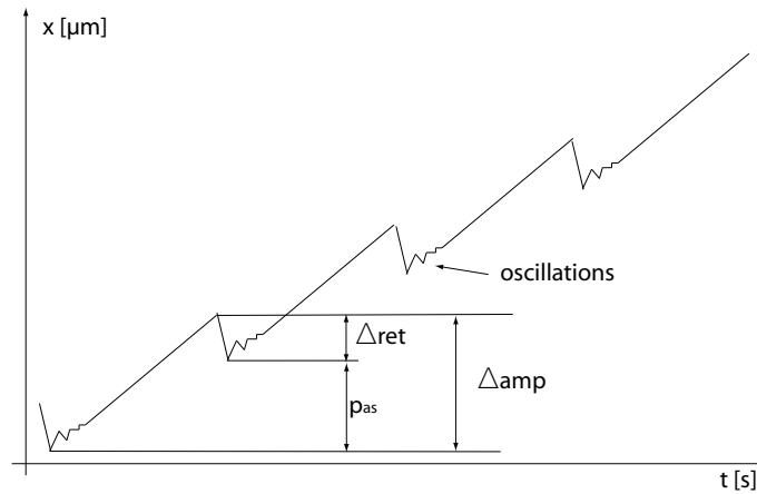
FIG. 3.12 – Evolution des mouvements inertiels.
