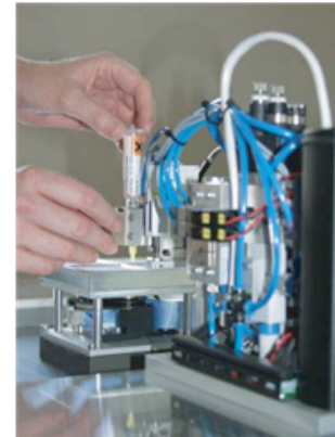
FIG. 2.19 – a : "MiniProd" composé de modules plug-and-produce [Gau04a] [Gau04b]. b : module de micromanipulation. c : module de microvissage. d : module de collage.
