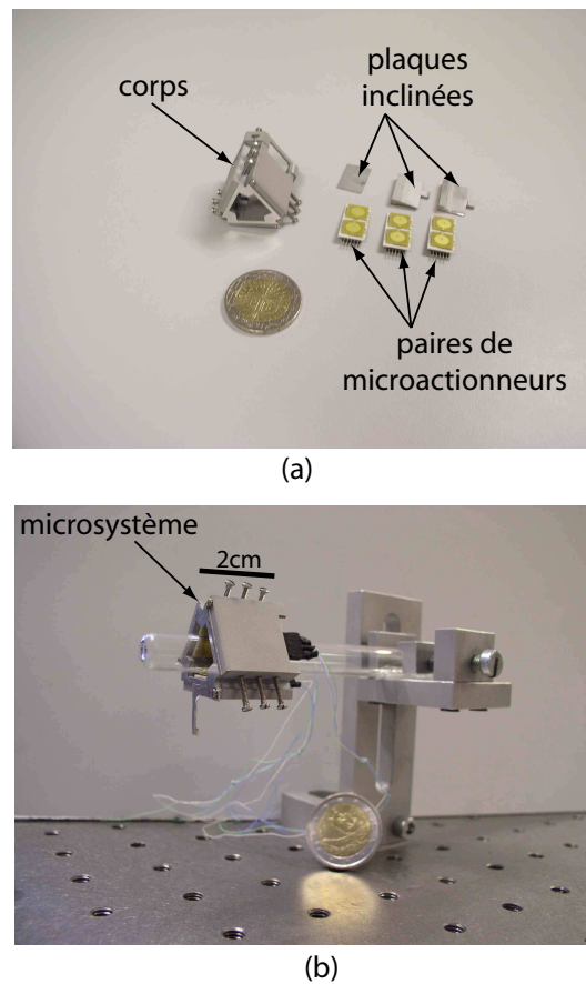
FIG. 3.22 – a : les composants du microsystème. b : le microsystème monté sur le tube.
