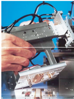
FIG. 2.19 – a : "MiniProd" composé de modules plug-and-produce [Gau04a] [Gau04b]. b : module de micromanipulation. c : module de microvissage. d : module de collage.
