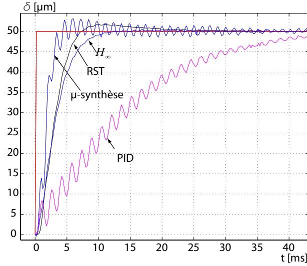
FIG. 5.44 – Résultat expérimental de la réponse en échelon.
