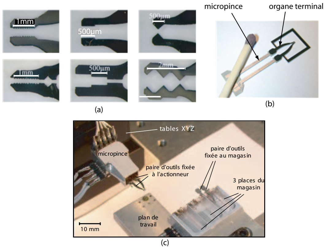
FIG. 2.13 – a et b : différents types d’organes terminaux et photographie d’une micropin équipée d’organes terminaux [Agn03b]. c : un système de changeur d’organe terminal [Clé02].
