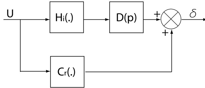
FIG. 5.54 – Schéma systématique de l'hystérésis statique, de la dérive et de la partie dynamique.
