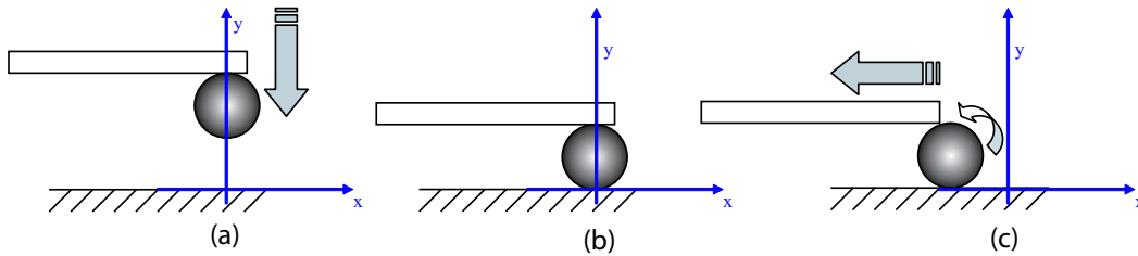
FIG. 5.4 – Dépose par roulement [Dio04].
