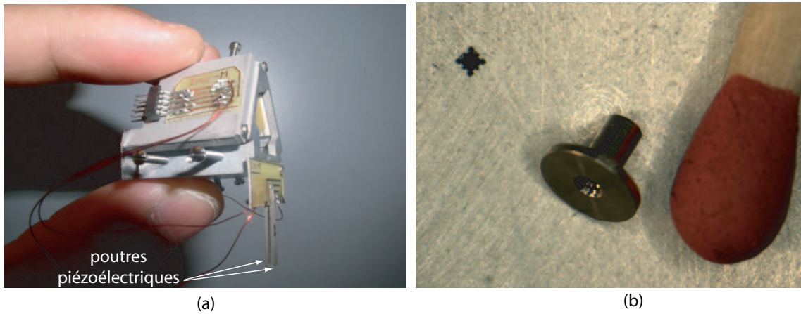
FIG. 6.9 – a : une micropince à deux poutres piézoélectriques sur le microsystème 2ddl. b : un mini-essieu.
