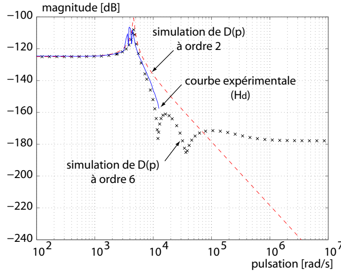
FIG. 5.16 – Magnitudes de H_i (trait continu), de D(p) avec l'équation (5.10) (trait caché) et de D(p) avec l'équation (5.11) (trait-x).
