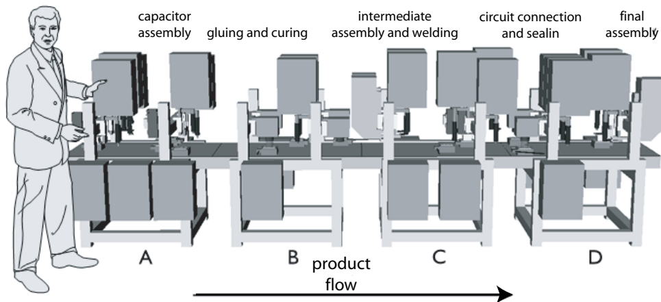
FIG. 2.27 – Une mini-usine [Hol98].
