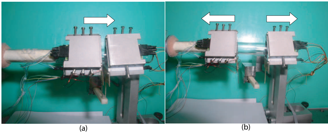
FIG. 6.16 – a : arrivé au lieu de dépose. b : écartement des microsystèmes.
