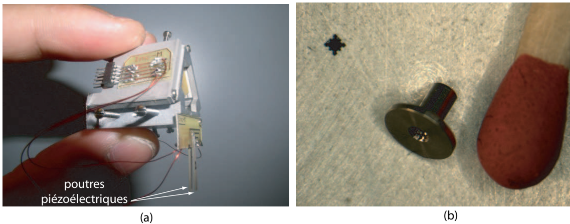
FIG. 6.9 – a : une micropince à deux poutres piézoélectriques sur le microsysteme 2ddl. b : un mini-essieu.
