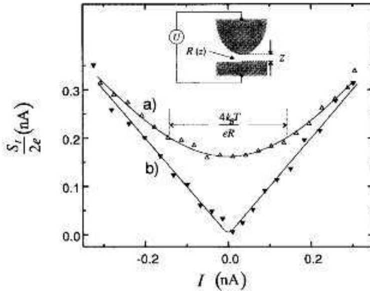
FIG. 1.8 – Bruit en fonction du courant. en haut \Theta = 300K et R \simeq 0.32G\Omega ; en bas \Theta = 77K et R \simeq 2.7G\Omega . Les traits pleins sont les estimations théoriques [38].
