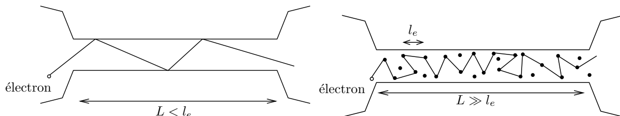
FIG. 1.2 – A gauche : schéma d'un conducteur mésoscopique ballistique, la longueur de l'échantillon est inférieure à l_e et les électrons subissent peu de chocs élastiques. A droite : schéma d'un conducteur diffusif, les électrons subissent beaucoup de chocs élastiques. Dans les deux cas, L est très inférieure à la longueur de cohérence l_\phi .
