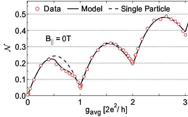
FIG. 1.7 – Bruit en fonction de la conductance. Le bruit s’annule lorsque la conductance est un multiple de 2e^2/h . \mathcal{N} est le bruit grenaille lorsque les effet thermiques sont pris en compte dans un point contact[34].
