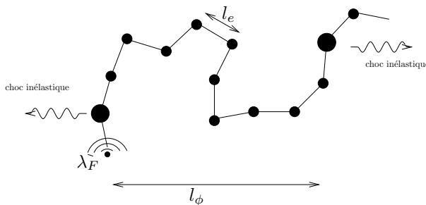
FIG. 1.1 – Schéma du parcours d'un électron de conduction dans un conducteur : l'électron subit des chocs élastiques contre des impuretés, ces chocs sont distants en moyenne de l_e = v_F \tau_e et il subit des chocs inélastiques. L'intervalle de temps entre deux chocs inélastiques est \tau_{in} et la distance moyenne l_{in} = \sqrt{D\tau_{in}} avec D le coefficient de diffusion.
