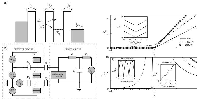
FIG. 5.1 – Aguado et Kouwenhoven [72] ont proposé de mesurer le bruit non-symétrisé à l'aide d'un circuit capacitif. S_- est mesuré sur les fréquences négatives et S_+ sur les fréquences positives. On voit apparaître une nette différence entre ces deux régimes de bruit pour un double point contact. Le courant fait apparaître également deux régimes.
