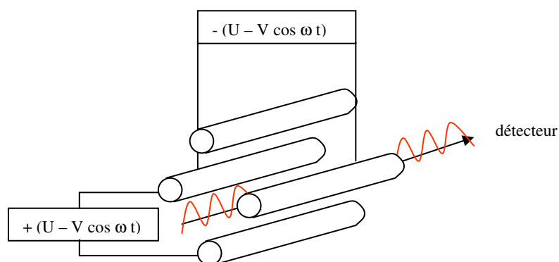
Figure 3 : Analyseur quadripolaire.
