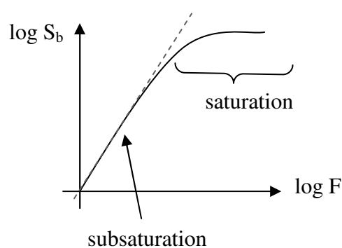
Figure III.5 : Illustration des domaines de subsaturation et de saturation de l'isotherme de Freundlich.
