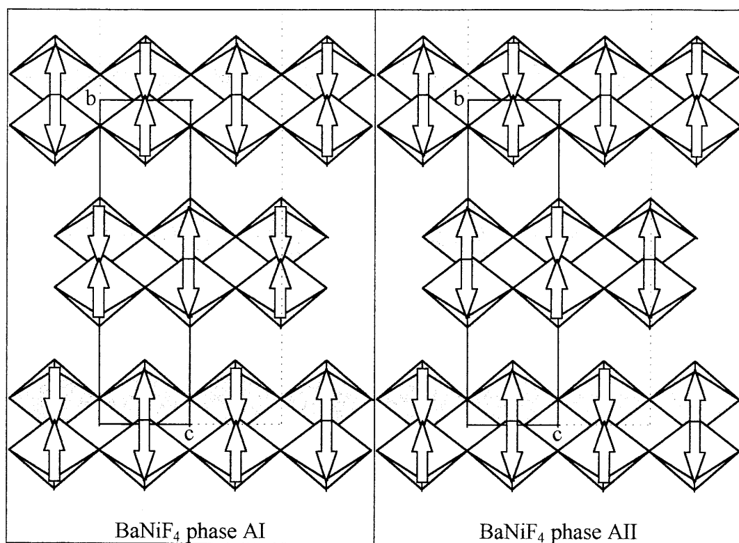
Figure 36 - Structures magnétiques de \text{BaNiF}_4
