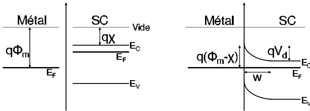
FIG. 7.3: Diagrammes de bandes d'une mise en contact métal/semiconducteur dopé n.
