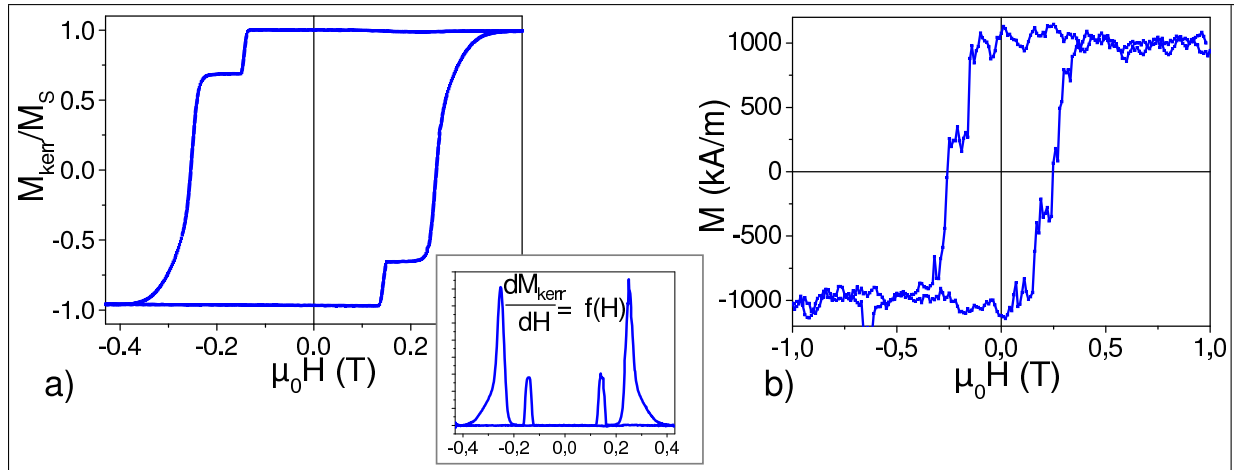
FIG. 4.2: Cycle d'aimantation majeur d'une structure \text{FePt}_{10\text{nm}}/\text{MgO}_{3\text{nm}}/\text{FePt}_{5\text{nm}} , mesuré par Effet Kerr Polaire (figure a) et VSM (figure b)), H étant perpendiculaire au plan des couches. Par effet Kerr Polaire, le signal mesuré ( M_{\text{kerr}} ) ne correspond pas exactement à l'aimantation de la structure, le signal de la couche enterrée étant plus faible que le signal de la couche supérieure.
