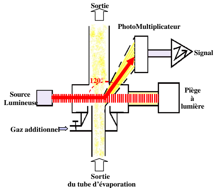
Figure I-35: Schéma de la cellule de détection du DEDL (Sedex55).
