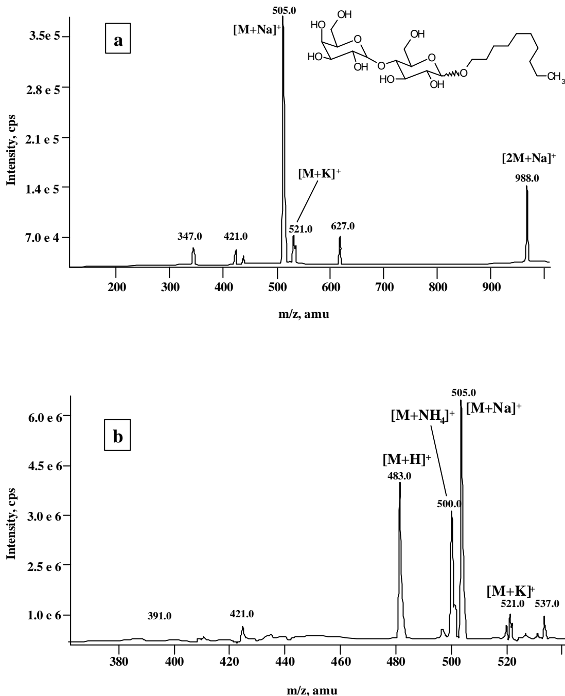
Figure 16: Spectre de masse en mode positif du décyl-lactoside ( M=482 ). a) infusion à 5 \mu\text{l}/\text{min} dans un mélange acétonitrile-eau (75-25). Le pic à m/z=505 ( M+23 ) correspond à l'ion adduit [M+\text{Na}]^+ . La masse moléculaire est confirmée par la présence d'un adduit [M+\text{K}]^+ à m/z=521 ( M+39 ) et la présence d'un ion dimère [2M+\text{Na}]^+ à m/z=988 . b) En acidifiant la solution avec \text{HCOOH} , l'ion [M+\text{H}]^+ apparaît sur le spectre ainsi que l'ion [M+\text{NH}_4]^+ vraisemblablement à cause de trace d'ammoniac sur la contre-électrode ou sur le capillaire. Source: IonSpray (+5,7kV), orifice (60V), Anneau (400V). [P. Chaimbault, C. Elfakir, M. Lafosse, J. High Resol. Chromatogr. 22 (1999) 188].
