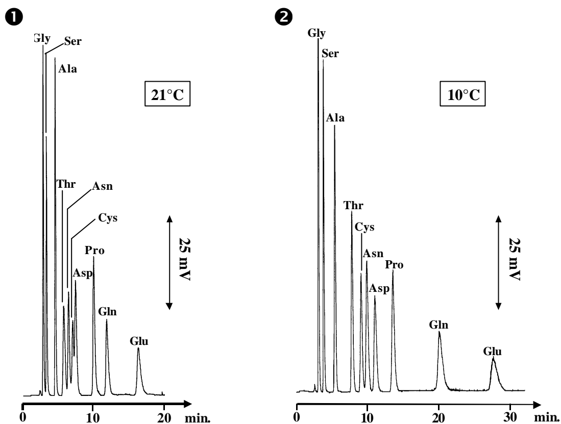
Figure III-12: Analyse isocratique CPL-DEDL des 10 acides aminés élus les premiers sur PGC. Phase mobile: solution aqueuse de NFPA (20mM). Colonne Hypercarb 5µm (100x2,1 D.I), Débit:200µl/min. Température de la colonne : ① 21°C ② 10°C. Standards à 100 mg/l. Volume injecté: 3µl.
