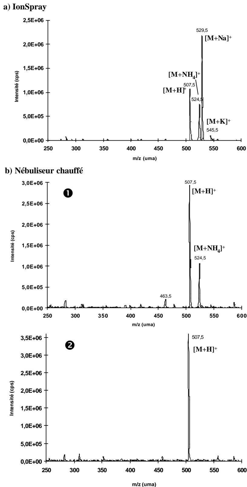
Figure I9: Spectres de masse de l'hexaéthylène glycol monohexadécylether ( C_{16}EO_6 ). a) IonSpray (5,7kV) et b) nébuliseur chauffé ( 3\mu A , 400^\circ C ). On notera en b- 1 la présence de l'adduit ammonium qui disparaît en b- 2 après nettoyage de la contre-électrode et de l'orifice. Concentration: 100mg/l, dilué par 10 pour l'ionisation avec le nébuliseur chauffé. Solvant: méthanol-eau- HCOOH 95/5/0,5 (v/v).
