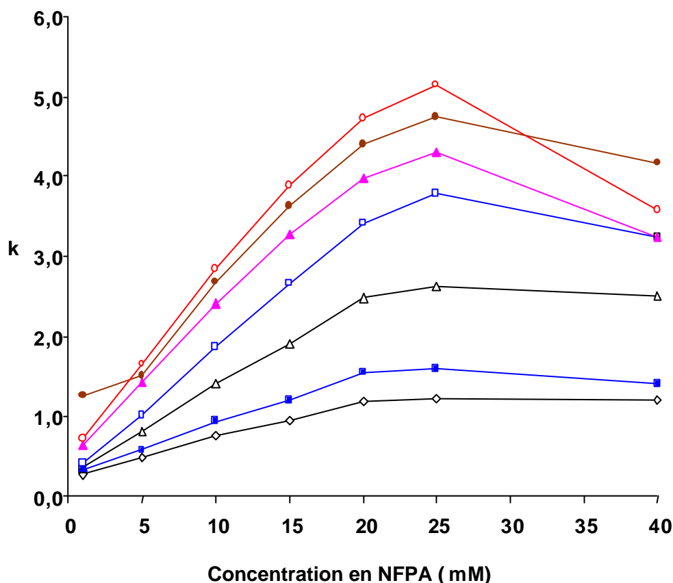
Figure III-11: Influence de la concentration en acide nonafluoropentanoïque (NFPA) sur la rétention des 7 acides aminés protéiques non dérivés élués les premiers sur PGC. Gly ( \diamond ), Ser ( \blacksquare ), Ala ( \Delta ), Thr ( \square ), Asn ( \blacktriangle ), Cys ( \bullet ), Asp ( \circ ).
