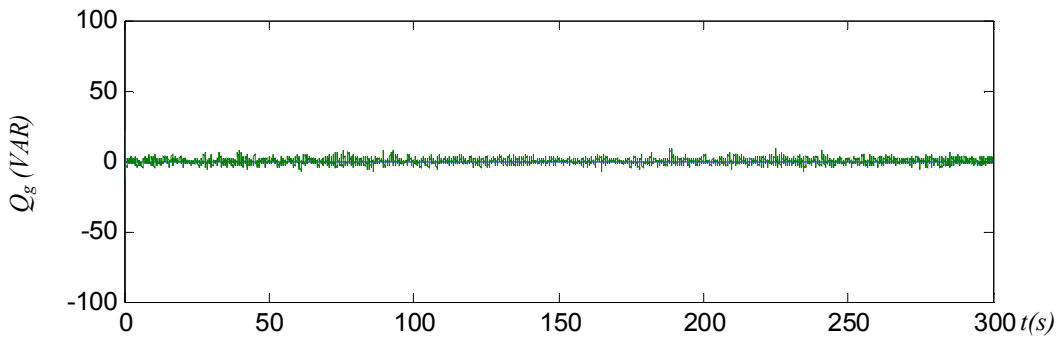
Fig. 4.12b: Puissance réactive transitée au réseau Q_{ref}=0 .
