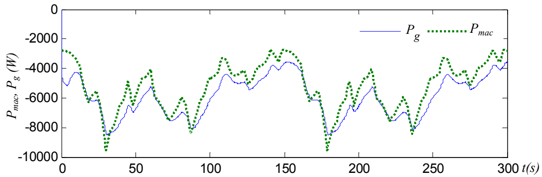
Fig. 4.12a: Puissance éolienne et puissance active transitée au réseau.
