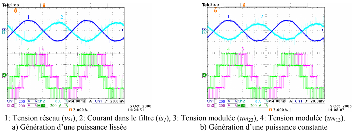
Fig. 2.45: Résultats expérimentaux pour la génération d'une puissance (lissée (a) et constante (b)) en utilisant un onduleur NPC à trois niveaux et un stockage avec une inertie de 0,2\text{kg m}^2 .
