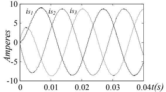
Fig. 1.29b : Courant dans la charge
