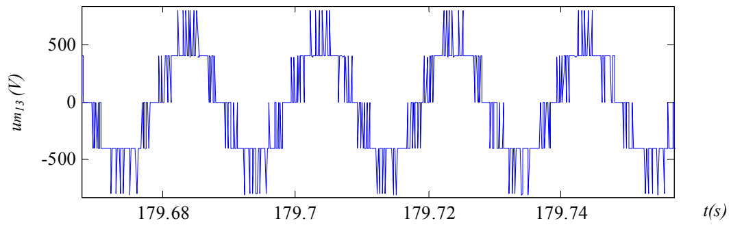
Fig. 2.53c: Tension modulée um_{13} côté réseau.
