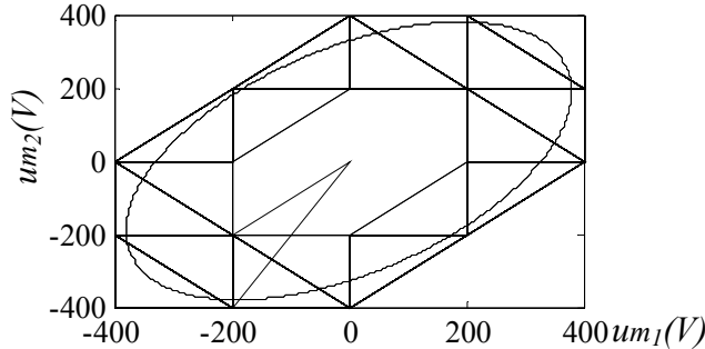
Fig.1.29a: Tensions de référence et les vecteurs utilisés.
