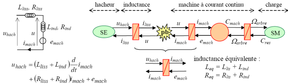
Fig. A.13: Exemple de la REM avec deux bobines en série.
