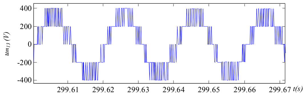
Fig. 2.39c: Tension modulée um_{13} .
