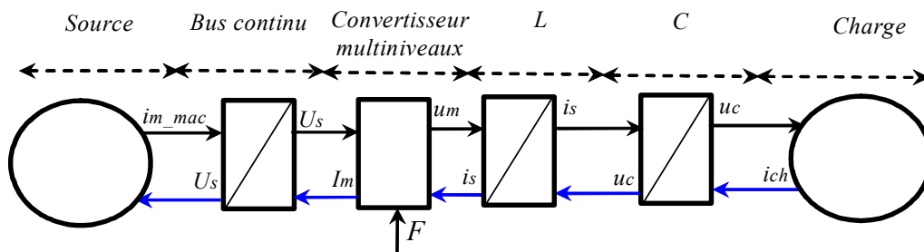
Fig. 1.2: R. E. M. du modèle de l'onduleur.
