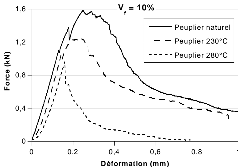
Figure 90 - Influence de la température de rétificaion sur l'allure des courbes de flexion
