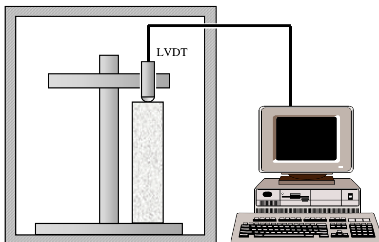
Figure 96 - Principe de mesure des variations dimensionnelles
