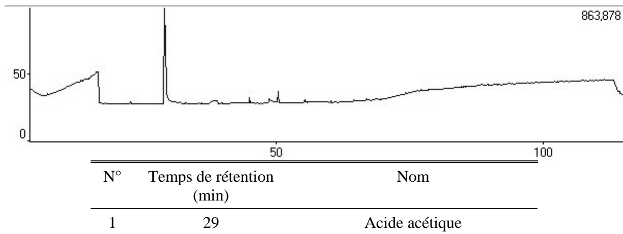
Figure 24 - Résultats de l'analyse CPG/SM des extraits aqueux de peuplier naturel
