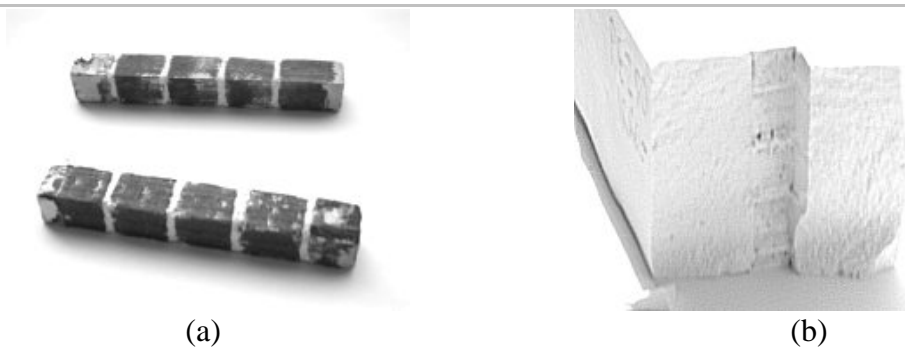
Figure 49 - Après l'essai : (a) échantillon de bois. (b) logement du bois dans l'échantillon de matrice
