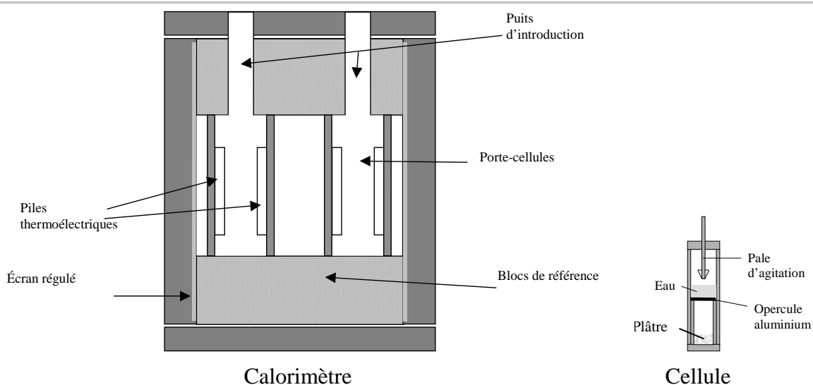
Figure 55 - Schéma du calorimètre
