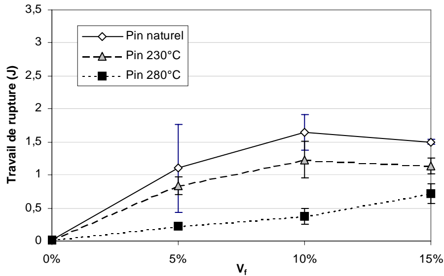
Figure 86 - Influence de la température de traitement sur le travail de rupture des composites contenant du pin défibré
