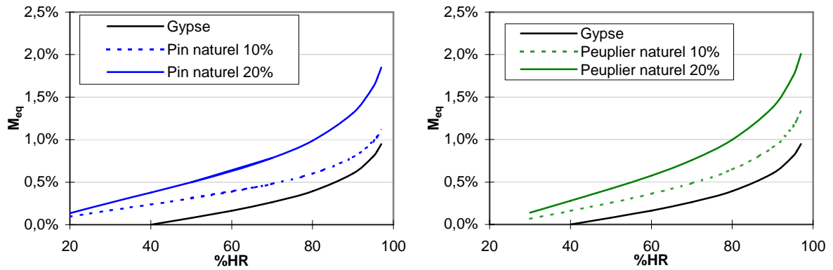
Figure 102 - Isothermes de reprise d'humidité des composites de pin sylvestre et de peuplier naturel – Morphologie : broyats - Température : 23°C
