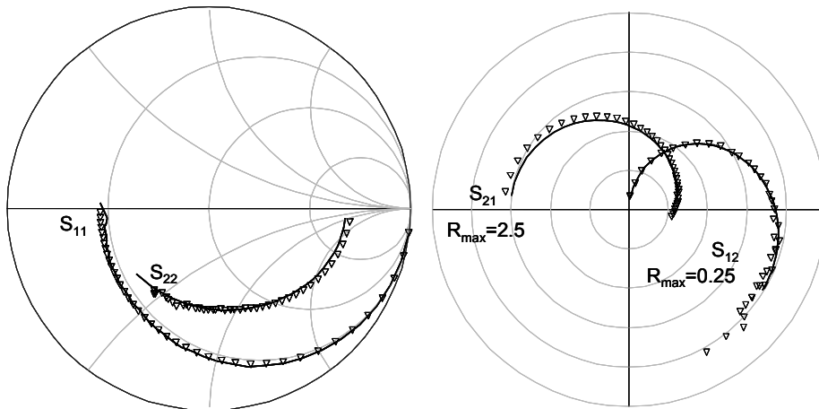
Fig 3.23b Accord simulation — mesures \Delta pour V_{GS} = 0 V et V_{DS} = 10 V Mesures effectuées de 40 MHz à 40 GHz (HEMT 2 \times 0.25 \times 75 \mu m^2 )
