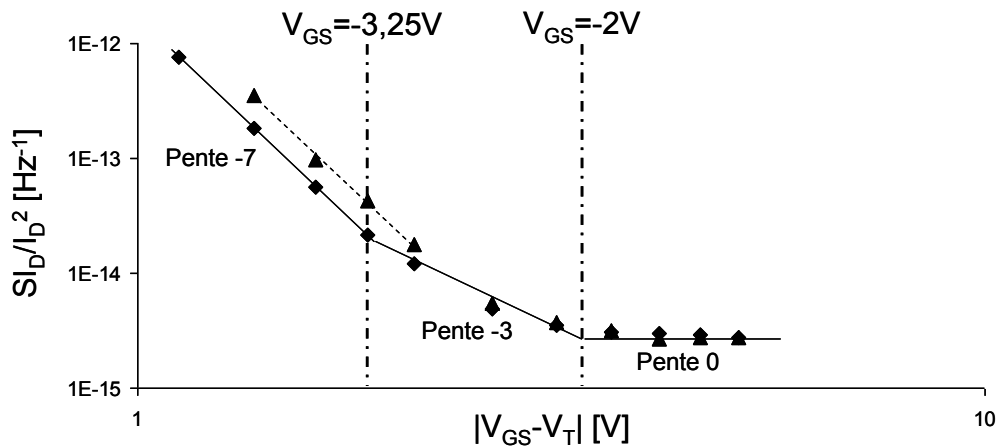
Fig 2.12 Représentation de Peransin du HEMT AlGaIn/GaN 0.15*2*50 \mu\text{m}^2 à 1kHz
