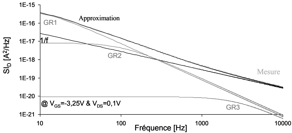
Fig 2.11 Spectre de bruit BF en régime ohmique HEMT AlGaIn/GaN 0.15*2*50 \mu\text{m}^2
