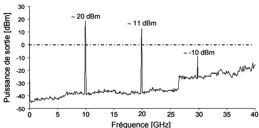
Figure 3.40 Mesure des harmoniques de l'oscillateur.
