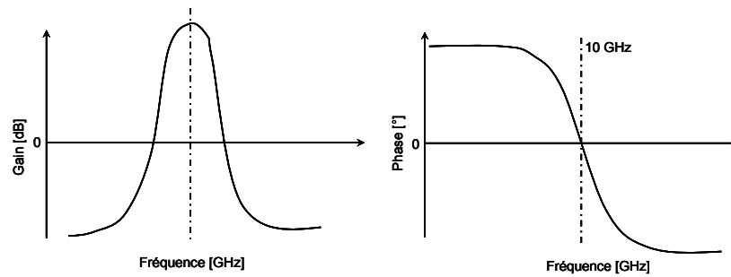
Fig 3.31 Condition à réaliser avec l'OscTest. (solution unique de 0 < \text{fréquence} \leq F_{\max} )
