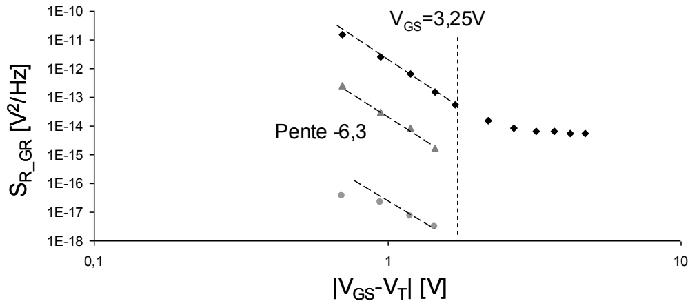
Fig 2.15 Evolution de l'amplitude du bruit des centres de G-R en fonction de V_G^*
