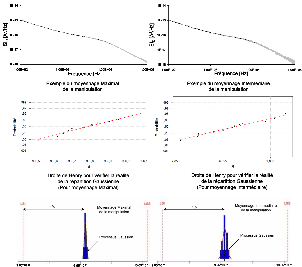
Fig 2.7a Etude de la répartition des valeurs de B pour des extractions avec différentes conditions initiales. (Moyennage maximal du banc)
