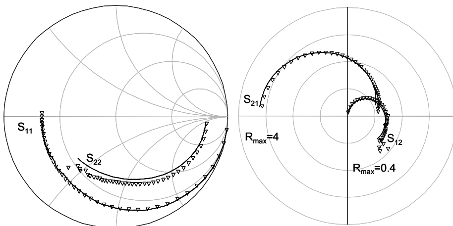
Fig 3.23c Accord simulation — mesures \Delta pour V_{GS} = -4 V et V_{DS} = 10 V Mesures effectuées de 40 MHz à 40 GHz (HEMT 2 \times 0.25 \times 75 \mu m^2 )
