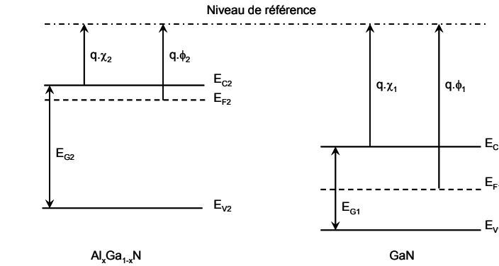
a) Schéma des bandes d'énergie des deux matériaux séparés.
