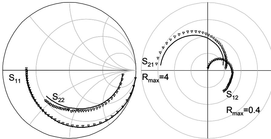
Fig 3.23a Accord simulation — mesures \Delta pour V_{GS} = -3 V et V_{DS} = 10 V Mesures effectuées de 40 MHz à 40 GHz (HEMT 2 \times 0.25 \times 75 \mu m^2 )
