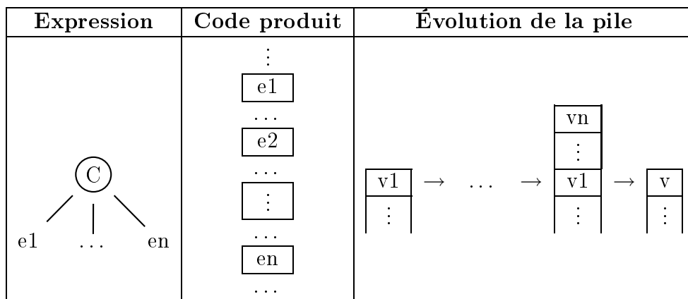
FIG. 1.11 – Compilation d'une expression Caml
