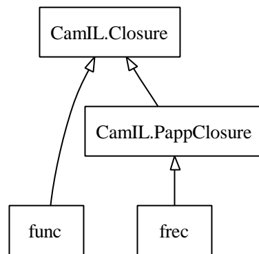
FIG. 3.2 – Hiérarchie des fermetures
