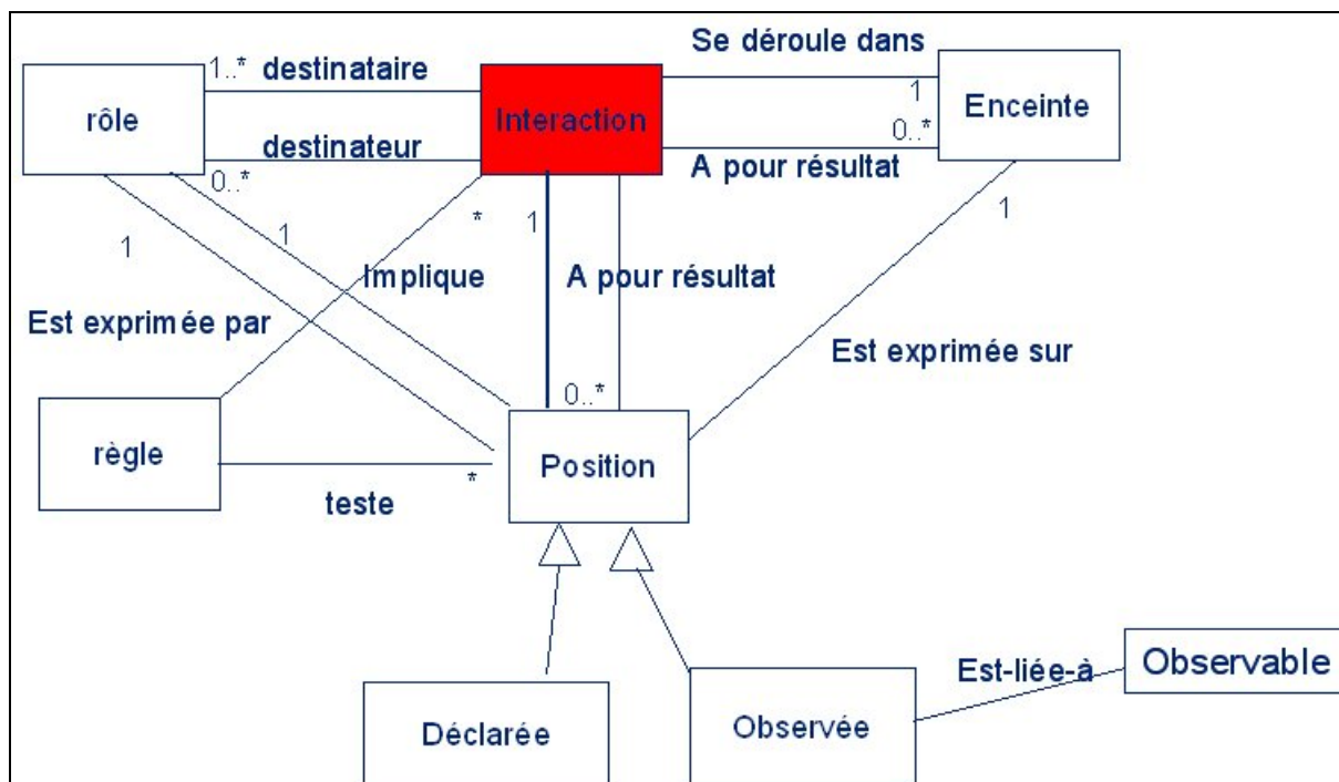
Figure 4-2. Schéma du métamodèle LDL (Martel et al. 2004)
