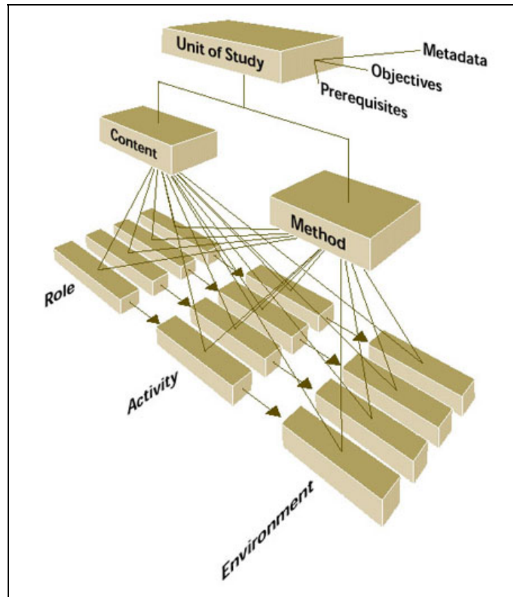
Figure 2-4. Schéma simplifié du modèle EML (Educational Modeling Language)
