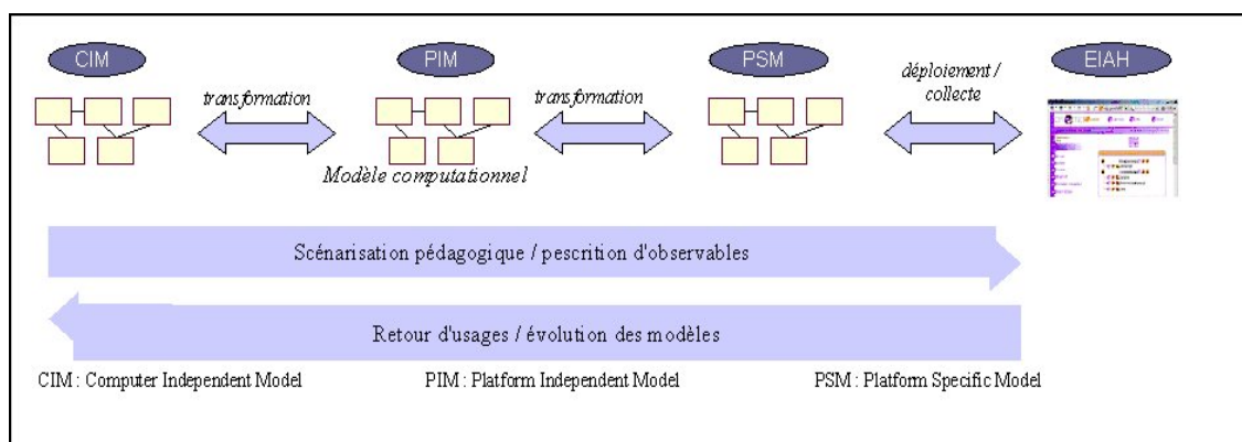
Figure 4-3. Chaîne de transformation des modèles à partir de l'IDM (Christophe Choquet 2005)
