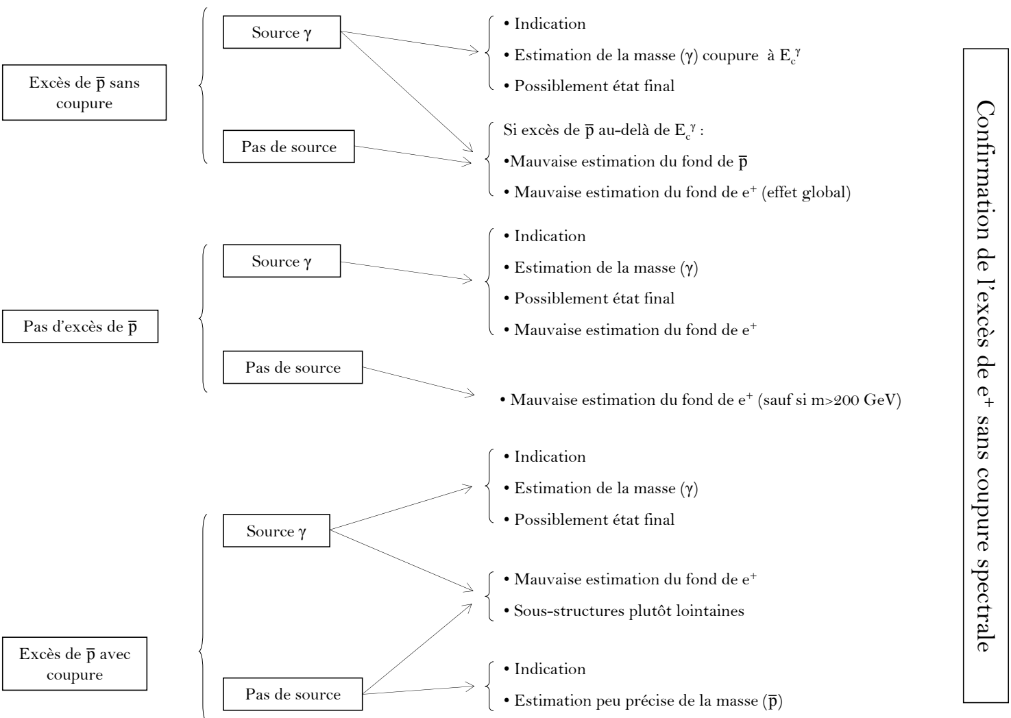
FIG. 11.29 – Différents scénarios possibles dans le cas de la confirmation de l'excès de positons sans observation de coupure dans le spectre.
