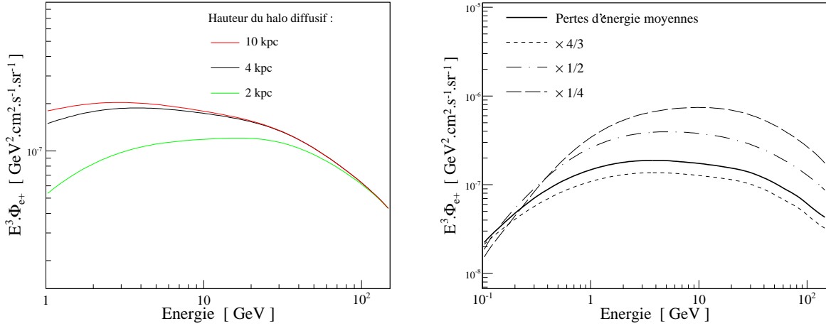
FIG. 9.16 – Influences de la modification de la hauteur de la zone diffusive et du taux de perte d'énergie sur le flux de positons.
