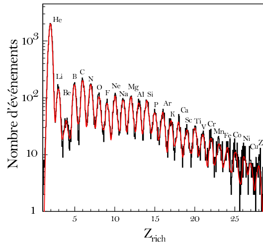
FIG. 5.6 – Séparation des charges obtenue en test faisceau (adapté de [163]).
