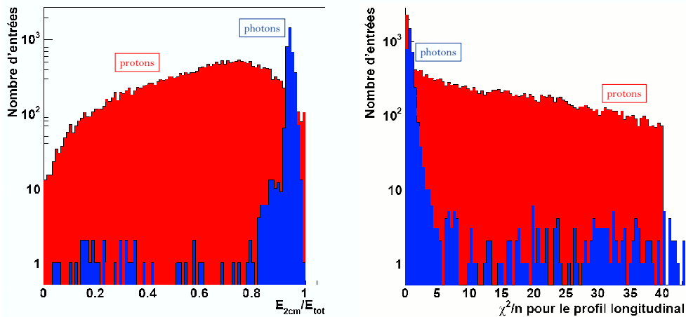
FIG. 11.13 – Variables discriminantes pour la séparation protons/photons : fraction d'énergie dans 2cm autour de l'axe de la gerbe (à gauche) et \chi^2 de l'ajustement longitudinal (à droite) [170].
