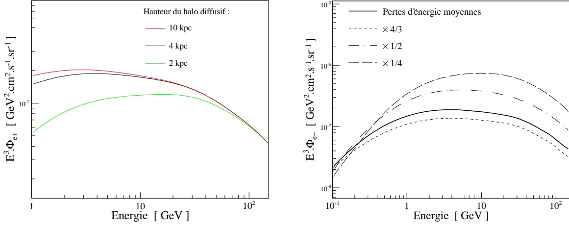
FIG. 9.16 – Influences de la modification de la hauteur de la zone diffuse et du taux de perte d'énergie sur le flux de positons.
