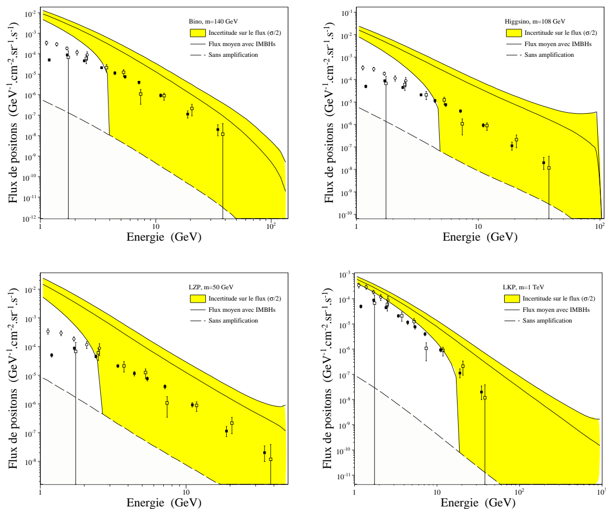
FIG. 10.10 – Flux exotiques de positons dans quatre modèles de physique des particules (en haut : en supersymétrie, en bas : en dimensions supplémentaires) et comparaison aux mesures actuelles.
