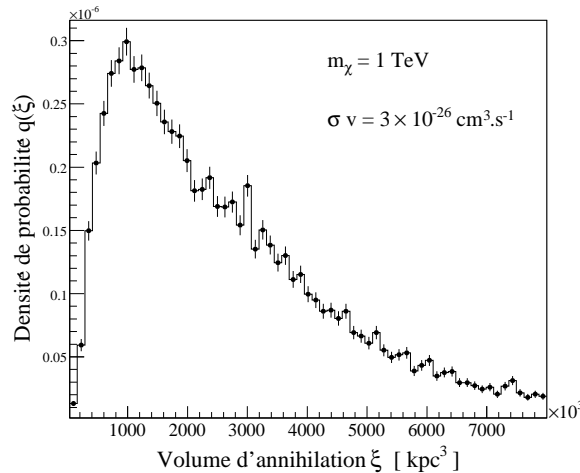
FIG. 10.5 – Densit\u00e9 de probabilit\u00e9 pour \xi dans le sc\u00e9nario B.
