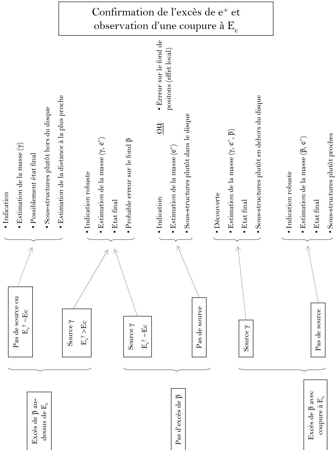
FIG. 11.28 – Différents scénarios possibles dans le cas de la confirmation de l'excès de positons accompagnée de l'observation d'une coupure dans le spectre.
