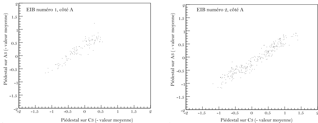
FIG. 6.10 – Corrélations des fluctuations des piédestaux d'un côté à l'autre du Écal (voir le texte).
