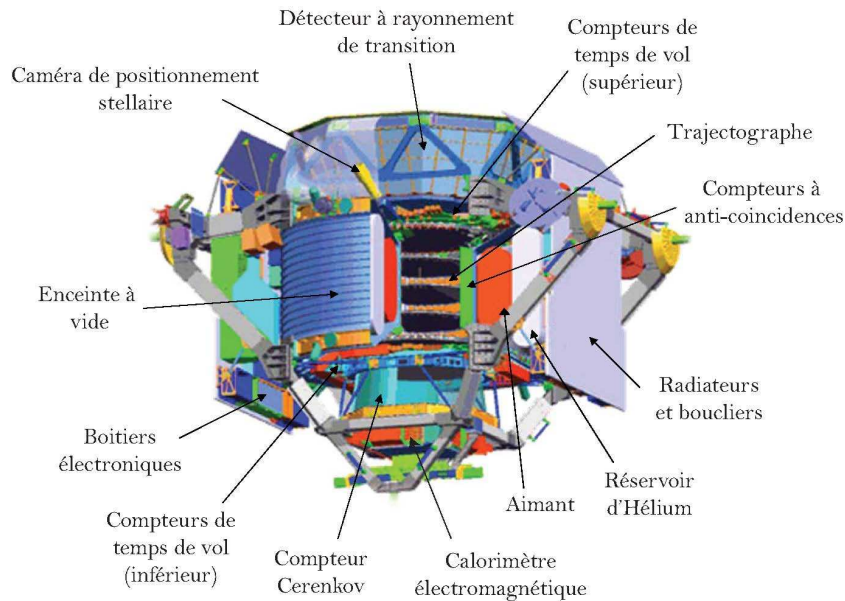
FIG. 5.1 – Le détecteur AMS02 et ses sous-systèmes.
