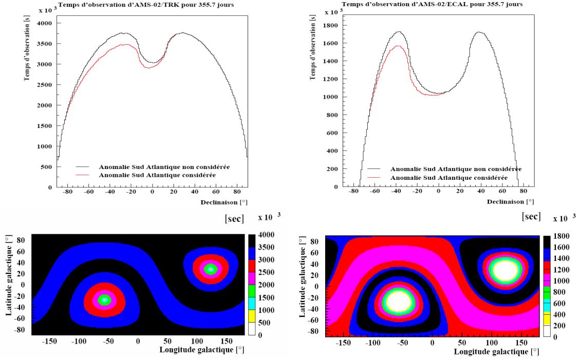
FIG. 11.17 – Cartes d’observation du ciel en \gamma par AMS02 pour le mode conversion à gauche et direct à droite [170].
