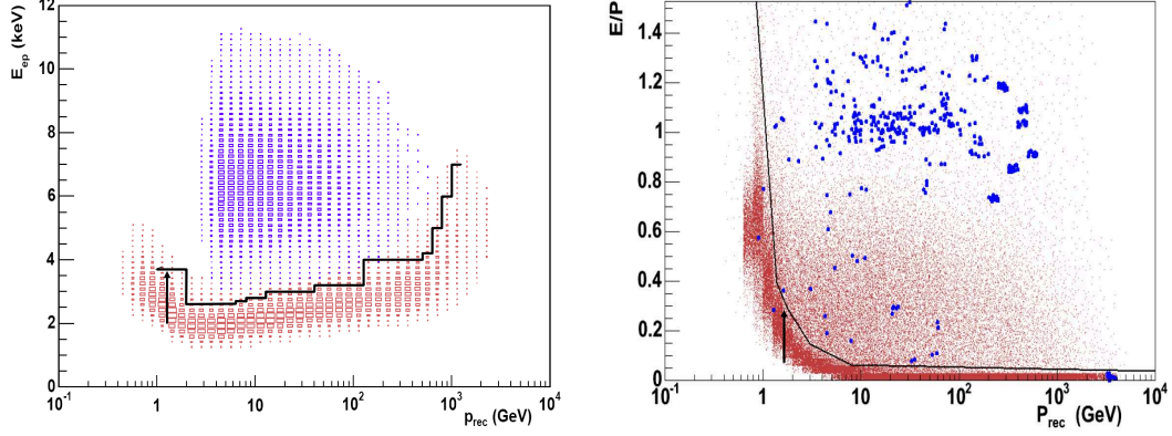
FIG. 11.3 – À gauche : sélection sur la valeur de l'énergie moyenne déposée dans le TRD. À droite : coupure sur le rapport E/p [260].
