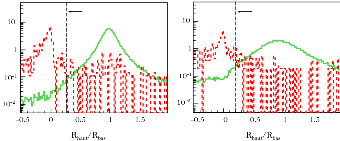
FIG. 11.1 – Distributions du rapport \mathcal{R}_{haut}/\mathcal{R}_{bas} pour des protons bons (vert plein) et négatifs (pointillé rouges) dans deux intervalles d'énergie : 25-80 GeV à gauche et 80-250 GeV à droite [260].
