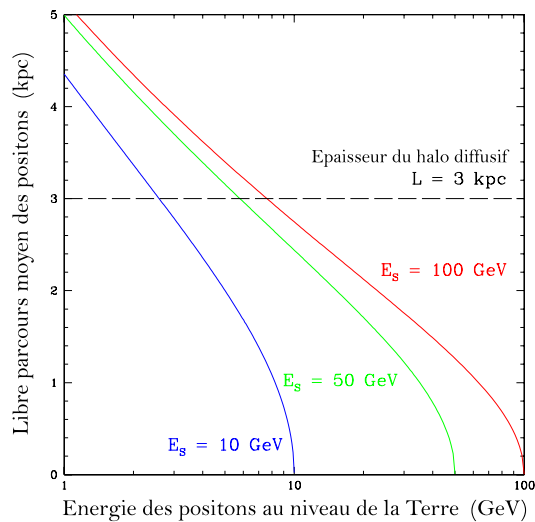
FIG. 10.2 – Libre parcours moyen d'un positron dans la voie lactée, en fonction de son énergie à la source, et à la détection (adapté de [244]).
