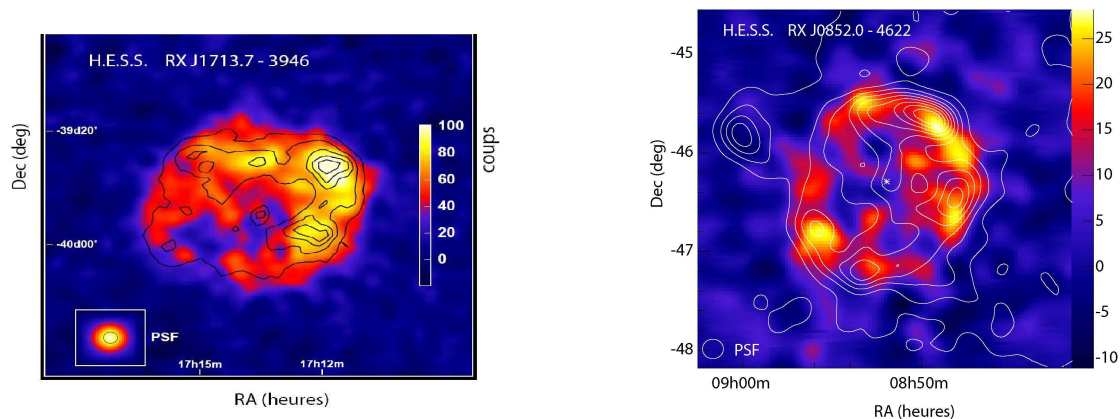
FIG. 4.2 – Images obtenues par le réseau de télescopes H.E.S.S. des restes de supernovae RXJ1713 [119] et RXJ0852 [120].
