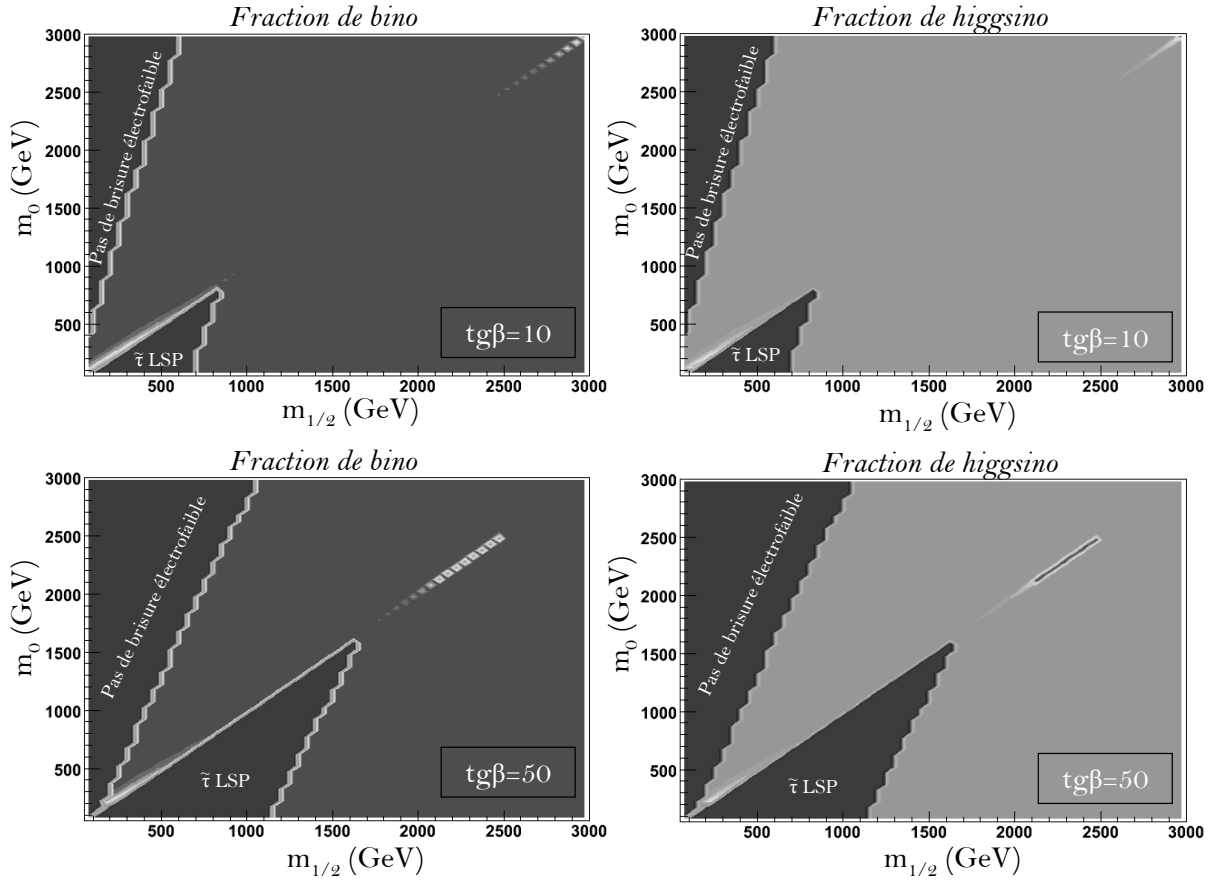
FIG. 3.3 – Contenu en champs de la LSP dans mSUGRA pour \mu > 0 , tg\beta = 10 (en haut) et tg\beta = 50 (en bas), dans le plan m_0 - m_{1/2} .
