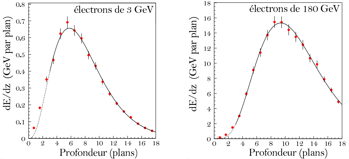
FIG. 5.9 – Profils longitudinaux de perte d'énergie dans le Ecal pour des électrons de 3 et 180 \text{ GeV} [170].
