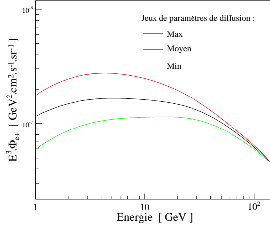
FIG. 9.17 – Flux de positons obtenus pour les jeux de paramètres conduisant aux flux extrémaux et moyen.
