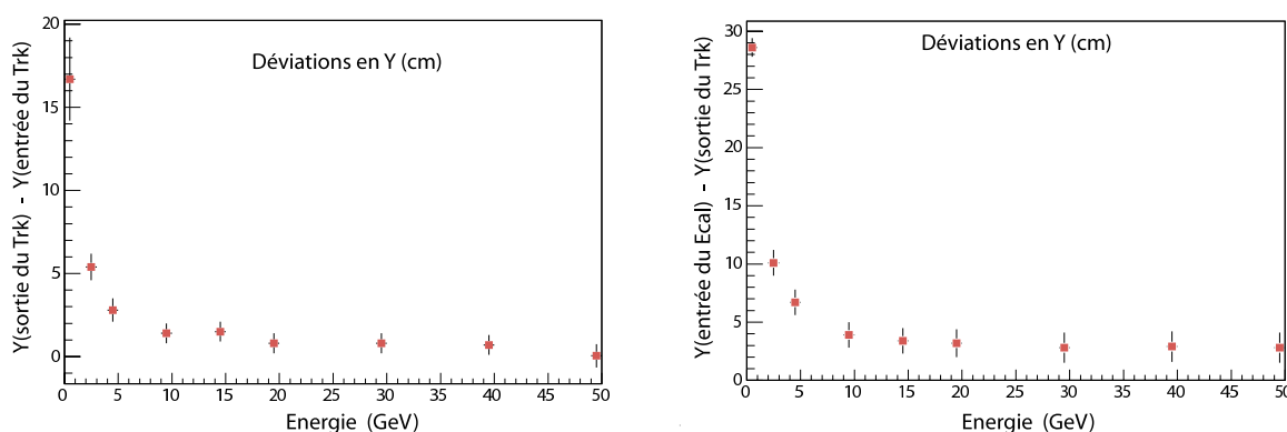
FIG. 7.12 – Déviation globale des électrons dans AMS-02.
