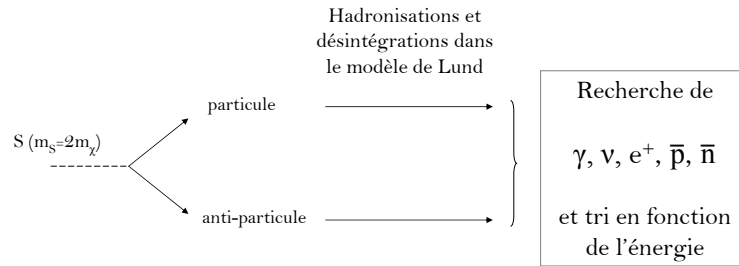
FIG. 9.3 – Principe de la génération des spectres de fragmentation dans PYTHIA.
