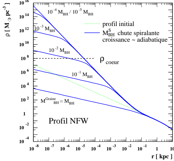
FIG. 8.2 – Modification du profil NFW en fonction de la masse de la graine excentrée ( M_{BH}^{Graine} en fonction de la masse finale M_{BH} ).
