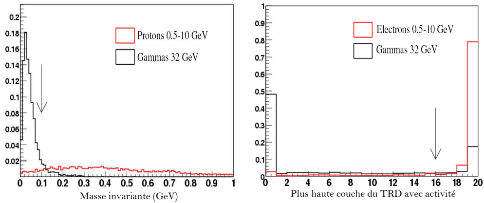
FIG. 11.15 – Coupures de sélections pour le mode conversion : masse invariante des traces à gauche et activité dans le TRD à droite [264].
