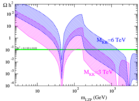
FIG. 3.6 – Contraintes cosmologiques sur les modèles à dimensions supplémentaires : UED à gauche [83] et Randall-Sundrum SO(10) à droite [68].
