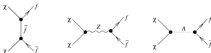
FIG. 8.3 – Diagrammes contribuant à l'annihilation de neutralinos en f\bar{f} dans le MSSM.
