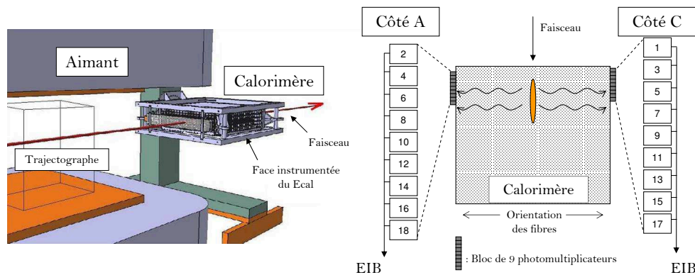
FIG. 6.6 – Positions relatives du calorimètre et des plans de Silicium (à gauche, [183]) et numérotation des photomultiplicateurs (à droite).
