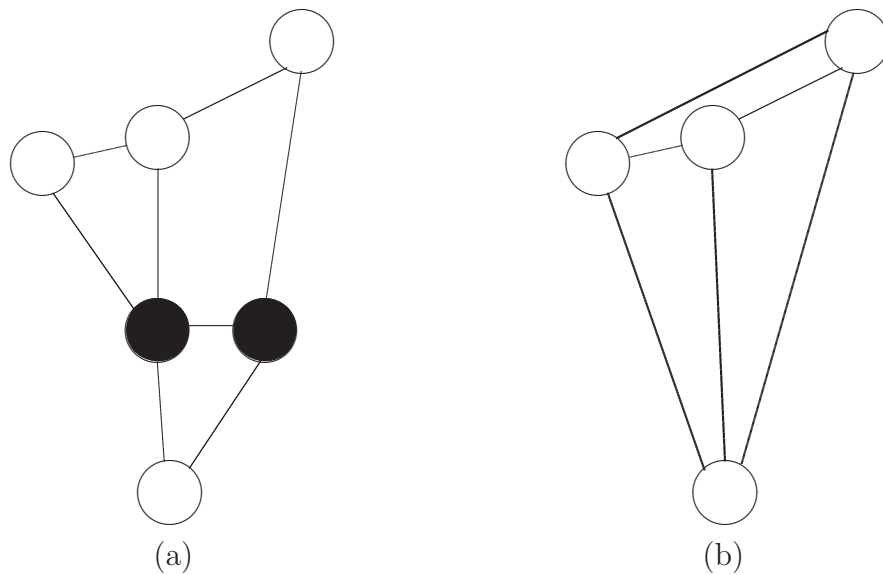
FIG. 1.4 – Marginalisation dans un graphe non orienté : (a) Exemple d'un graphe non orienté (b) Marginalisation du graphe (a) par rapport aux variables en noir
